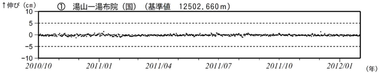
図2※ 鶴見岳・伽藍岳 GPS連続観測による基線長変化（2010年10月～2012年1月）
