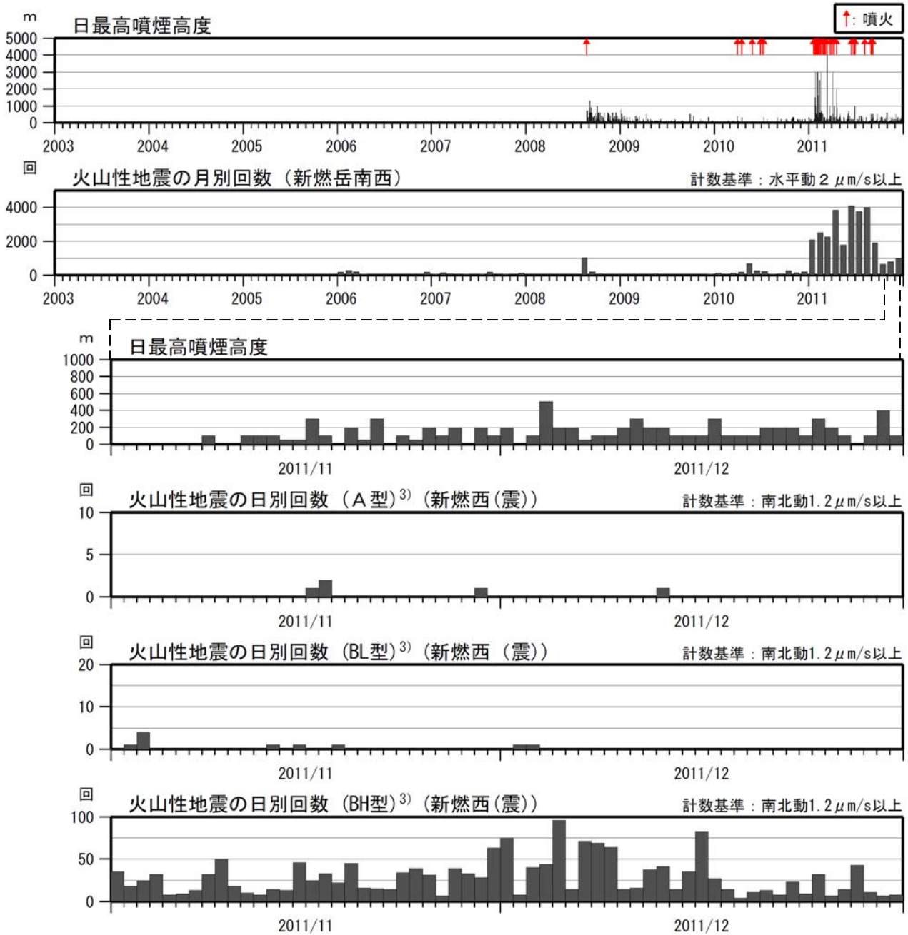
図 2※ 霧島山（新燃岳） 火山活動経過図（2003 年 1 月～2011 年 12 月）
