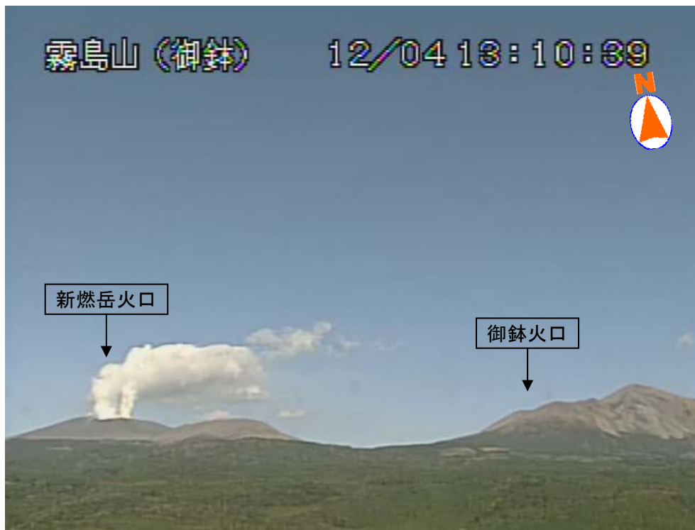
図 9 霧島山（御鉢） 遠望カメラによる御鉢の状況（12 月 4 日、猪子石遠望カメラより） 火口縁を超える噴煙は認められませんでした。
