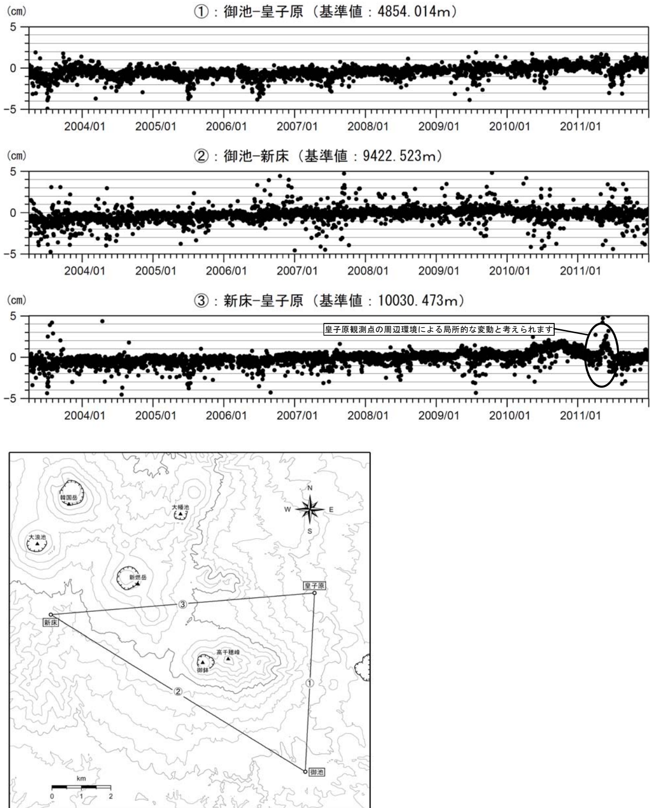
図 11 霧島山（御鉢） GPS 連続観測による基線長変化（2003 年 4 月～2011 年 12 月） <12 月の状況>
