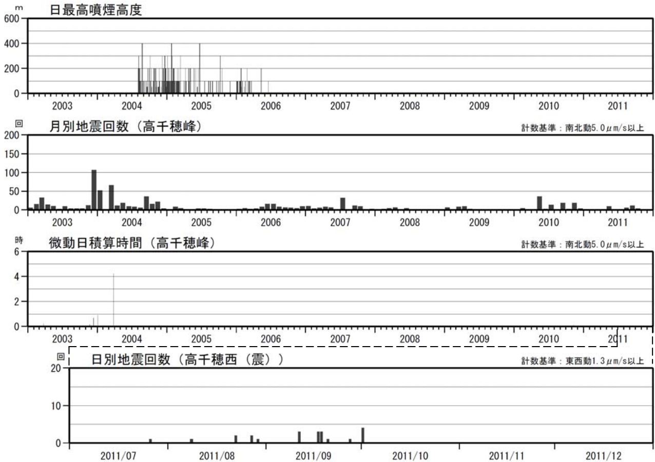
図 10※ 霧島山（御鉢） 火山活動経過図（2003 年 1 月～2011 年 12 月）
