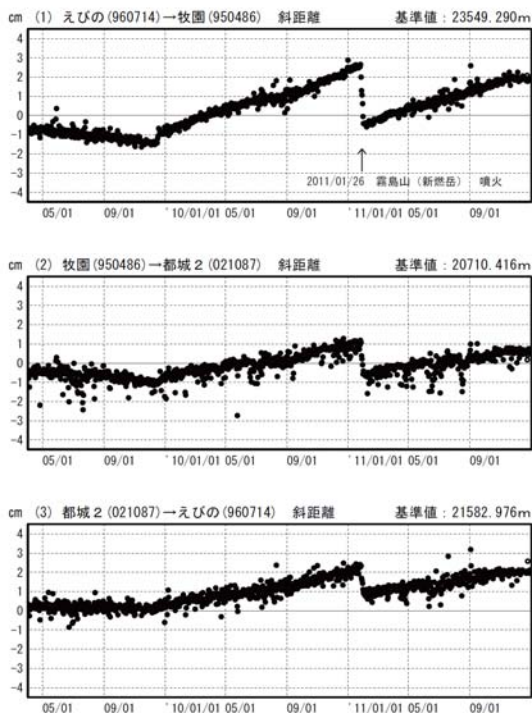
図7※ 霧島山（新燃岳） 国土地理院によるGPS観測結果*（2009年4月～2011年12月） 国土地理院のGPSによる地殻変動観測では、新燃岳の北西数kmの地下深くのマグマだまりへのマグマの供給を示す変化が続いています。なお、GPSの一部の基線ではこれまで見られていた伸びの傾向がやや鈍化しています。
