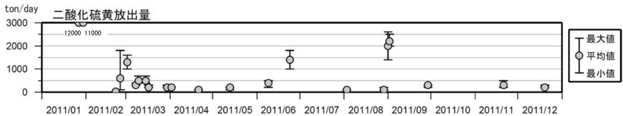
図 4 霧島山（新燃岳） 火山ガスの状況（2011 年 1 月～12 月）
