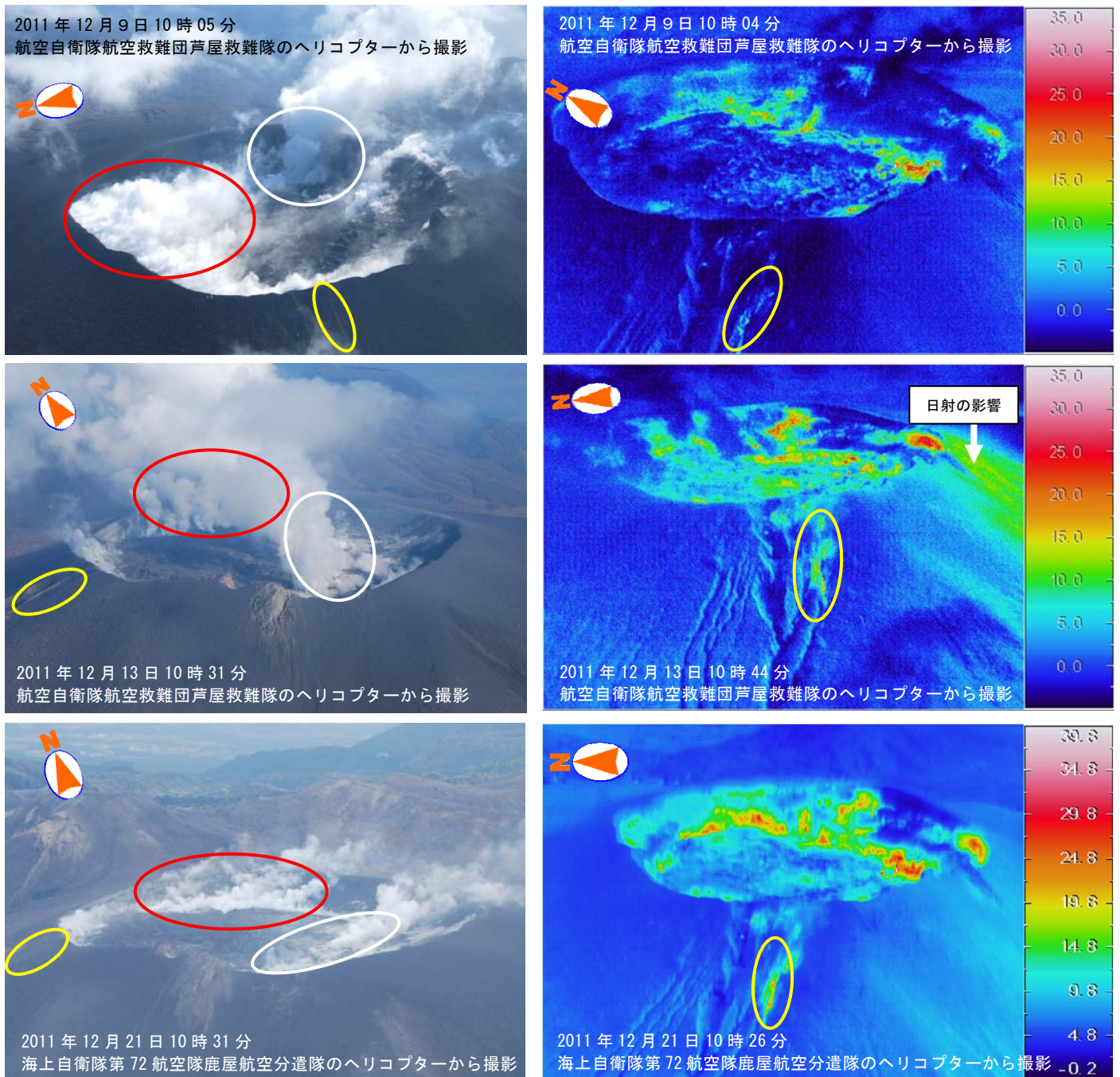
図5 霧島山（新燃岳） 火口付近の状況（左図） 赤外熱映像装置による火口付近の地表面温度分布（右図）
