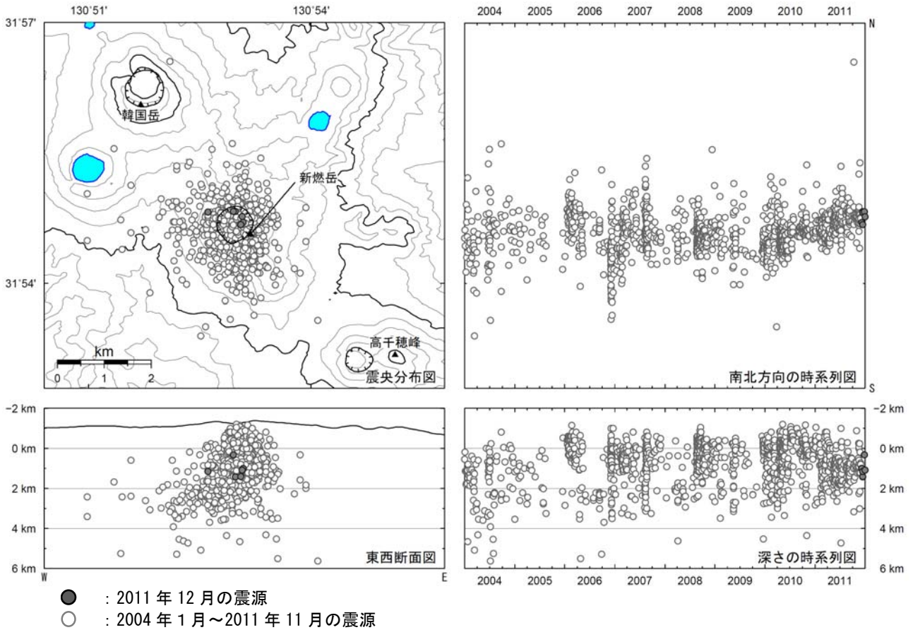
図 3※ 霧島山（新燃岳） 震源分布図（2004 年 1 月～2011 年 12 月）
