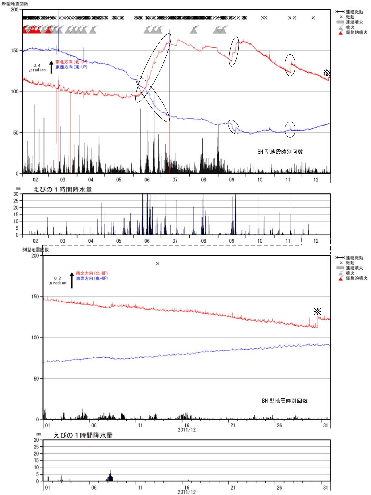
図 6 霧島山（新燃岳） BH 型地震の時間別回数と高千穂河原傾斜計の変化（2011 年 2 月～12 月）
