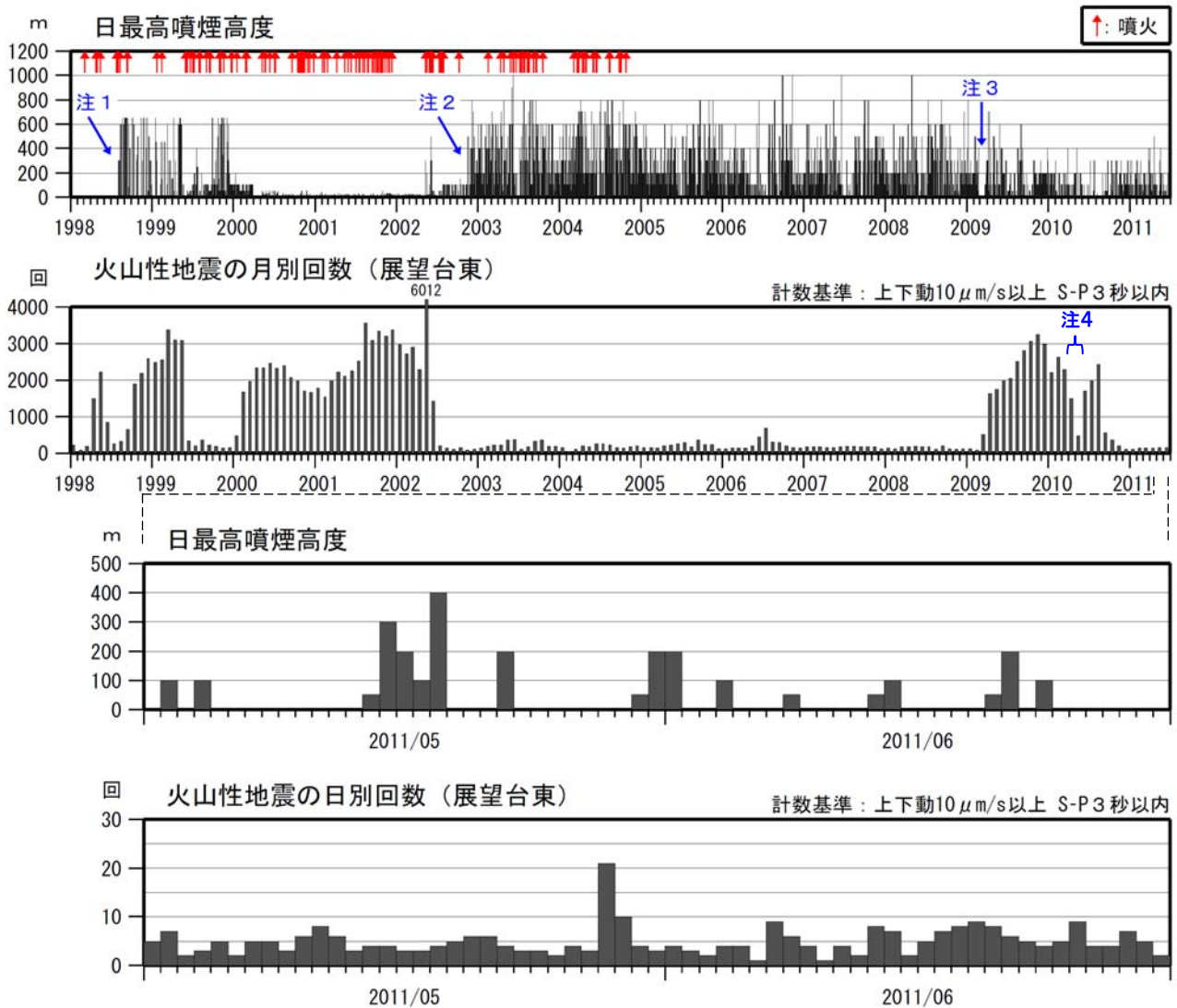
図 2 薩摩硫黄島 火山活動経過図（1998 年 1 月～2011 年 6 月）
