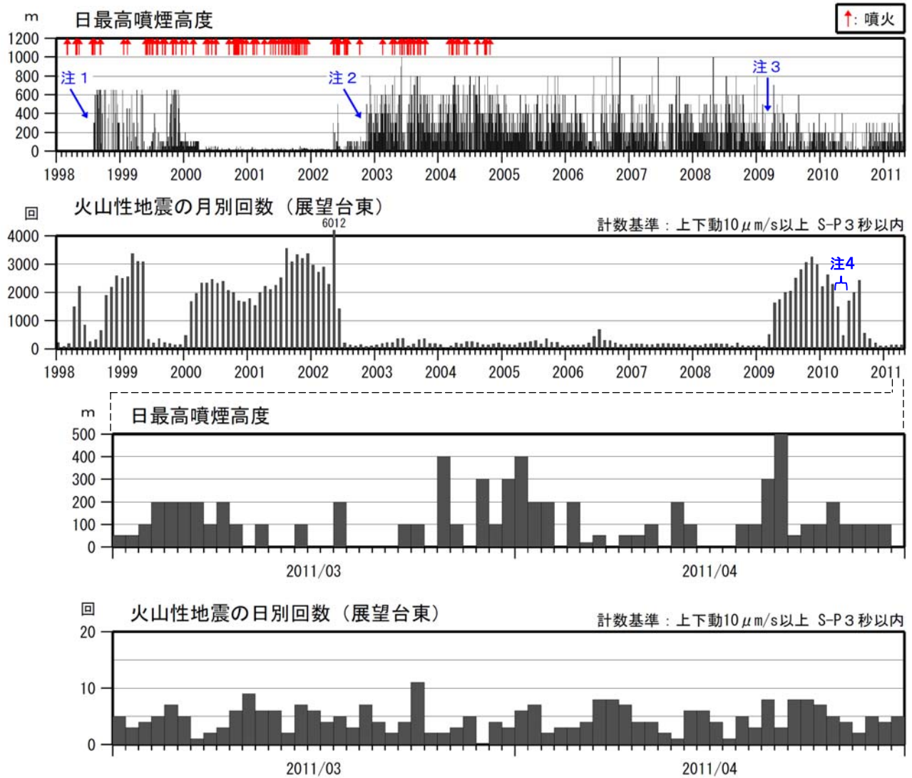
図2 薩摩硫黄島 火山活動経過図（1998年1月～2011年4月）
