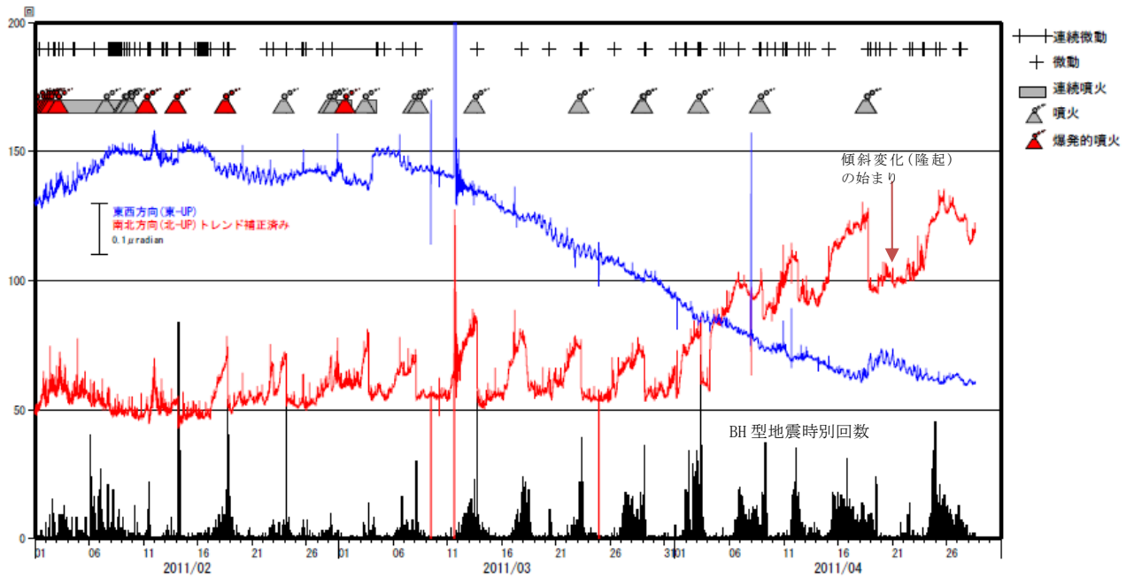
図3 霧島山（新燃岳）BH型地震 2) の時間別回数と高千穂河原傾斜計の変化 (2011年2月1日～4月28日) 4月22日05時頃(↓)から新燃岳側のわずかな隆起が認められていましたが、27日からゆるやかに沈降しています。
