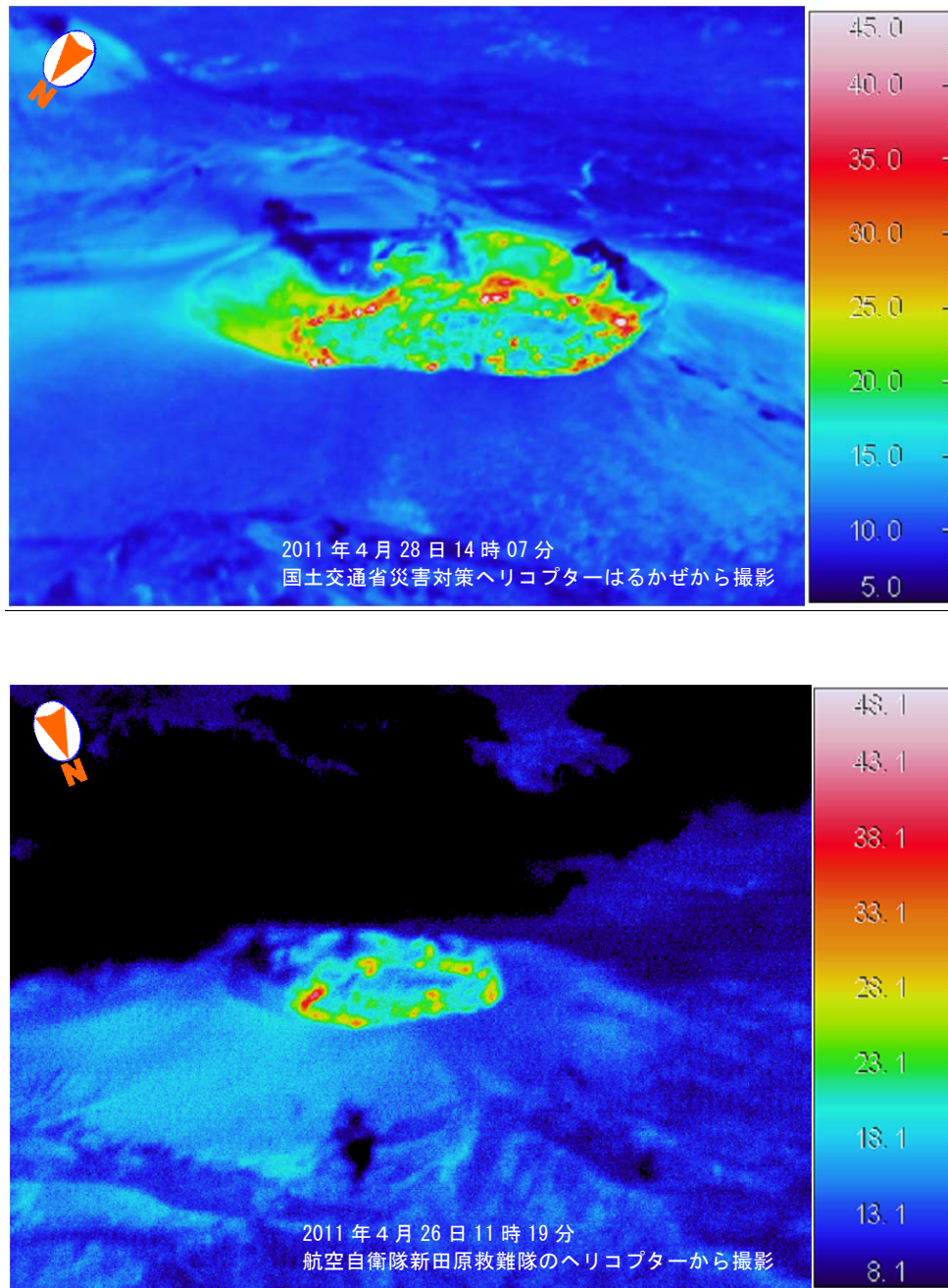
図 2 霧島山（新燃岳） 赤外熱映像装置による火口付近の地表面温度分布
