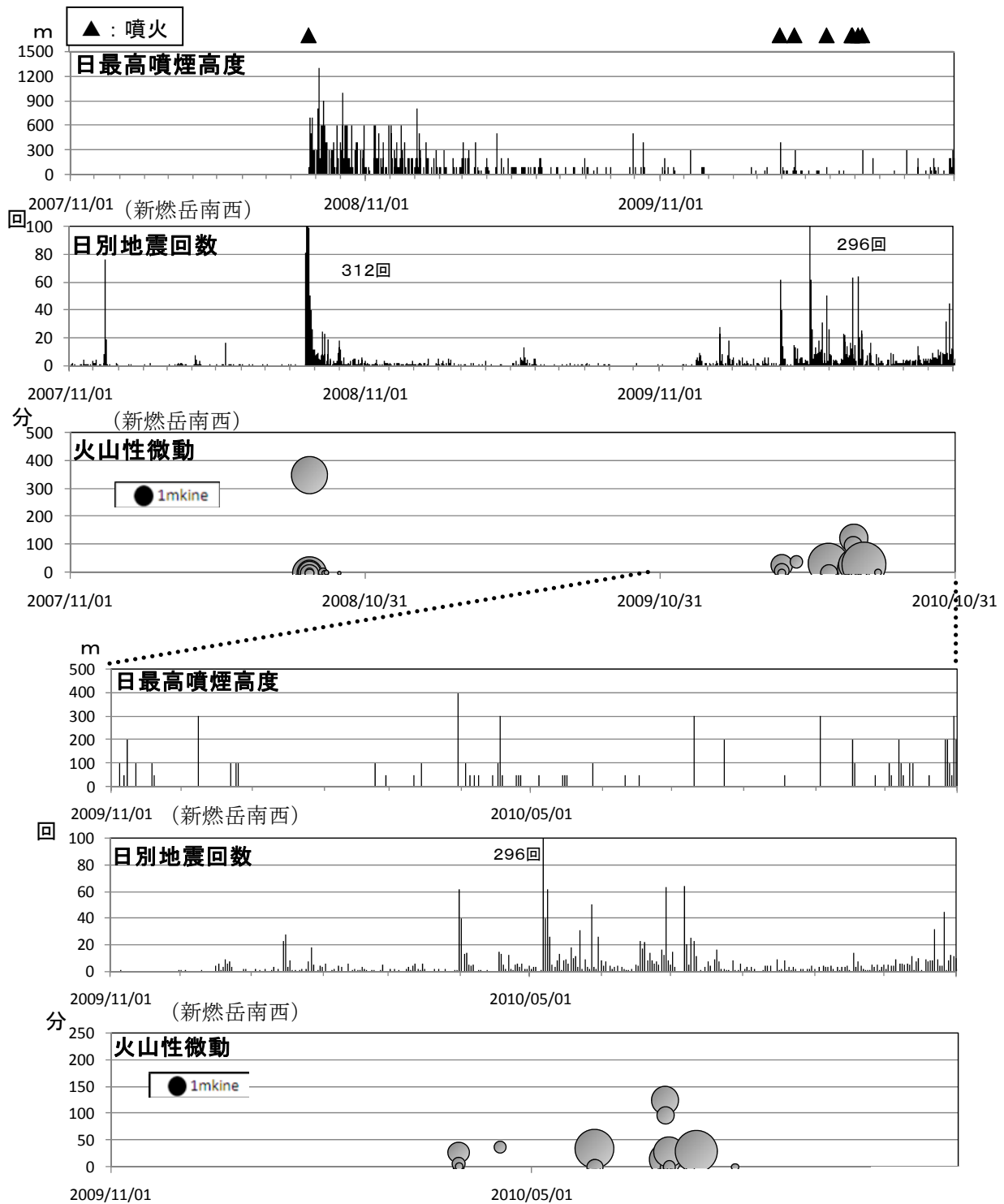
図2 霧島山（新燃岳） 火山活動経過図（2007年11月～2010年10月）
