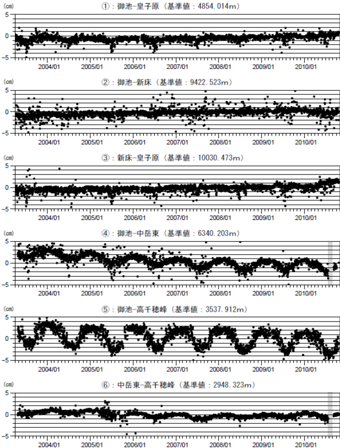
図7 霧島山（御鉢） GPS 連続観測による基線長変化（2003 年 4 月～2010 年 10 月） <10 月の状況>
