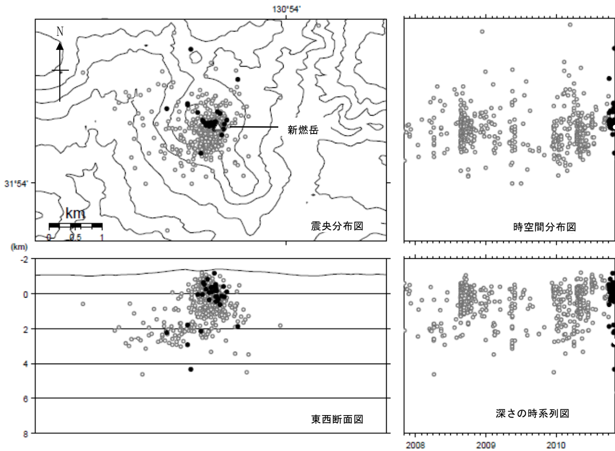
図 3※ 霧島山（新燃岳） 震源分布図（2007 年 11 月～2010 年 10 月）
