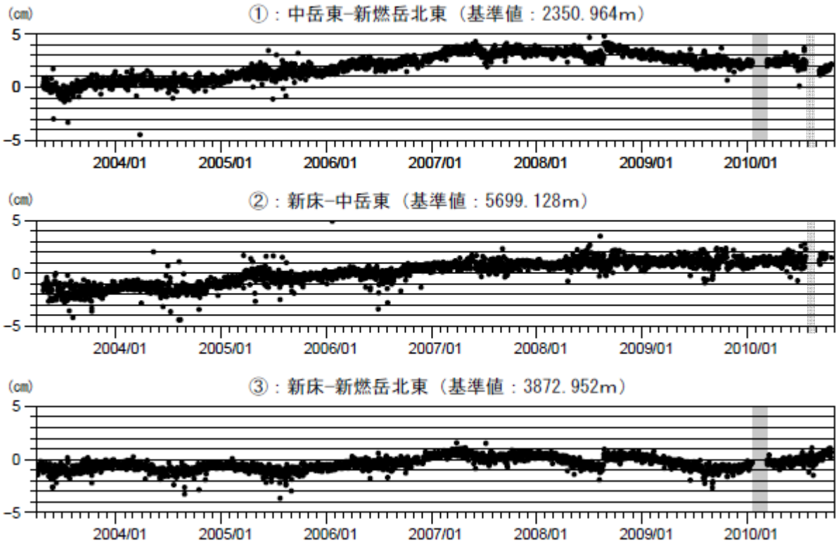
図 4 霧島山（新燃岳） GPS 連続観測による基線長変化（2003 年 4 月～2010 年 10 月） 火山活動によると考えられる変化は認められませんでした。
