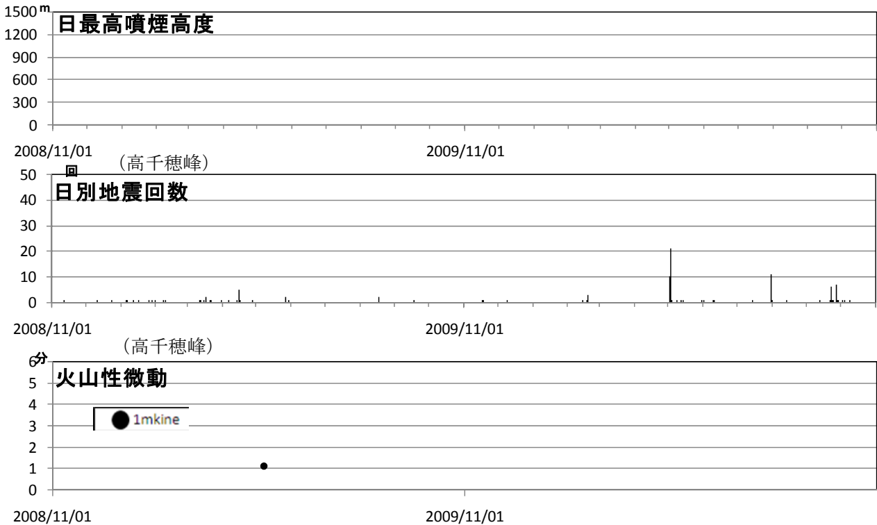
図 6 霧島山（御鉢） 火山活動経過図（2008 年 11 月～2010 年 10 月）
