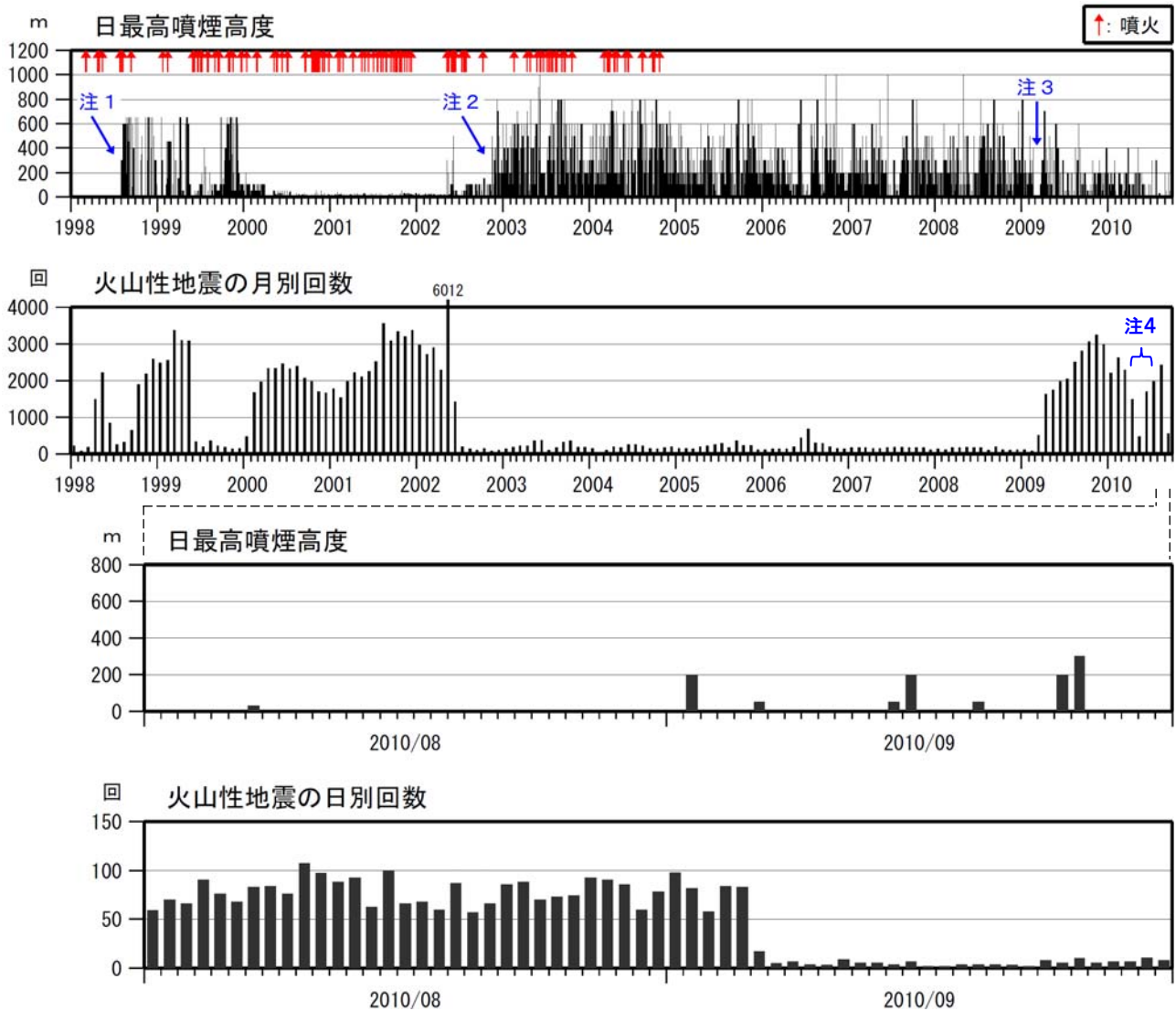
図2 薩摩硫黄島 火山活動経過図（1998年1月～2010年9月）
