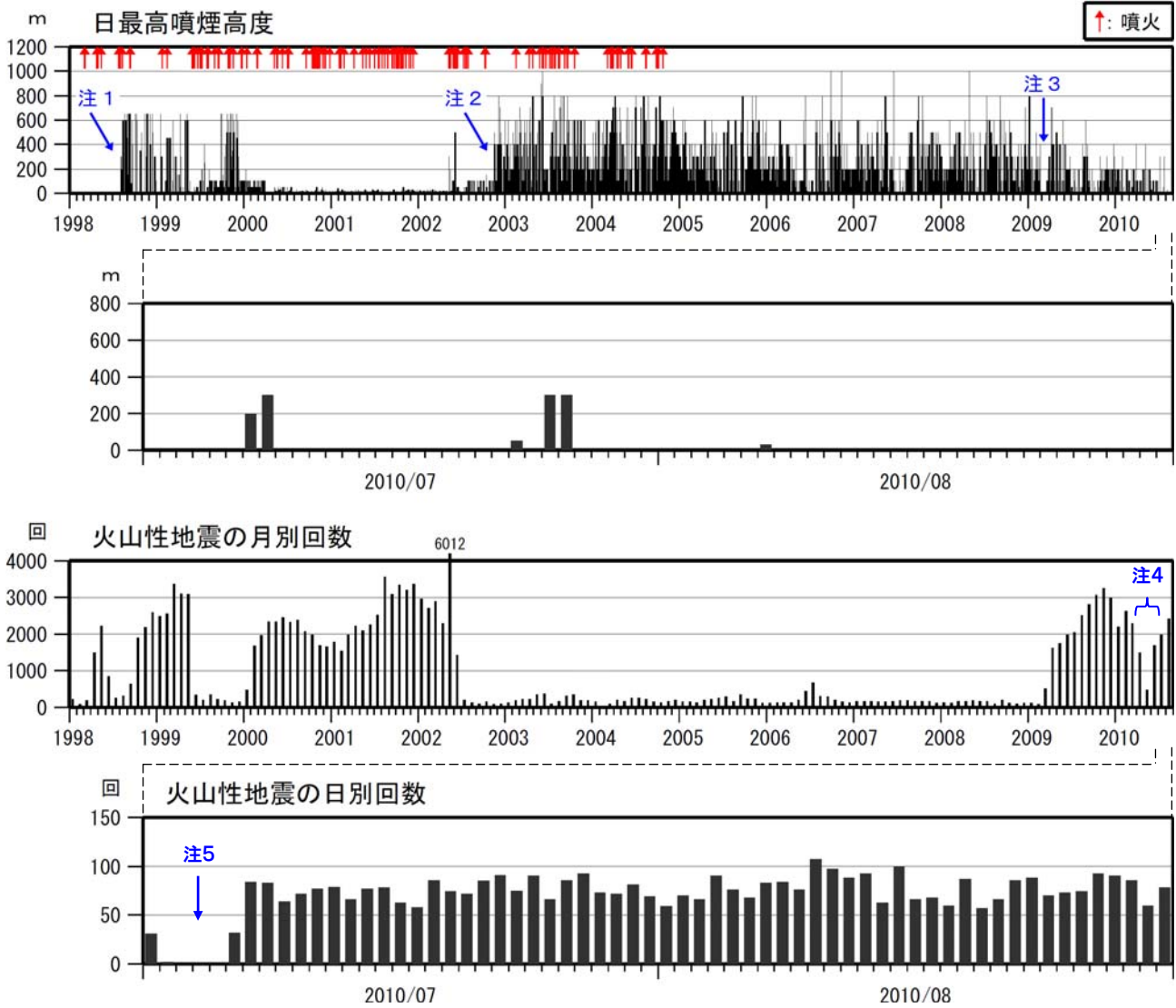
図2 薩摩硫黄島 火山活動経過図（1998年1月～2010年8月）
