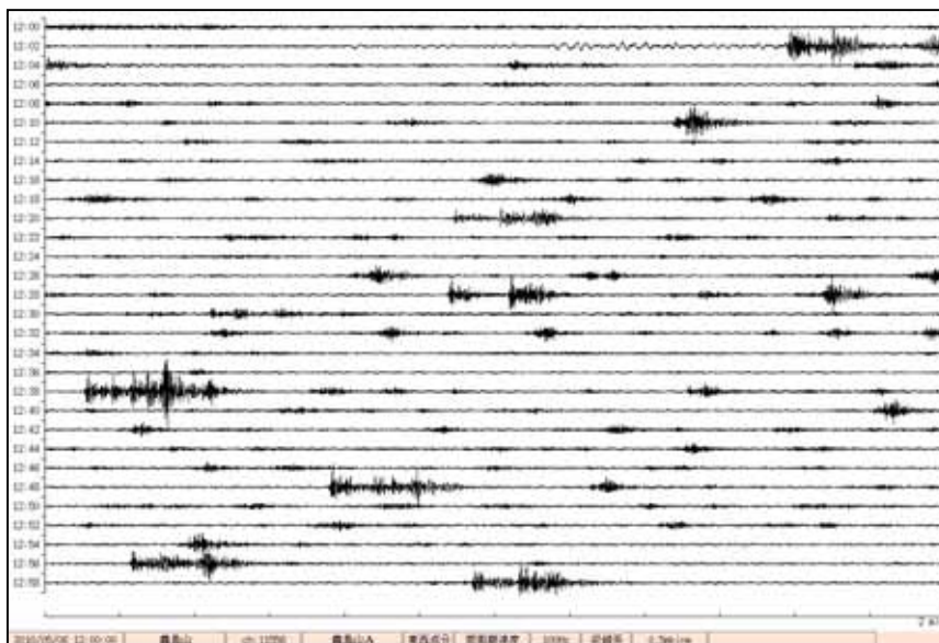
図 1 霧島山（新燃岳）火山性地震の状況（2010 年 5 月 6 日 12 時～13 時）
