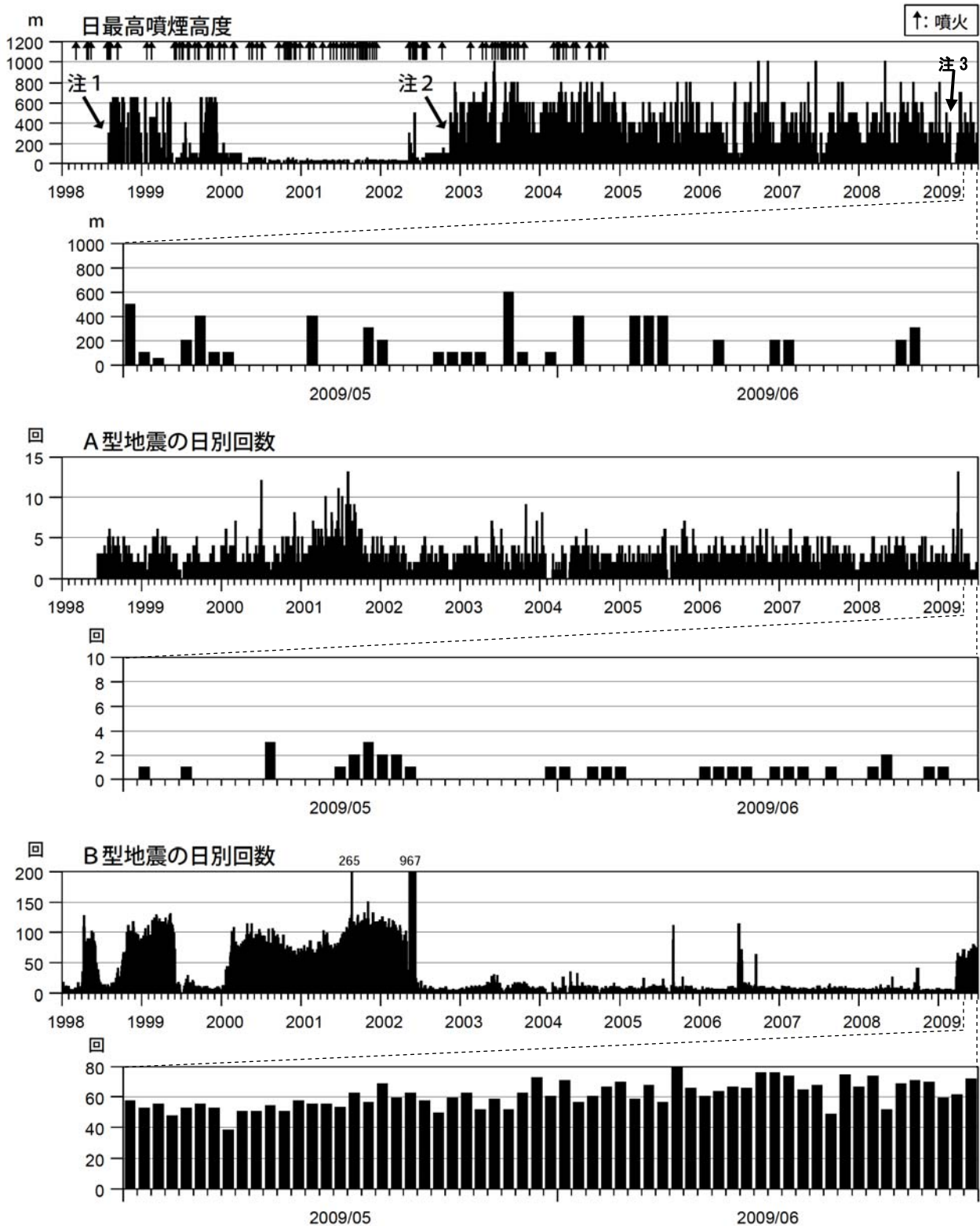
図2 薩摩硫黄島 火山活動経過図（1998年1月～2009年6月）
