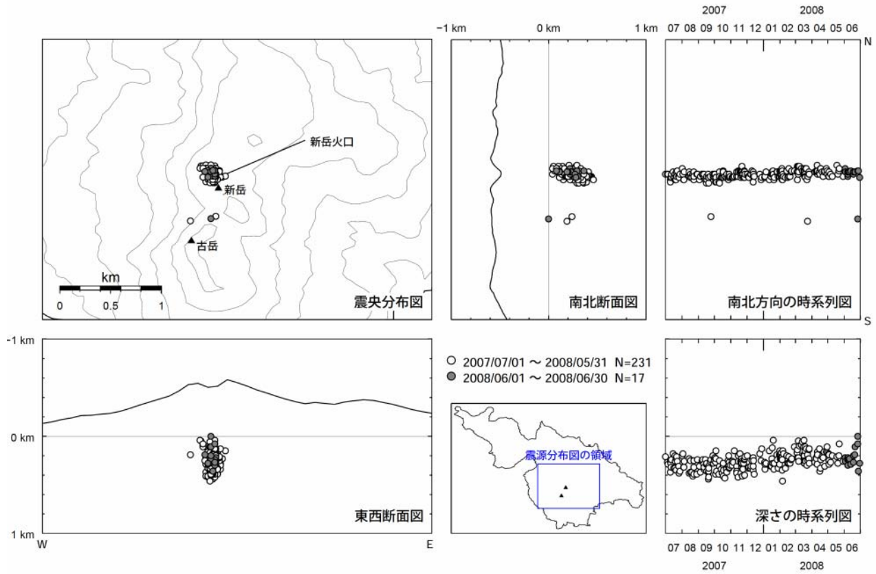
図3 口永良部島 震源分布図(2007年7月~2008年6月)
