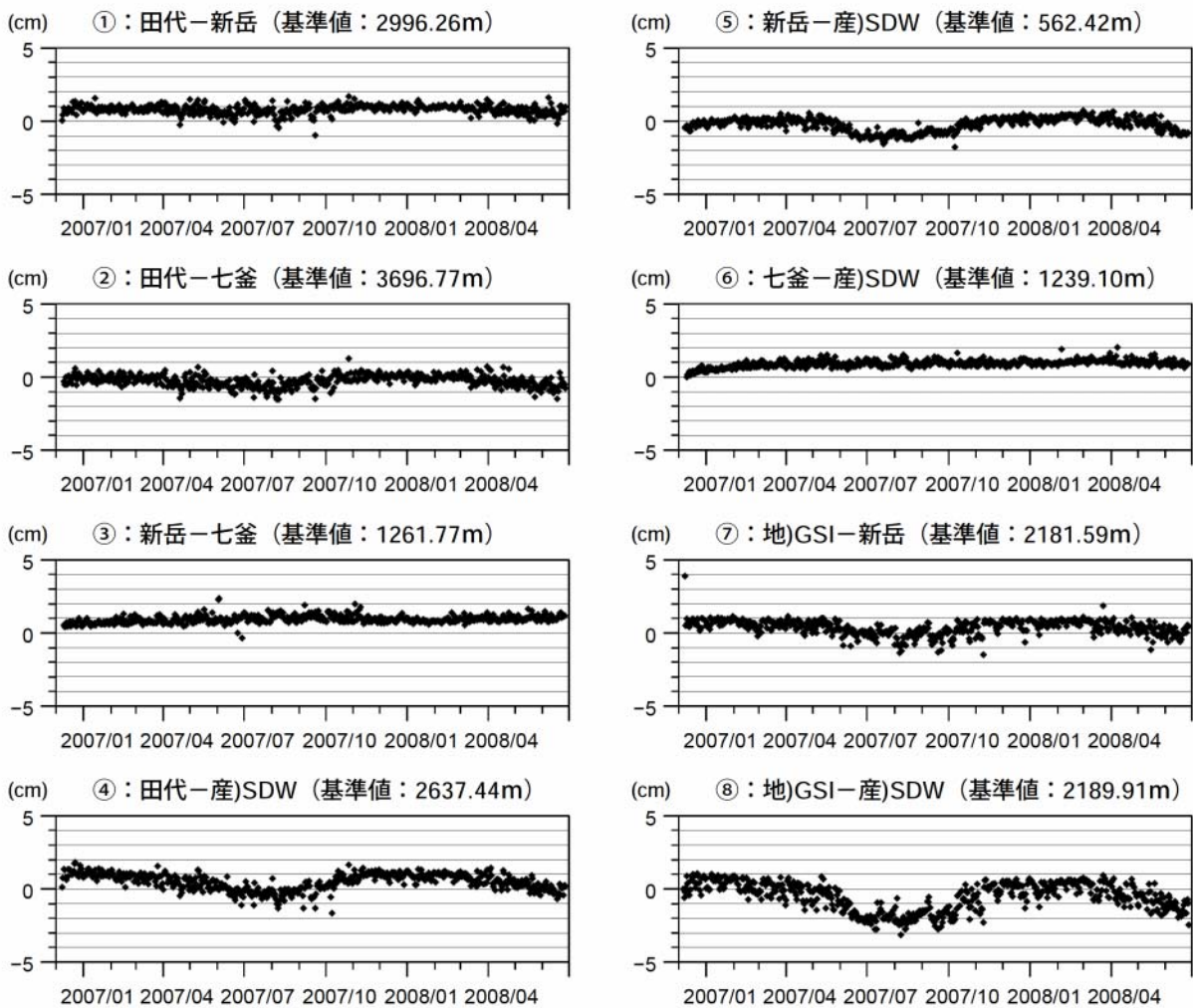
図5 口永良部島 GPS 連続観測による基線長変化(2006年12月8日~2008年6月30日)
