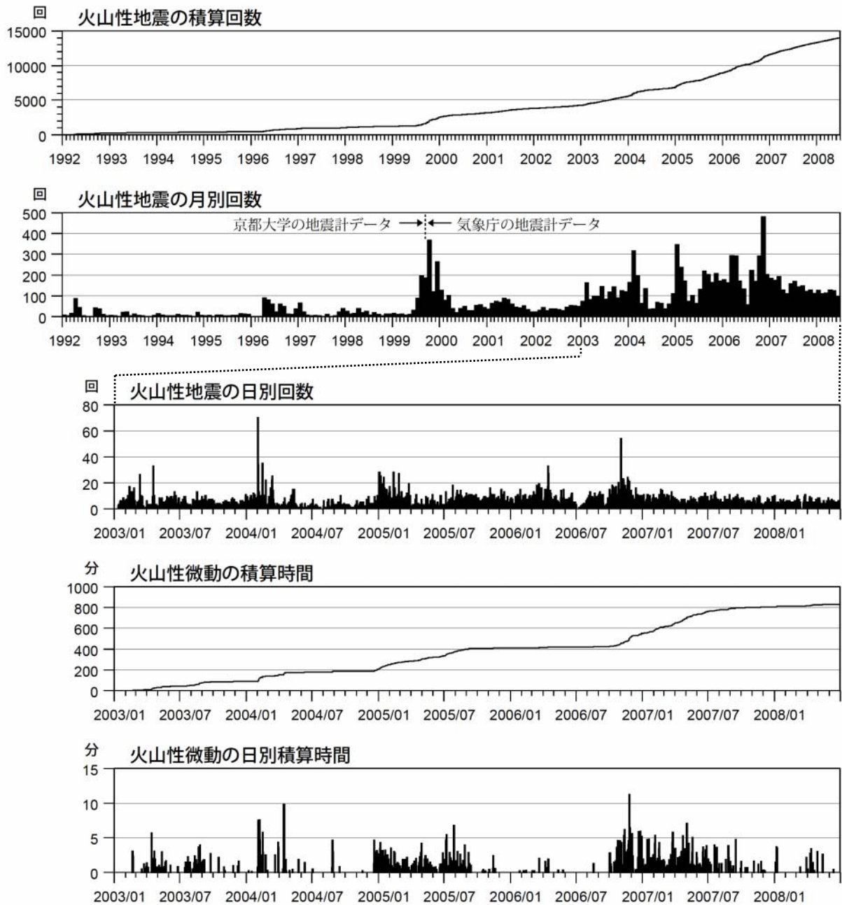
図2 口永良部島 火山性地震・微動活動経過図(1992年1月～2008年6月) ・火山性地震及び火山性微動は少ない状態で経過しています。
