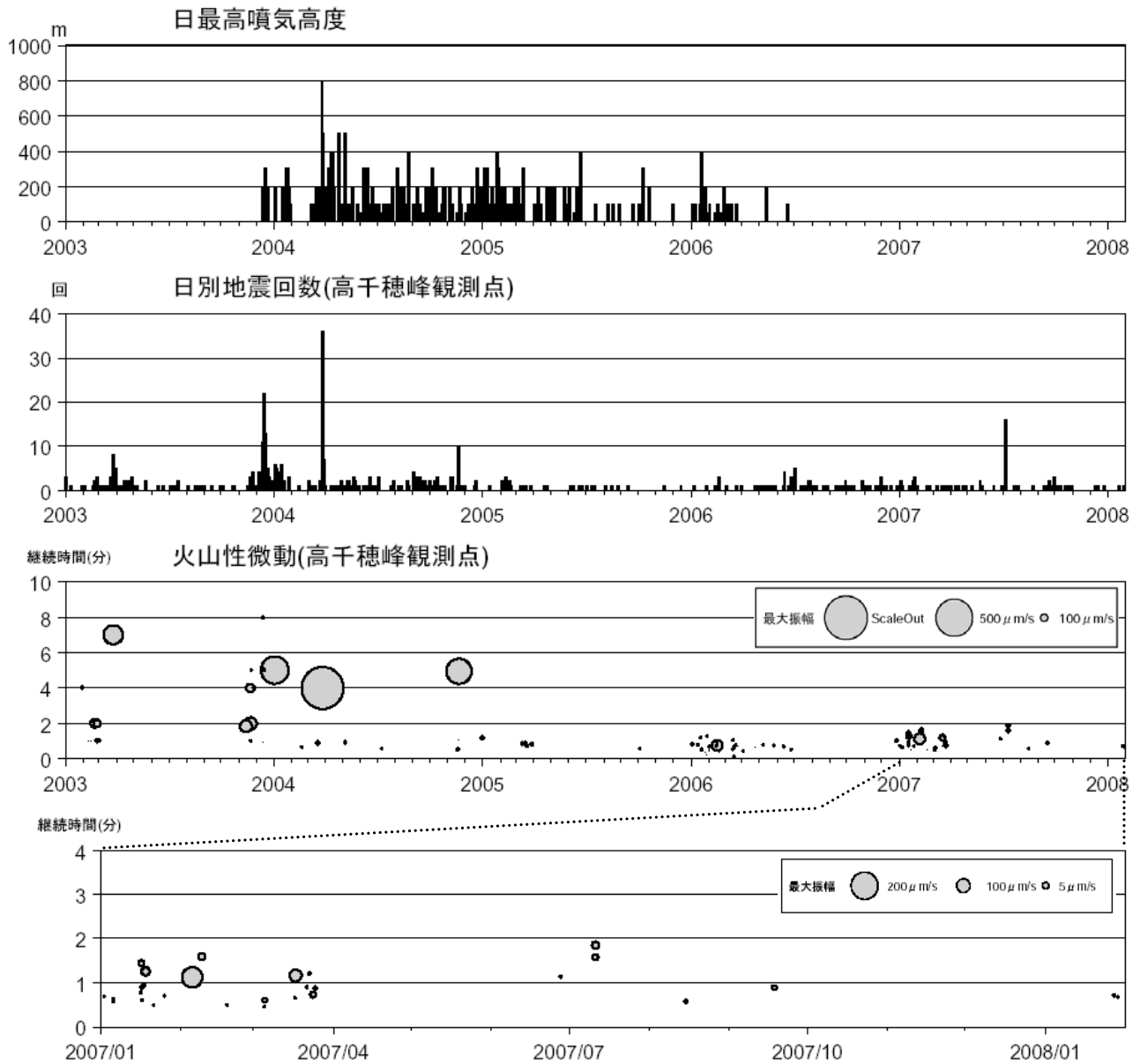
図 6 霧島山(御鉢) 火山活動経過図(2003 年 1 月～2008 年 1 月)
