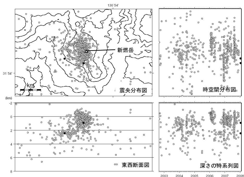
図 3※ 霧島山(新燃岳) 震源分布図(2002 年 9 月～2008 年 1 月)
