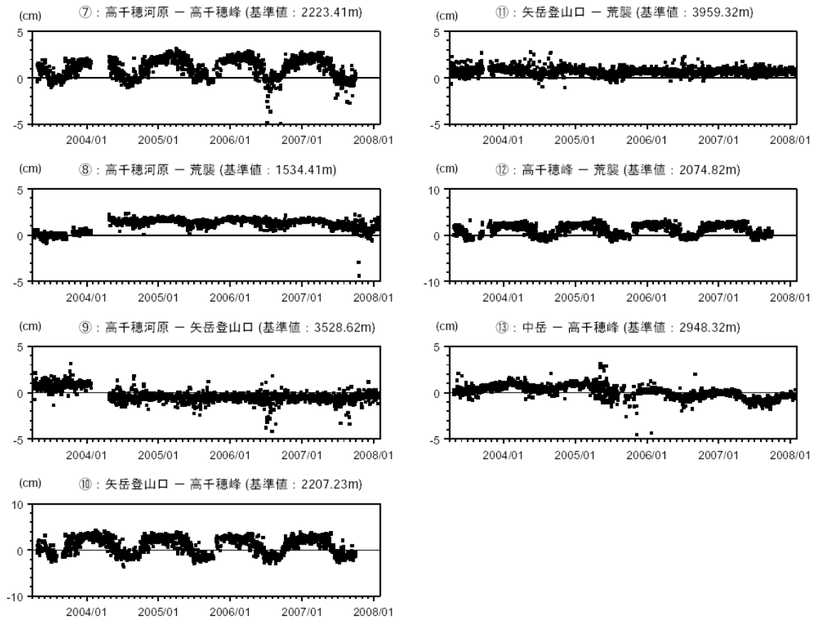
図 10 霧島山（御鉢） GPS 連続観測による基線長変化（2003 年 4 月～2008 年 1 月） 各基線長には火山活動に起因するとみられる変化はありませんでした。
