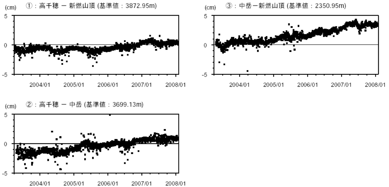
図4 霧島山(新燃岳) GPS 連続観測による基線長変化 (2003 年 4 月～2008 年 1 月) 長期的には新燃岳の山体膨張を示す観測結果が得られていますが、2007 年 4 月頃からは伸びがやや鈍化しています。
