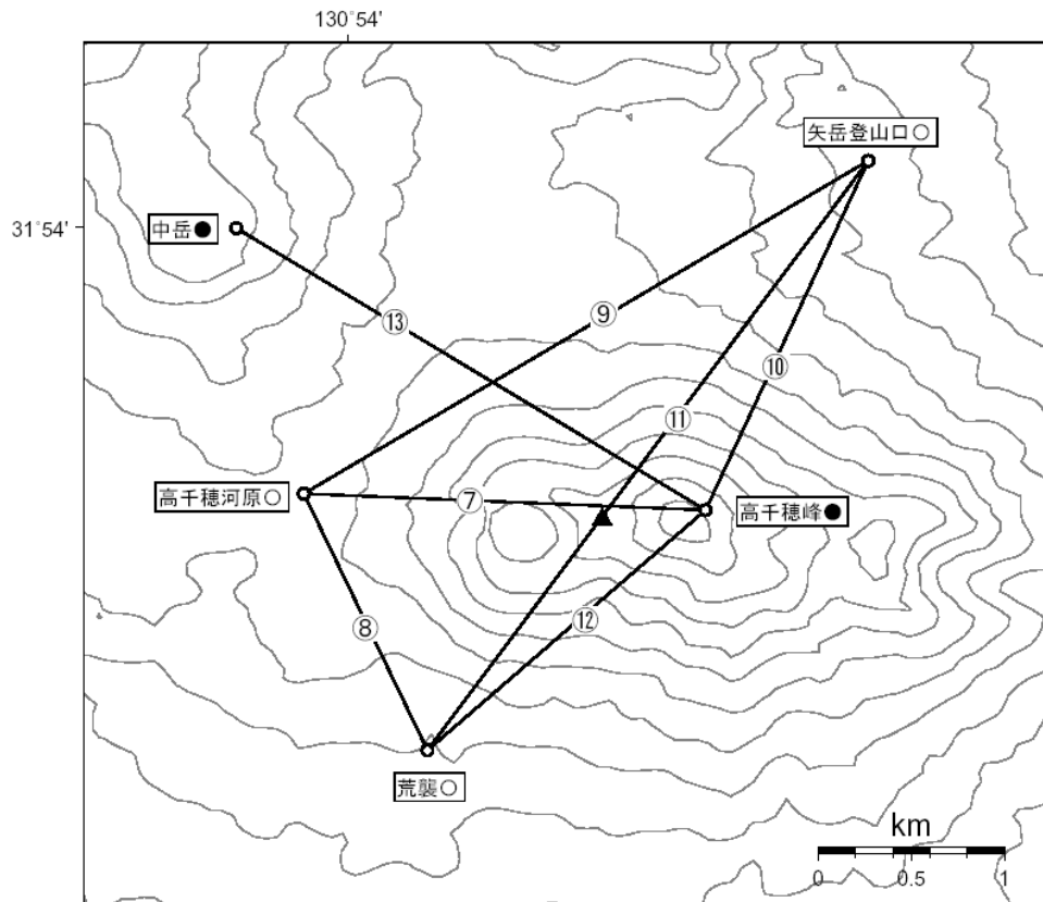
図 11 霧島山（御鉢） GPS 連続観測点と基線番号 この基線は図 10 の⑦～⑬に対応しています。
