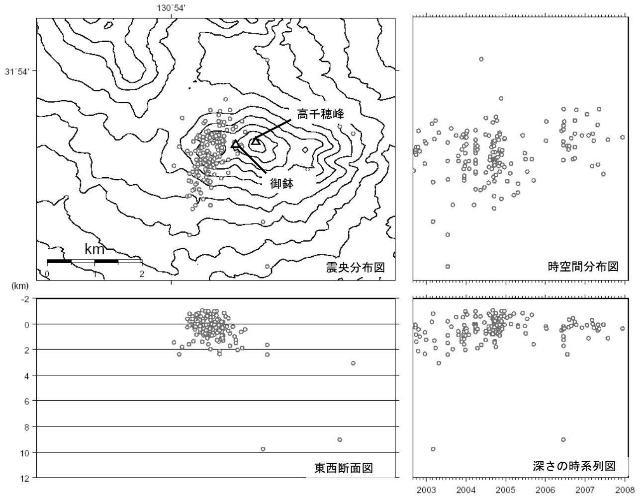
図 7※ 霧島山（御鉢） 震源分布図(2003 年 9 月～2008 年 1 月)
