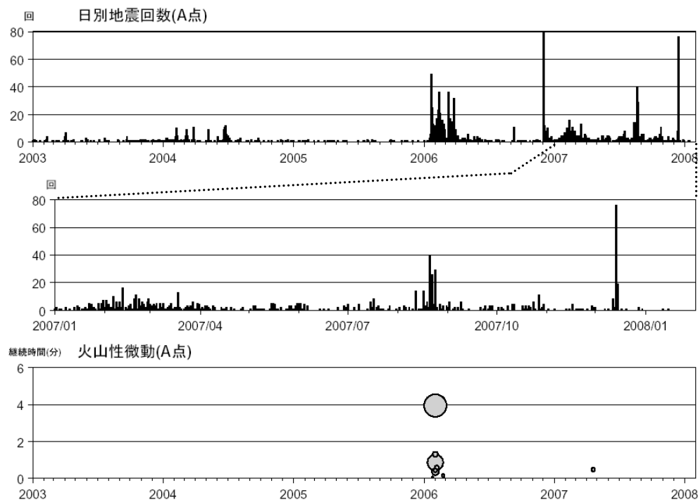
図 2 霧島山(新燃岳) 地震・微動活動経過図(2003 年 1 月～2008 年 1 月)
