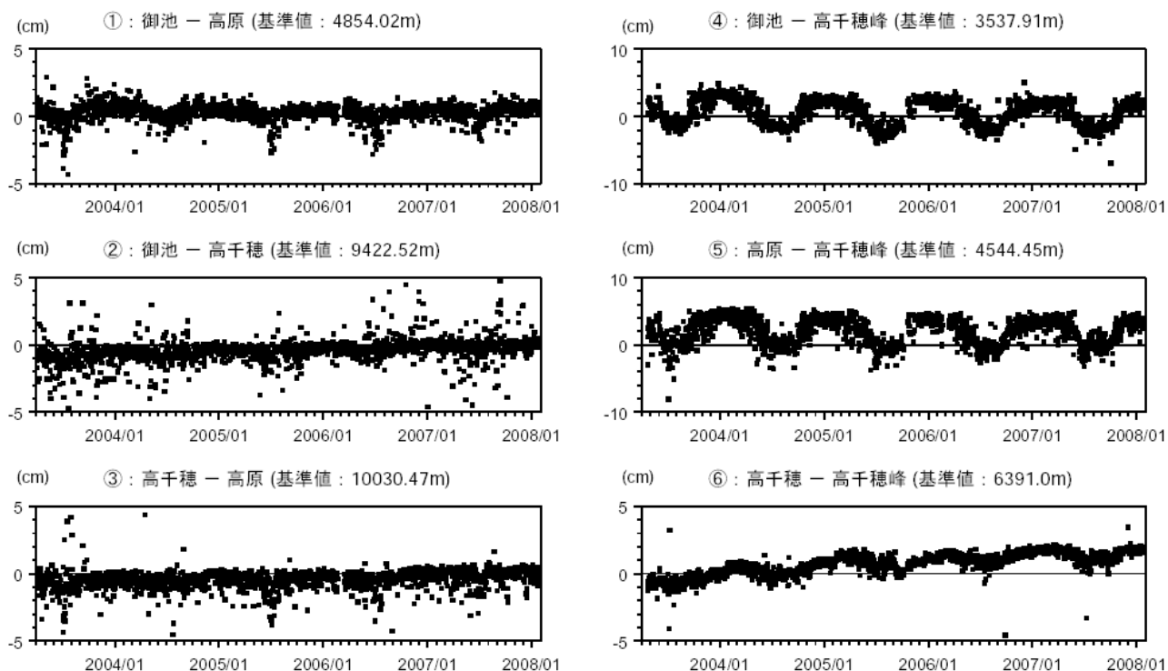
図 8 霧島山（御鉢） GPS 連続観測による基線長変化（2003 年 4 月～2008 年 1 月） 各基線長には火山活動に起因するとみられる変化はありませんでした。
