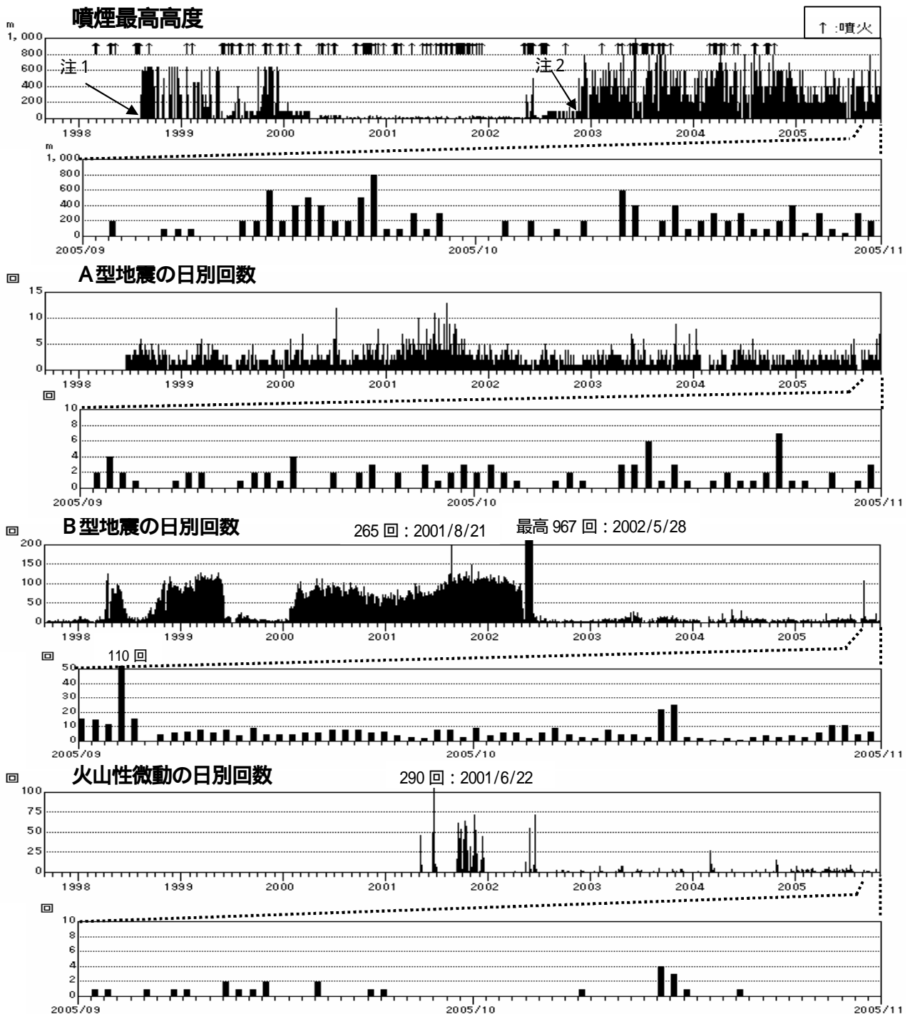
図2 火山活動経過図(1997年9月10日~2005年10月31日)
