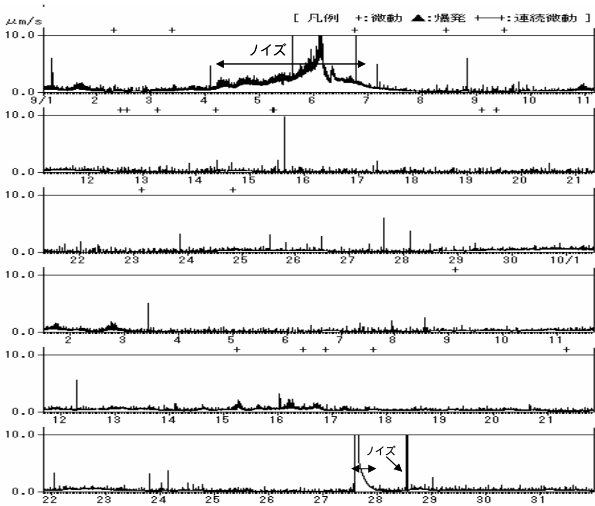
図3 1分間平均振幅の時間変化(地震計ST11点上下動成分(2005年9月1日~10月31日))
