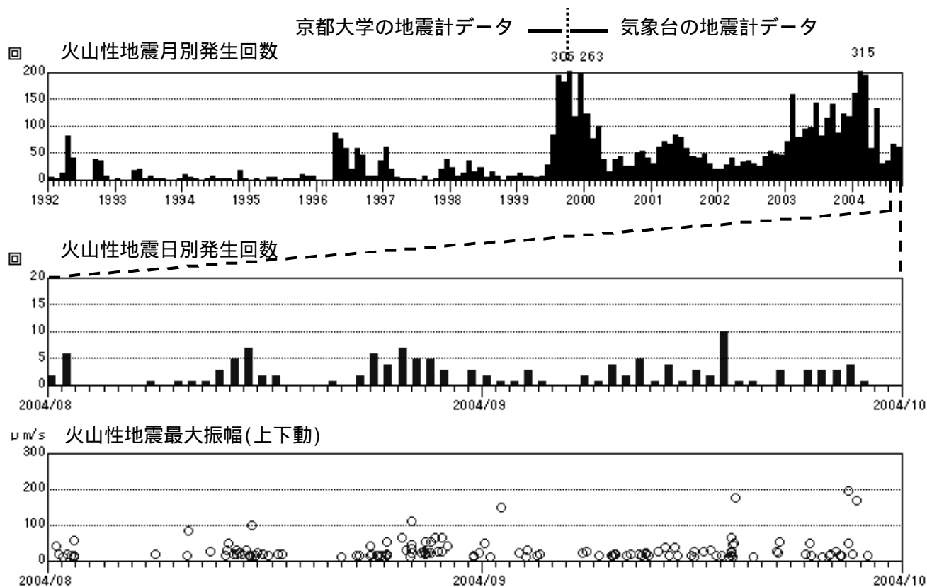
図1 火山性地震活動経過図(1992年1月1日~2004年9月30日) 1999年9月12日までは、京都大学のデータを利用。
