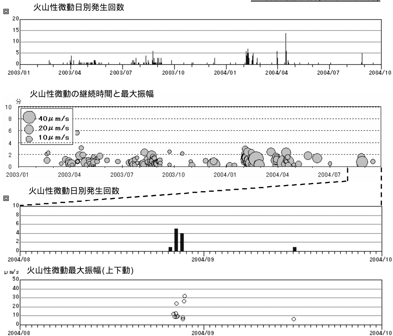
図2 火山性微動活動経過図(2003年1月1日~2004年9月30日)
