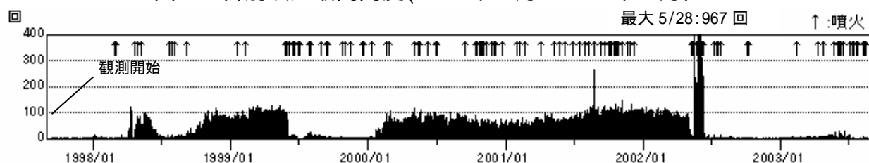
図2 火山性地震の日別回数(1997年9月～2003年8月)
