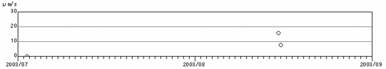
図 10 火山性微動の最大振幅(ST11 点上下動)(2003 年 7 月 1 日～ 8 月 31 日)
