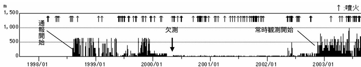
図1 日別噴煙最高高度(1998年8月～2003年8月)
