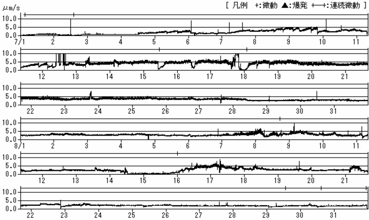
図 11 1 分間平均振幅の時間変化(ST11 点上下動)(2003 年 7 月 1 日～ 8 月 31 日)
