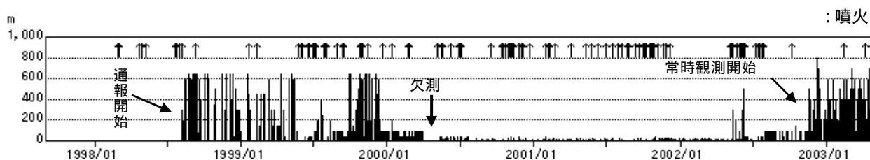
図 1 噴煙の日最高高度(1998 年 8 月～2003 年 4 月)
