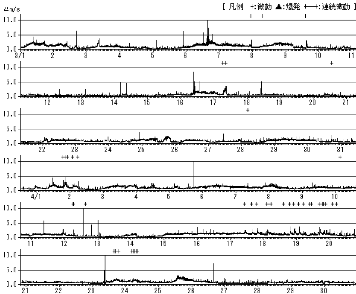
図 11 1 分間平均振幅の時間変化(上下動)(2003 年 3 月 1 日～ 4 月 30 日)
