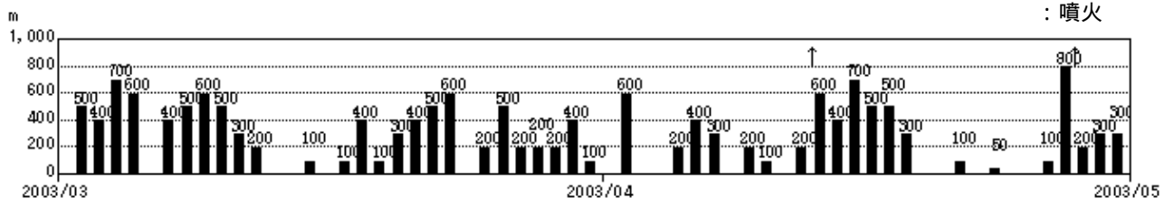
図4 噴煙の日最高高度(2003年3月1日~4月30日)
