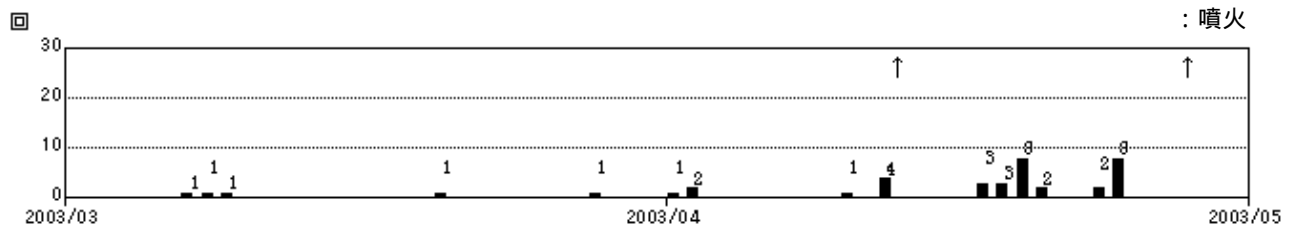
図9 火山性微動の発生回数(2003年3月1日~4月30日)
