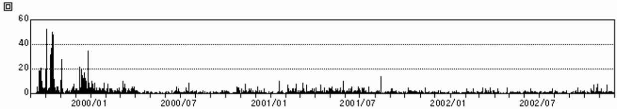
図1 A型地震日別地震回数(1999年9月12日～2002年11月30日)
