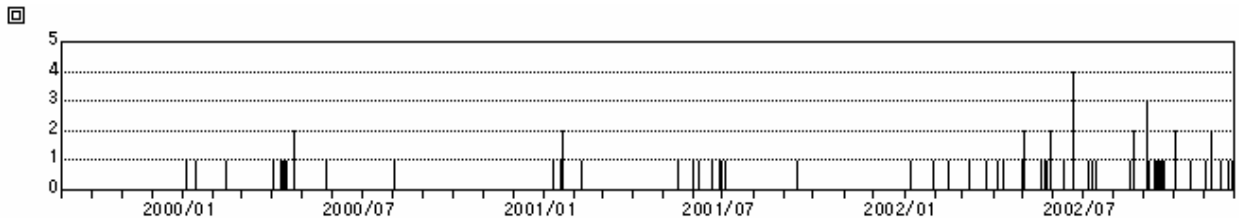
図2 B型地震日別地震回数(1999年9月12日～2002年11月30日)
