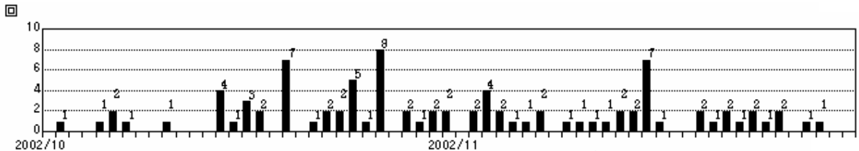
図3 A型地震日別地震回数(2002年10月1日～2002年11月30日)
