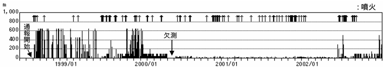
図 1 噴煙の日最高高度(1998 年 8 月～2002 年 11 月)
