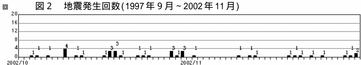
図 3 A 型地震の発生回数(2002 年 10 月 1 日～11 月 30 日)
