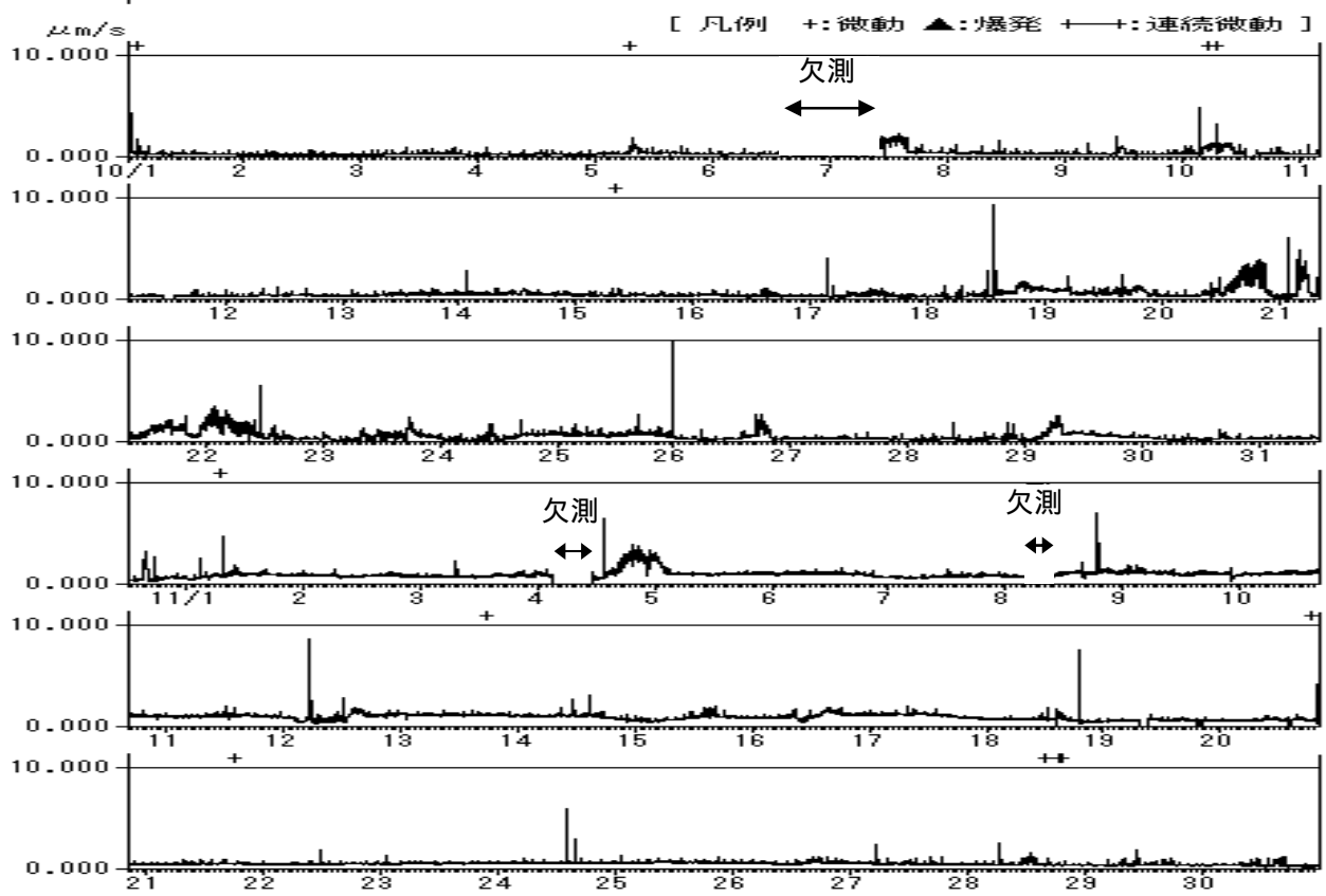
図7 1分間平均振幅の時間変化(上下動)(2002年10月1日~11月30日)
