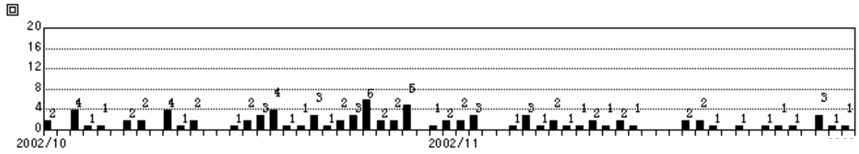
図5 B型地震の発生回数(2002年10月1日~11月30日)
