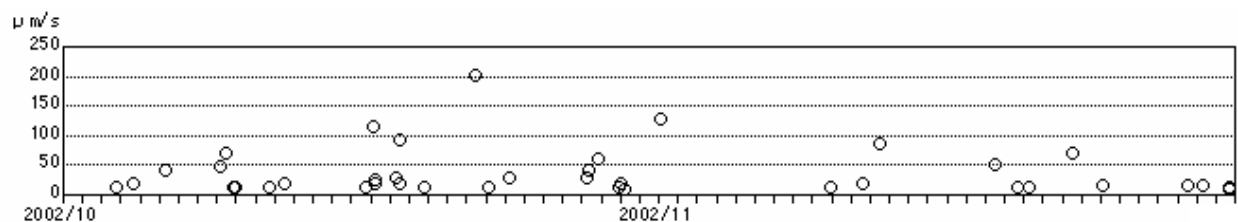
図 4 A 型地震の最大振幅分布(上下動)(2002 年 10 月 1 日～11 月 30 日)
