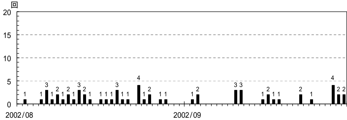
図3 A型地震の発生回数(2002年8月1日～9月30日)
