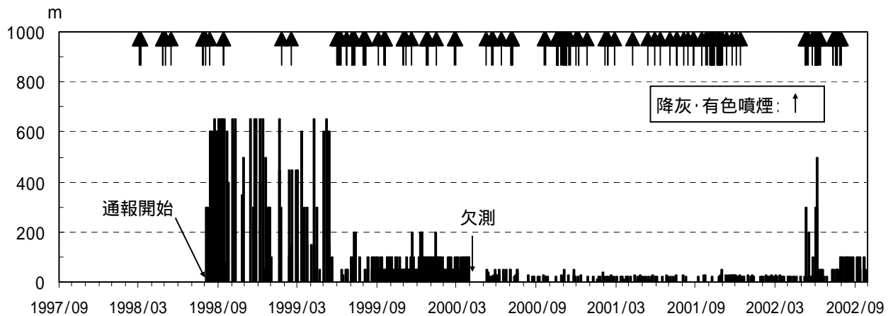
図 1 噴煙の日最高高度(1998 年 8 月 ~ 2002 年 9 月 : 三島村役場硫黄島出張所による)
