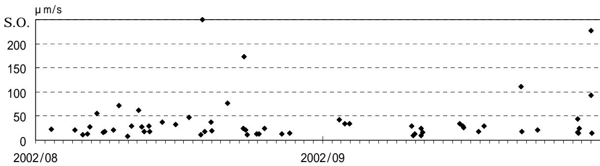
図4 A型地震の最大振幅分布(U-D成分)(2002年8月1日～9月30日)
