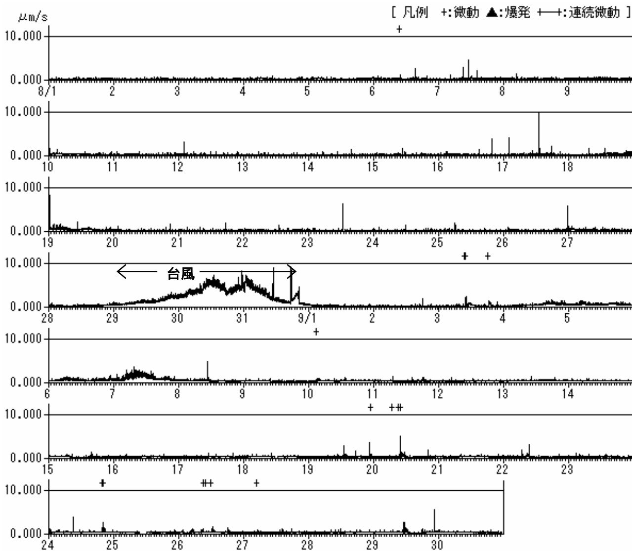
図7 1分間平均振幅の時間変化(U-D成分)(2002年8月1日～9月30日)
