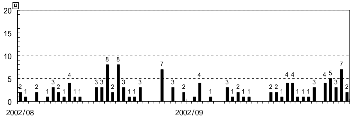
図5 B型地震の発生回数(2002年8月1日～9月30日)
