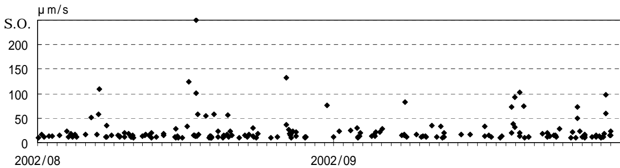
図6 B型地震の最大振幅分布(U-D成分)(2002年8月1日～9月30日)
