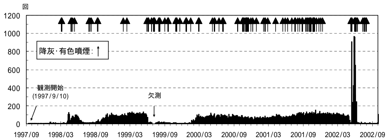
図 2 地震発生回数(1997 年 9 月 ~ 2002 年 9 月)
