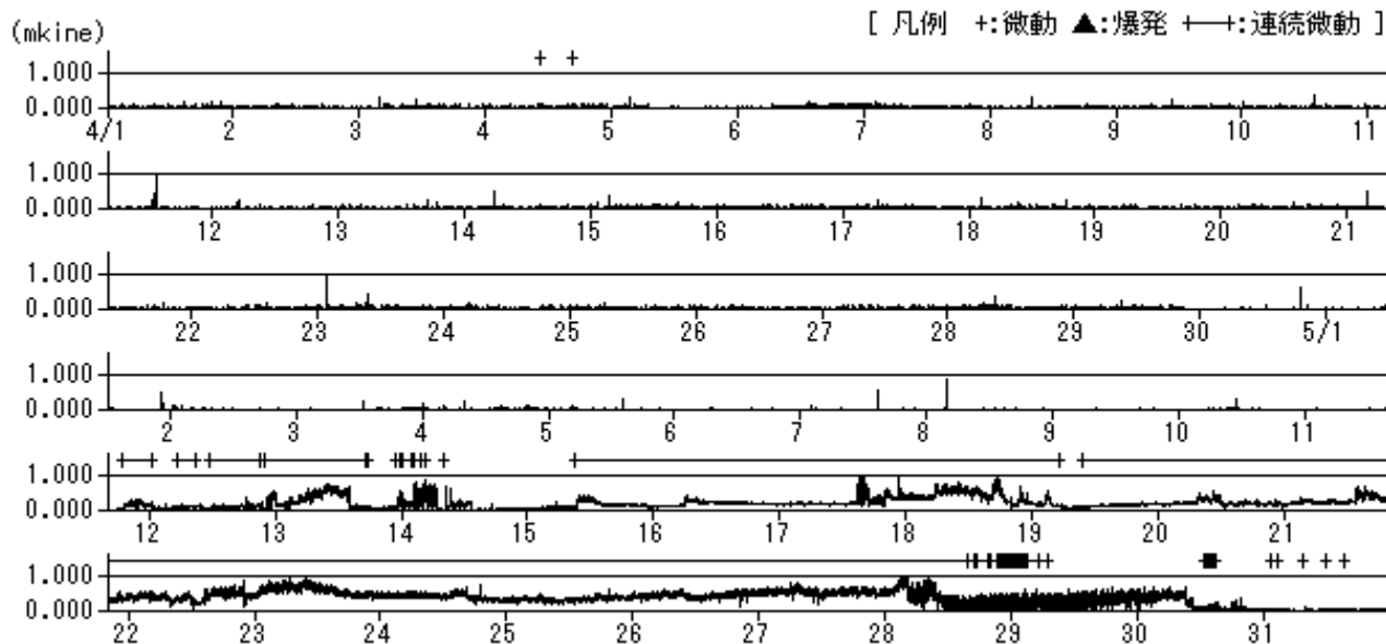
図6 1分間平均振幅(U-D成分)の時間変化(2002年4月~5月)
