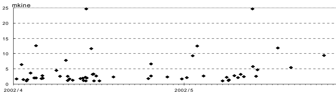
図3 A型地震の最大振幅(U-D成分)分布(2002年4月~5月)
