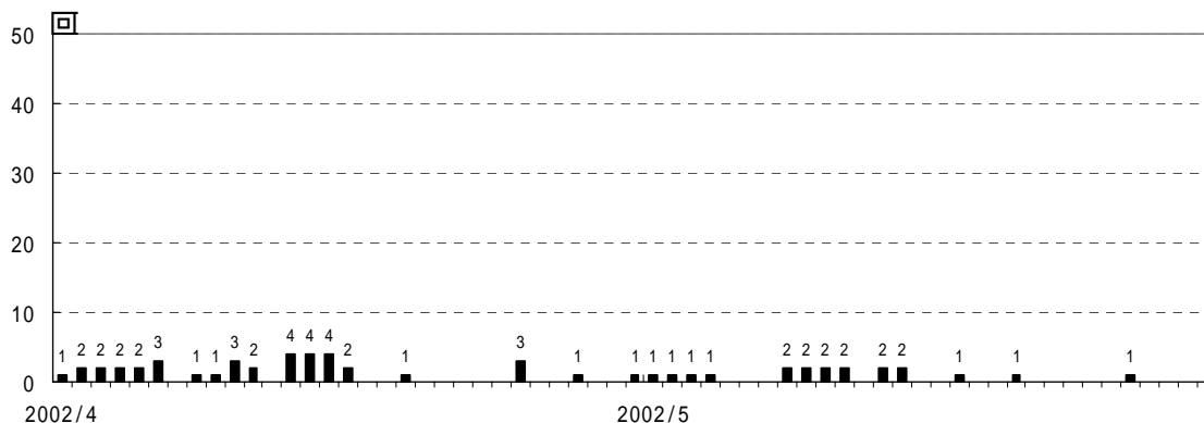
図2 A型地震の発生回数(2002年4月～5月)
