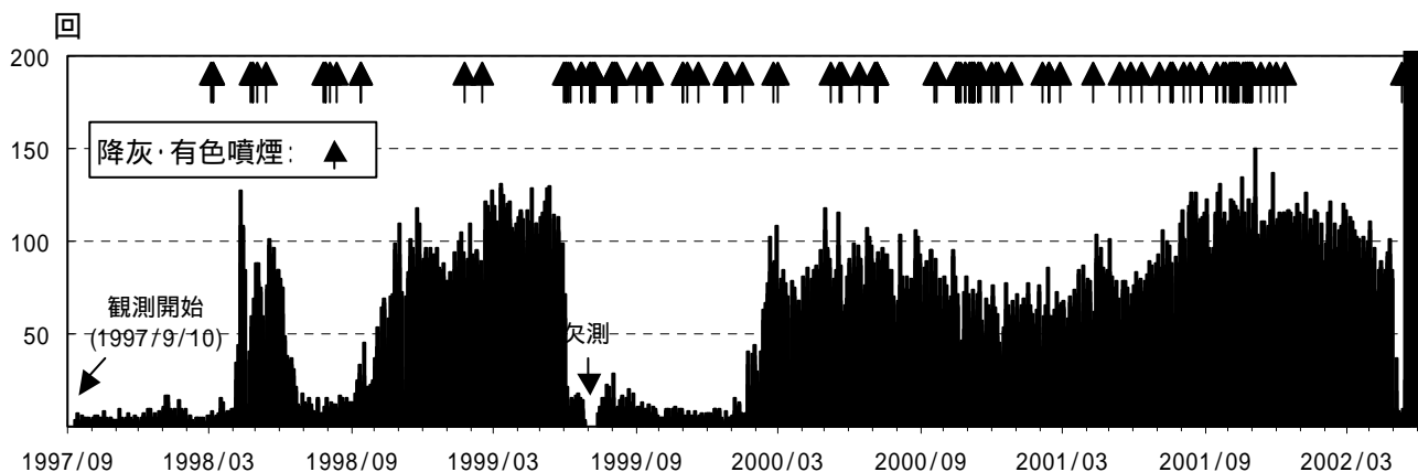
図1 観測開始以来の地震発生回数と噴火(1997年9月～2002年5月)
