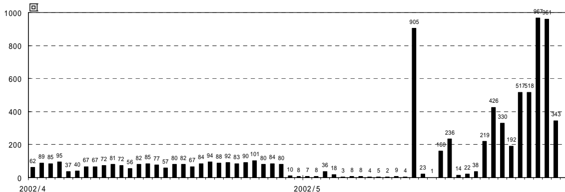
図4 B型地震の日別発生回数(2002年4月~5月)
