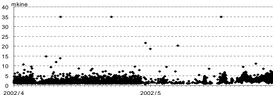
図5 B型地震の最大振幅(U-D成分)分布(2002年4月~5月)
