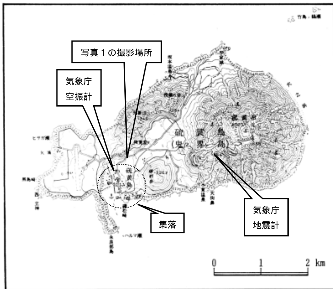
図 7 薩摩硫黄島観測点等位置図
