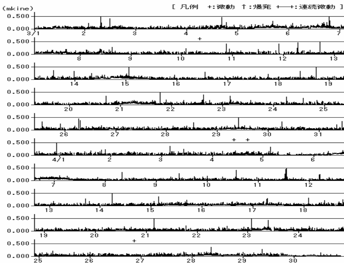
図6 1分間平均振幅(U-D成分)の時間変化(2002年3月~4月)
