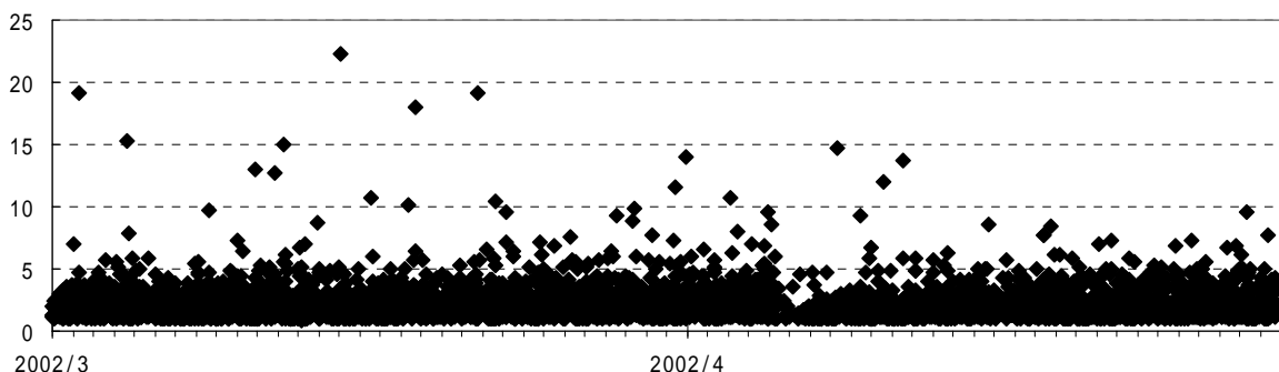
図5 B型地震の最大振幅(U-D成分)分布(2002年3月~4月)
