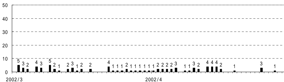
図2 A型地震の発生回数(2002年3月~4月)
