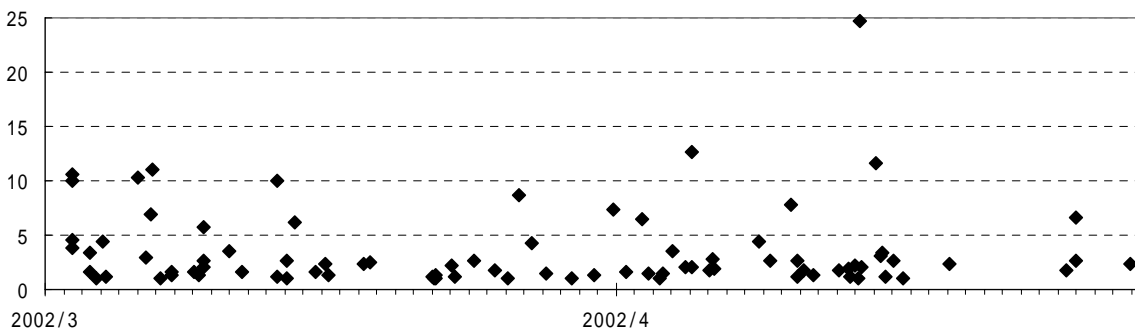
図3 A型地震の最大振幅(U-D成分)分布(2002年3月~4月)
