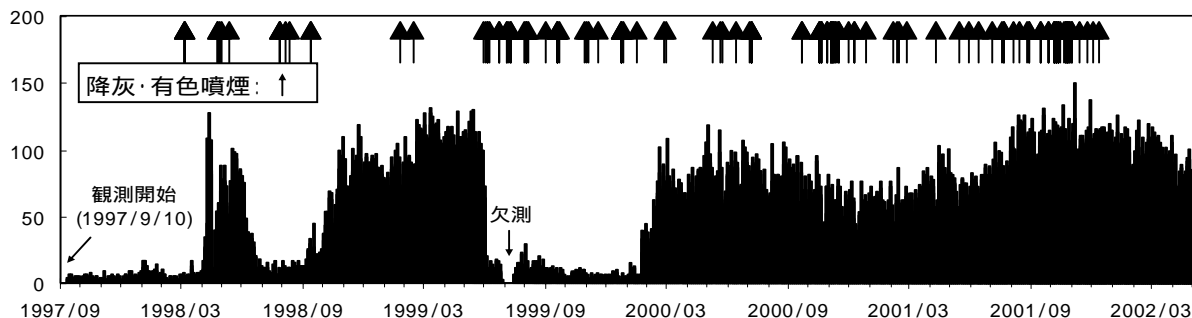
図1 観測開始以来の地震発生回数と噴火(1997年9月~2002年4月)
