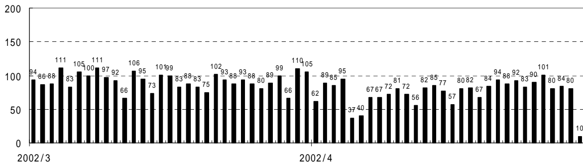
図4 B型地震の日別発生回数(2002年3月~4月)
