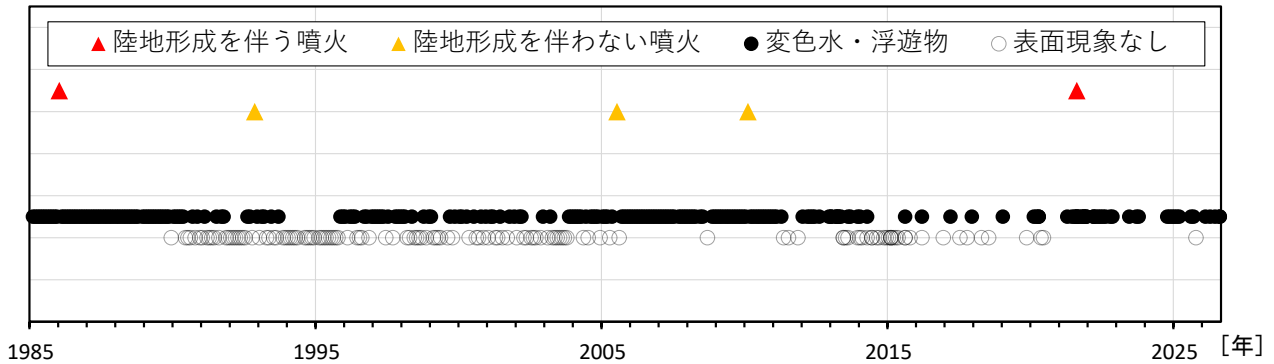
図3 福徳岡ノ場 1985年以降の活動状況
