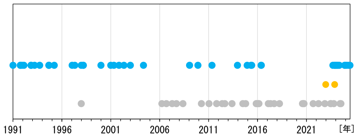
図3 須美寿島 1991年11月以降の活動状況
