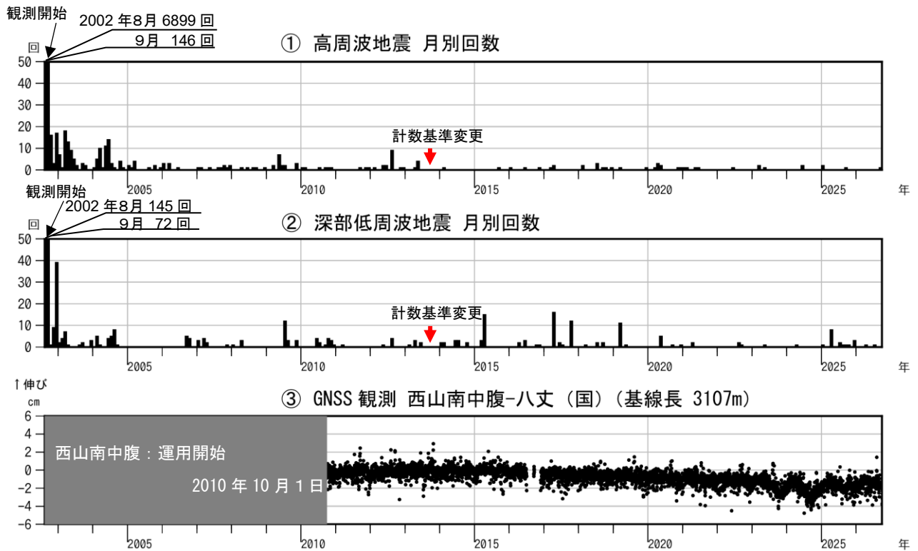
図2 八丈島 火山活動経過図（2002年8月13日～2026年9月30日）
