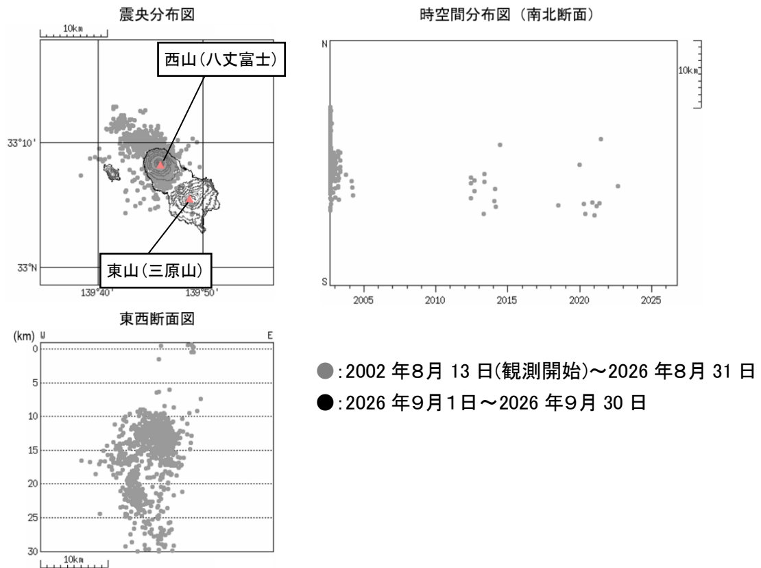
図3 八丈島 震源分布図（2002 年 8 月 13 日～2026 年 9 月 30 日）
