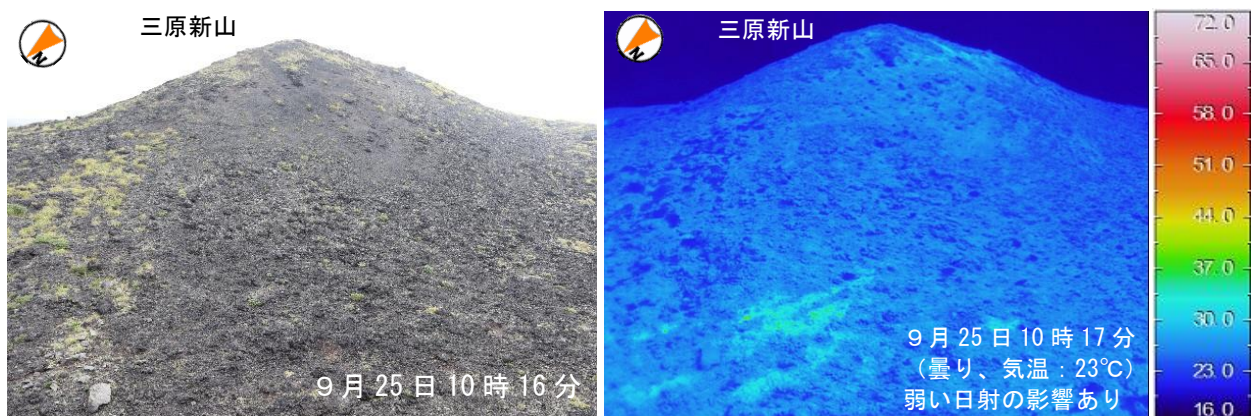
図6-2 伊豆大島 三原新山及び火口原南西の状況（撮影方向は図7参照）
