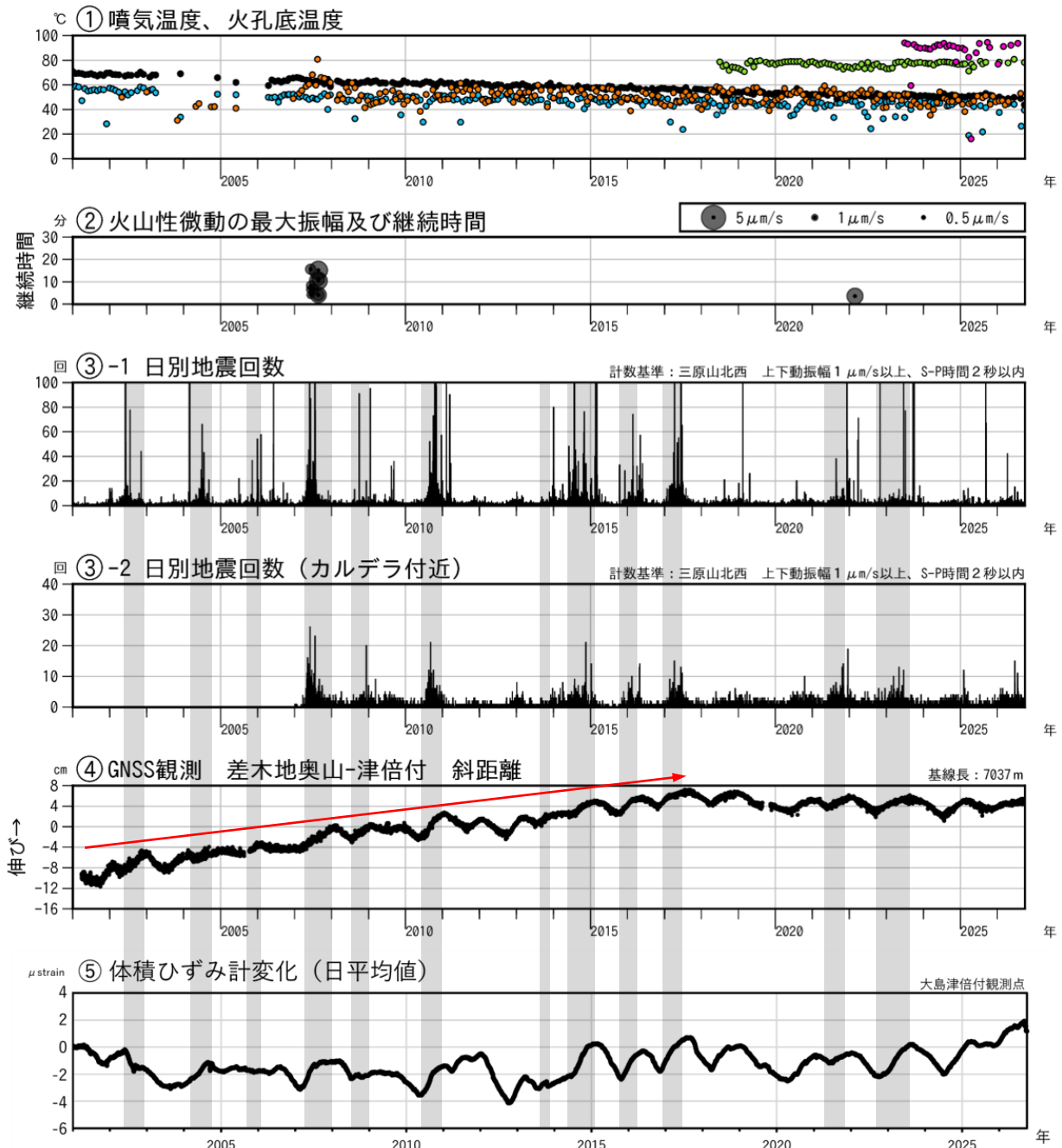
図2 伊豆大島 最近の火山活動経過図（2001年1月～2026年9月）
