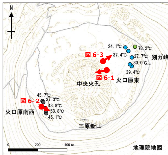
図7 伊豆大島 噴気温度の分布及び現地調査での撮影位置・撮影方向
