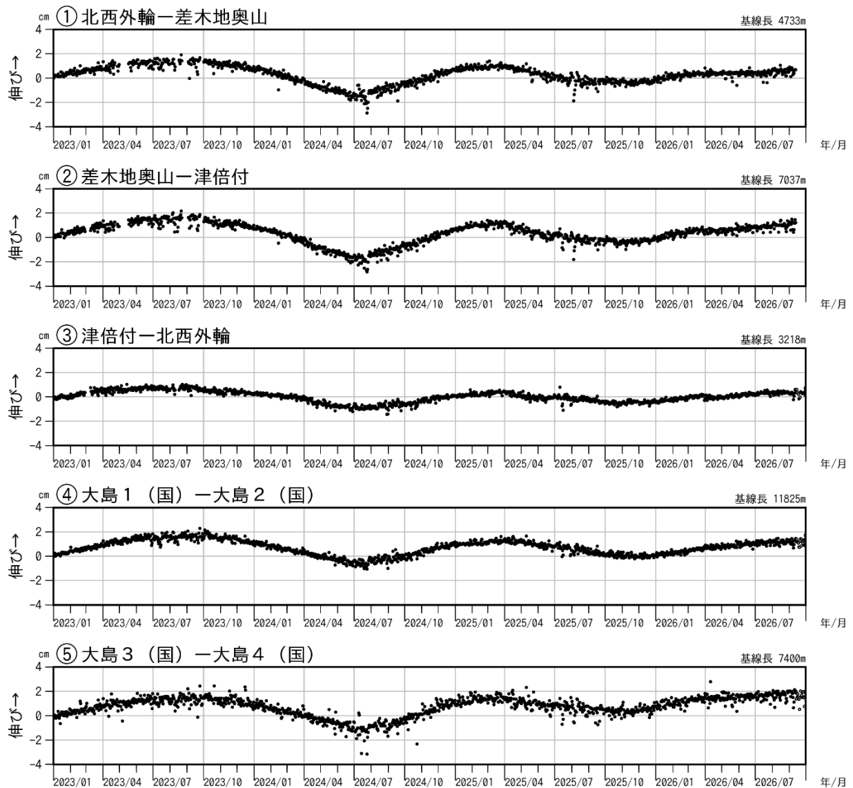
図 3-2 伊豆大島 GNSS 連続観測による基線長変化 (2023 年 1 月～2026 年 9 月)
