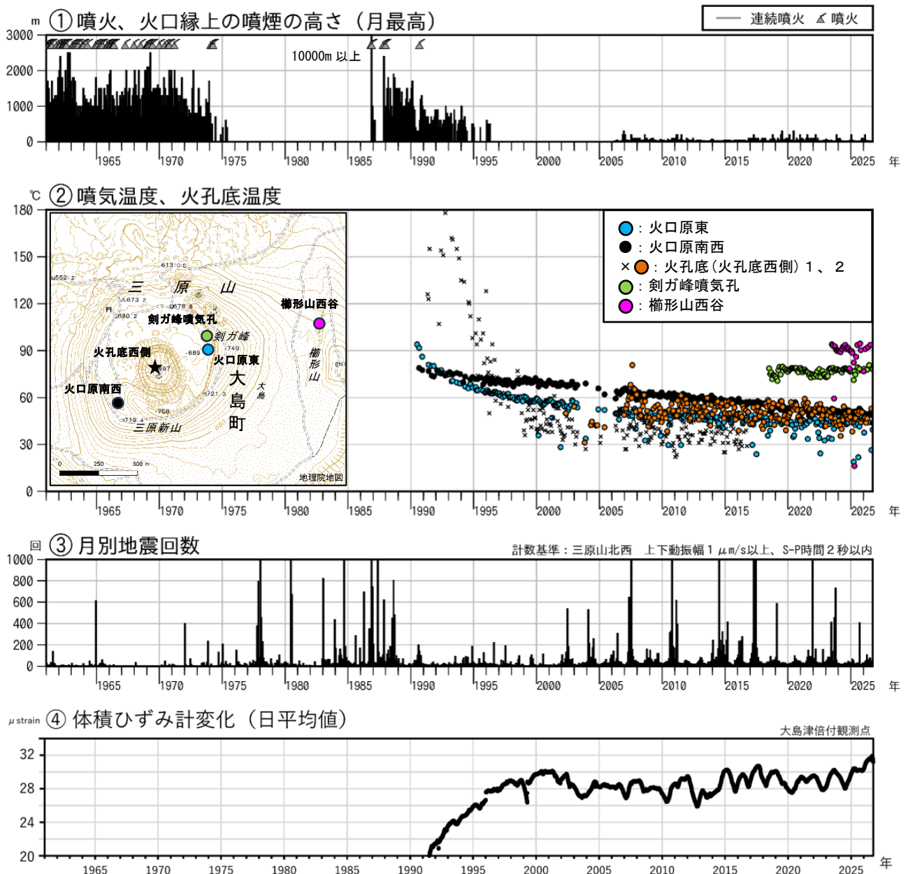
図1 伊豆大島 長期間の火山活動経過図（1961年1月～2026年9月）
