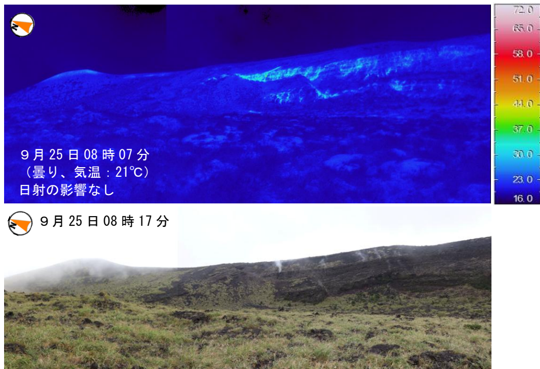
図6-3 伊豆大島 剣ガ峰の状況（撮影方向は図7参照）
