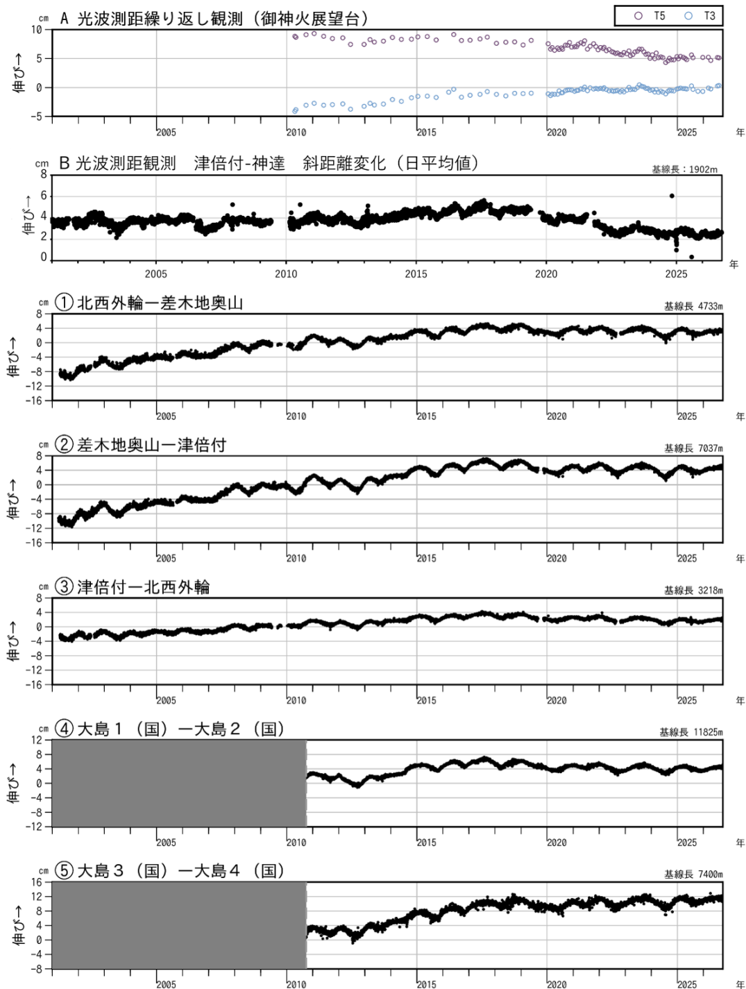
図3-1 伊豆大島 GNSS 連続観測及び光波測距観測による基線長変化(2001年1月～2026年9月)
