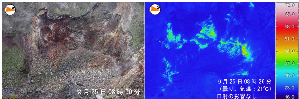
図6-1 伊豆大島 中央火孔内の状況（撮影方向は図7参照）
