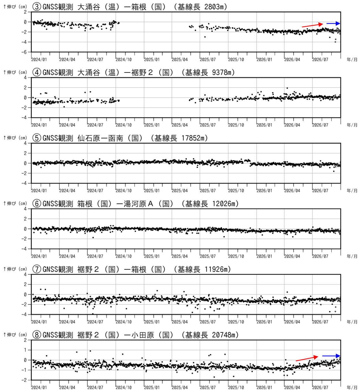
図3－3 箱根山 GNSS 連続観測による基線長変化（2024 年 1 月 1 日～2026 年 9 月 30 日）
