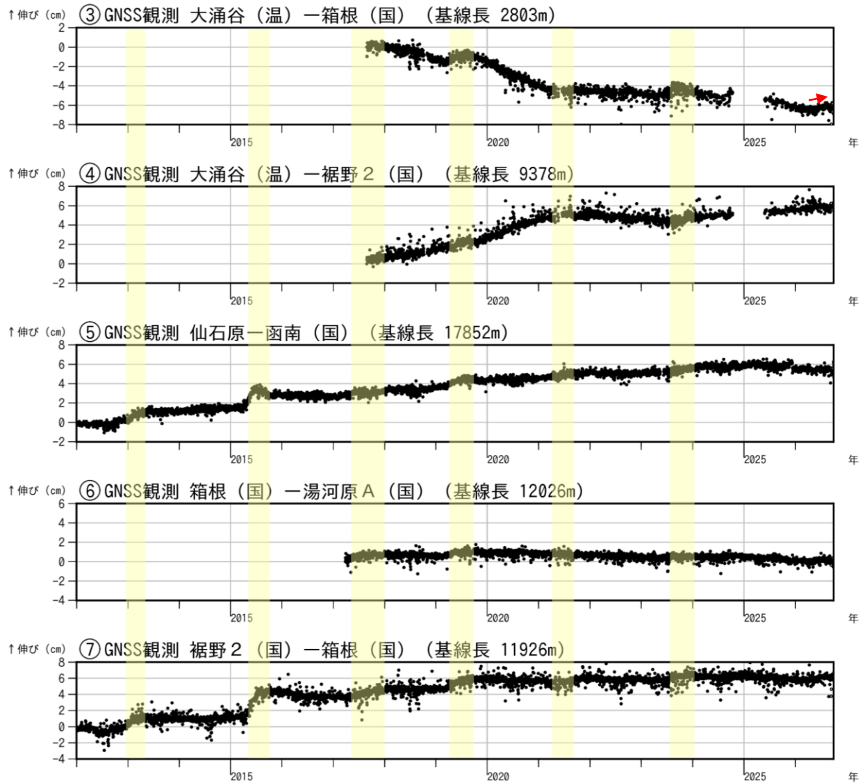
図3-2 箱根山 GNSS 連続観測による 基線長変化及び観測点配置図 (2012年1月1日～2026年9月30日)
