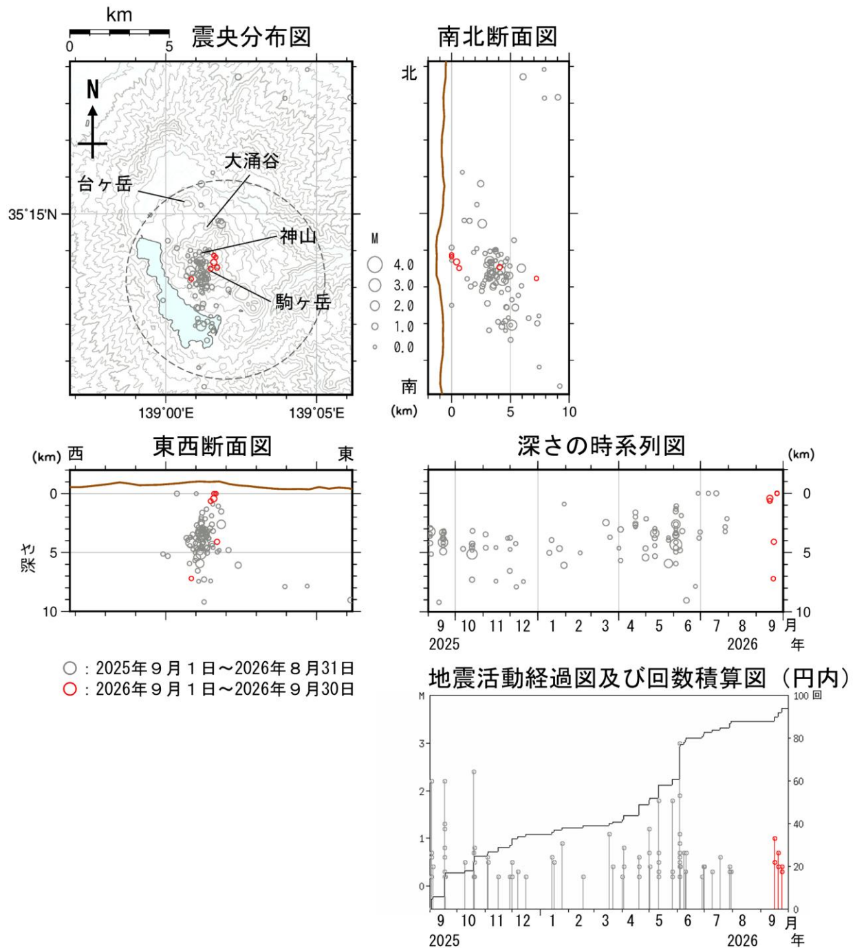
図4 箱根山 広域地震観測網による山体周辺の震源分布図（2025年9月1日～2026年9月30日）
