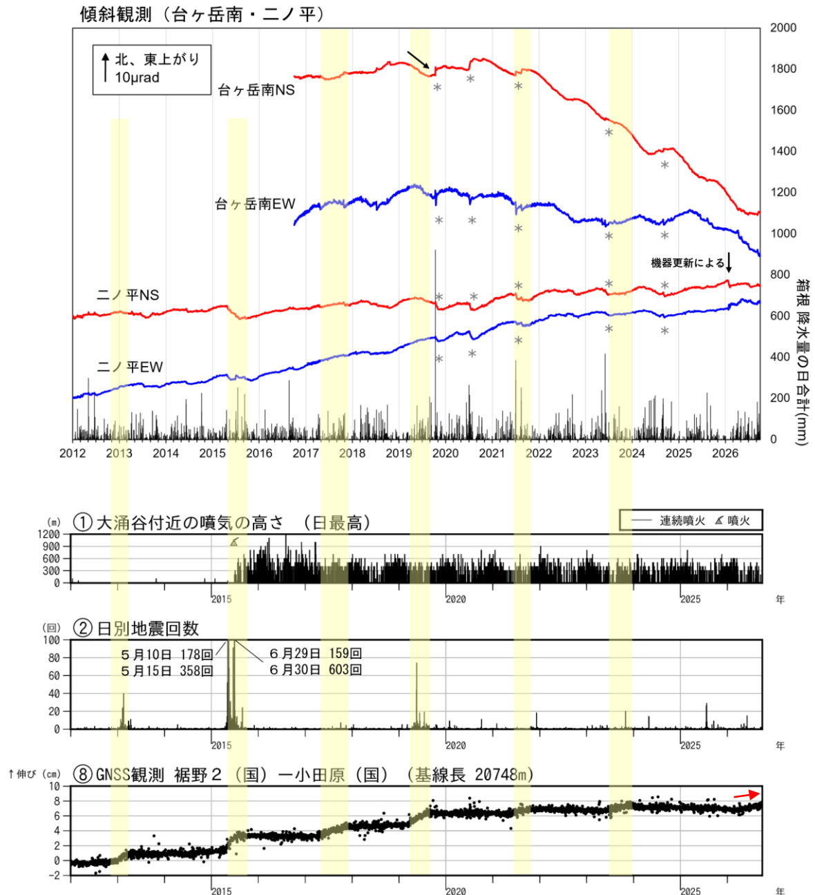
図3-1 箱根山 火山活動経過図（2012年1月1日～2026年9月30日）
