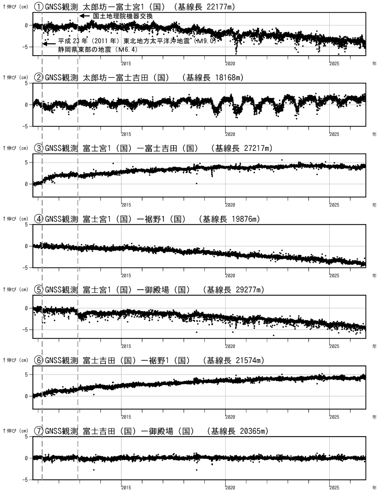
図4 富士山 GNSS 連続観測による基線長変化 (2010年10月1日～2026年9月30日) (国): 国土地理院 「平成23年(2011年)東北地方太平洋沖地震」及び2011年3月15日に発生した静岡県東部の地震(M6.4)によるステップ状の変化を補正しています。 ①～⑦は図5のGNSS基線①～⑦に対応しています。
