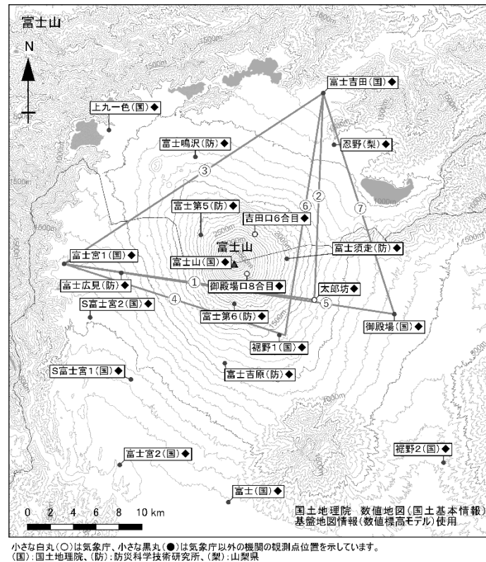
図5 富士山 GNSS観測点配置図
