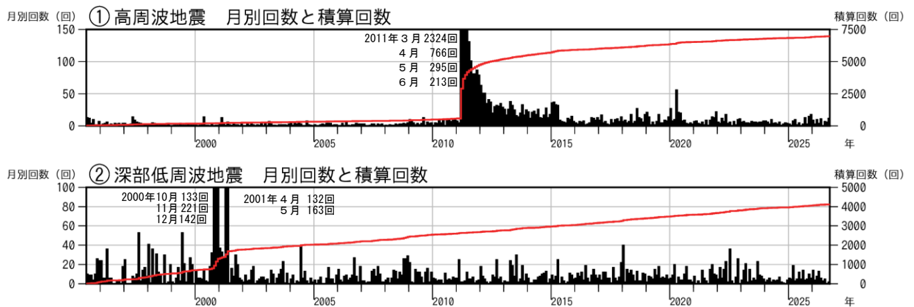
図2 富士山 月別地震回数（1995年6月1日～2026年9月30日）
