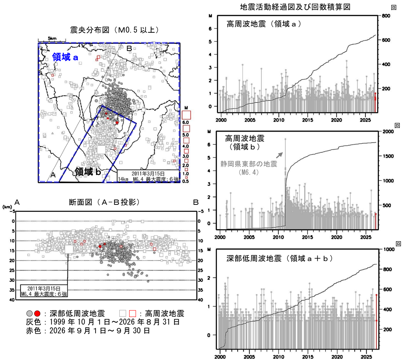
図3 富士山 広域地震観測網による山体及び周辺の地震活動(1999年10月1日～2026年9月30日)
