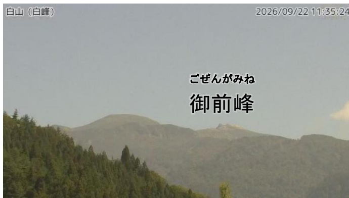
図1 白山 山頂部の状況 （9月22日 白峰監視カメラによる）
