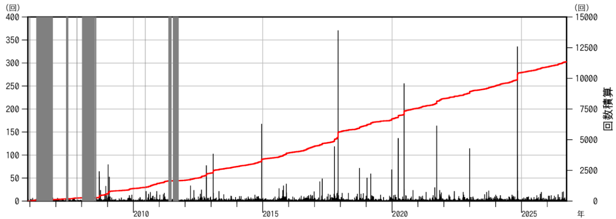
図3 白山 日別地震回数と積算回数（2005年12月1日～2026年9月30日） 図の灰色部分は機器障害による欠測期間。赤線は積算回数を示します。
