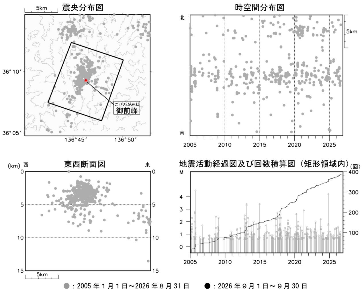
図4 白山 広域地震観測網による山体・周辺の地震活動（2005年1月1日～2026年9月30日） 広域地震観測網により震源決定したもので、深さは全て海面以下として決定しています。なお、2020年9月以降については、地震観測点の標高を考慮する等、震源決定の手法を変更しています。 M（マグニチュード）は地震の規模を表します。M0.6以上の地震を表示しています。 図中の震源要素は一部暫定値を含んでおり、後日変更することがあります。 ・今期間、白山付近の地震活動は低調に経過しました。
