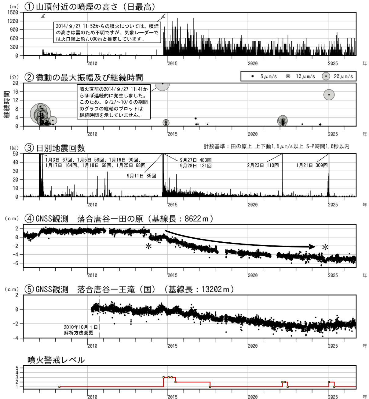
図1 御嶽山 長期間の火山活動経過図（2006年1月1日～2026年9月30日）
