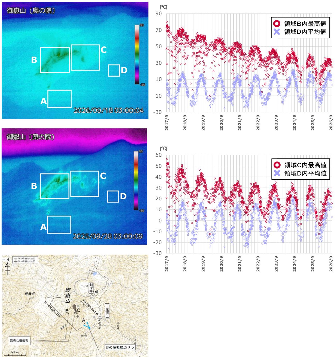
図3 御嶽山 奥の院赤外熱映像カメラによる地獄谷火口における最高温度の推移 (2017年9月13日～2026年9月30日)
