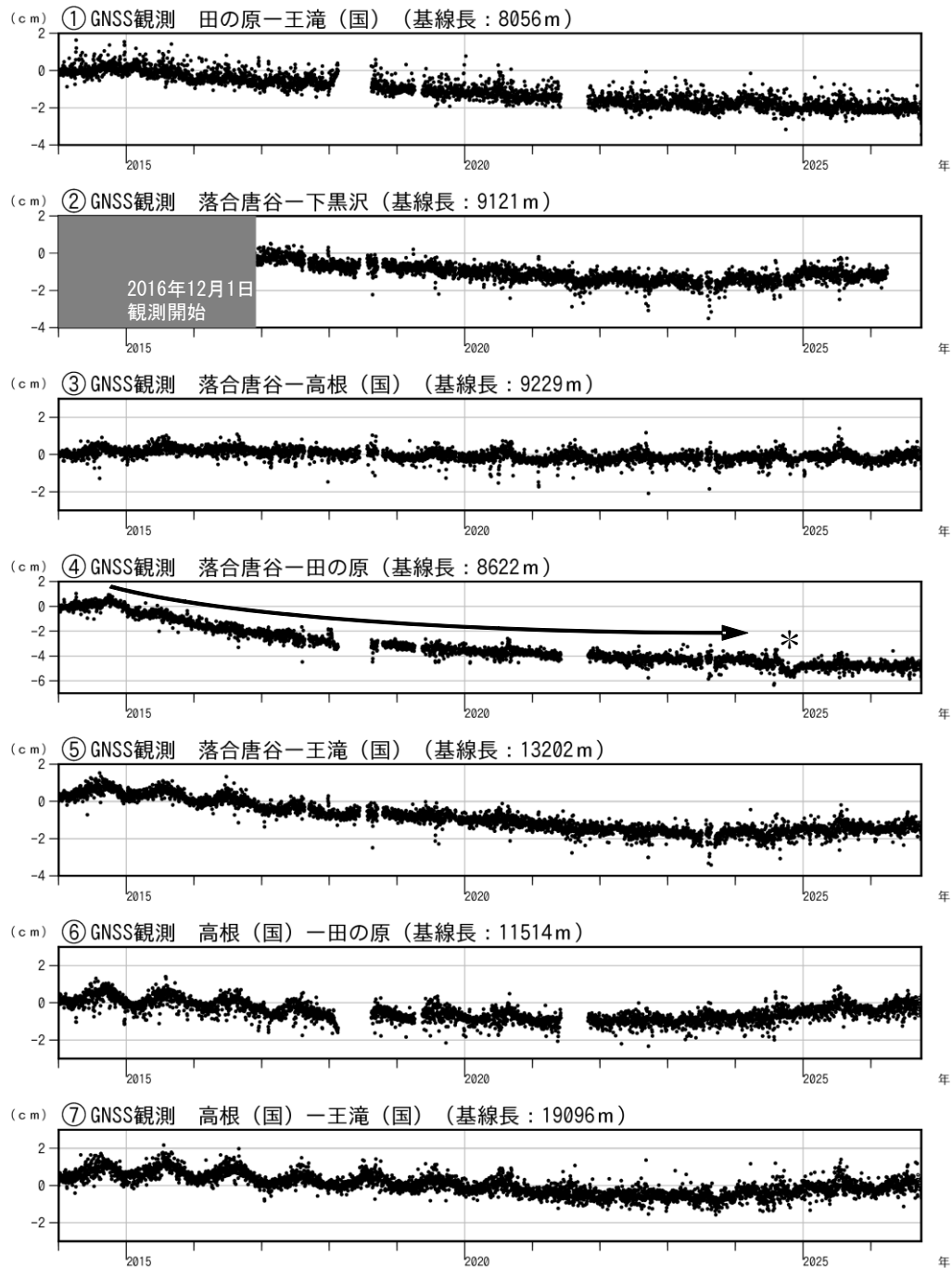
図5 御嶽山 GNSS 連続観測結果（2014年1月1日～2026年9月30日）
