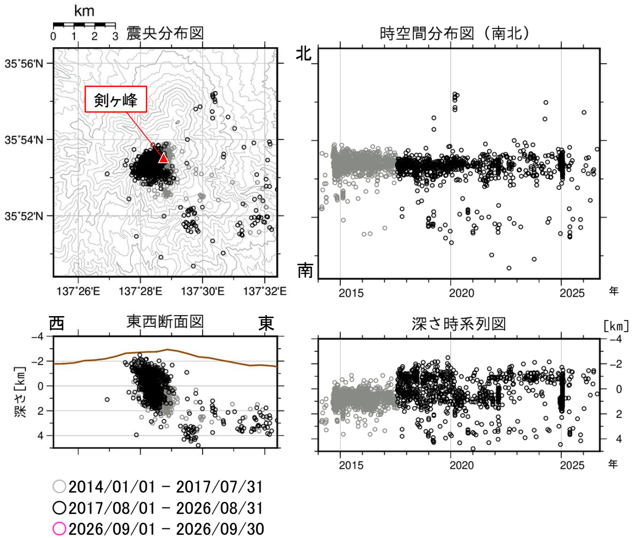
図4 御嶽山 震源分布図（2014年1月1日～2026年9月30日） 2017年8月1日以降の震源分布は、震源計算に使用する観測点を新たに追加して再計算したものを示しています。 観測点の移動状況により、求まる震源の数の減少や位置の精度低下が生じる場合があります。
