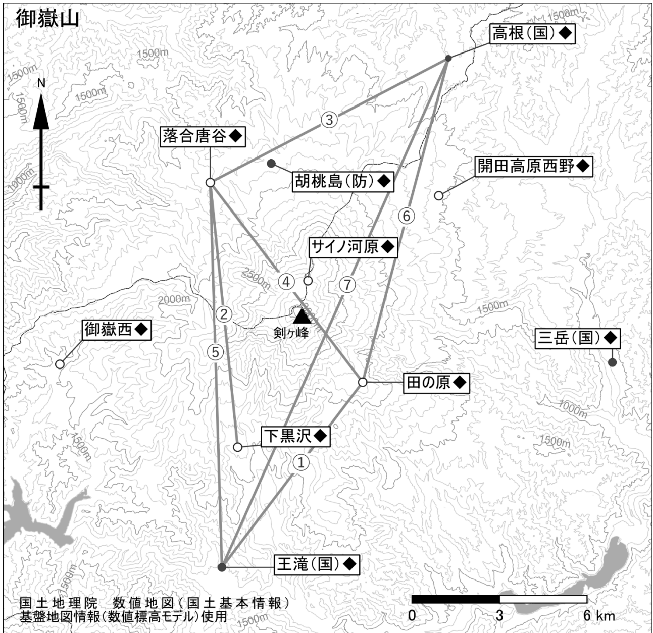
図6 御嶽山 GNSS 連続観測点と基線番号
