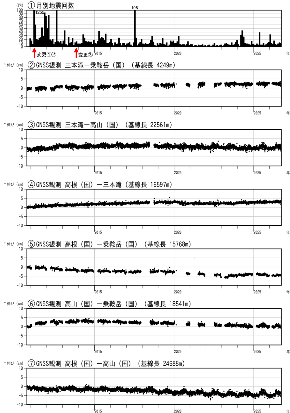
図2 乗鞍岳 火山活動経過図（2010年10月1日～2026年9月30日）
