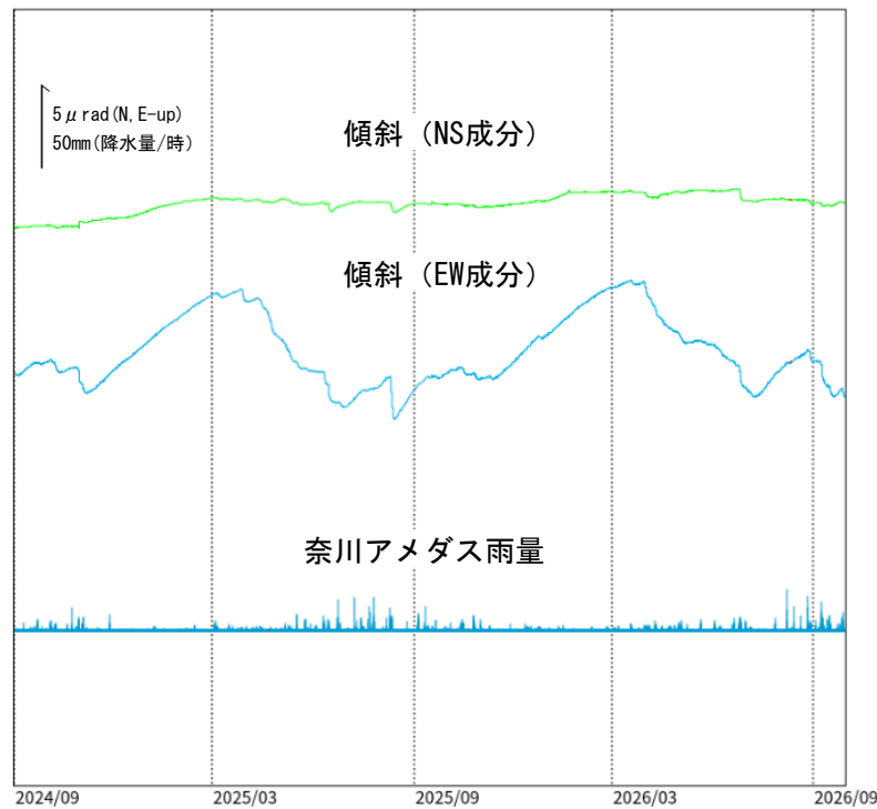
図4 乗鞍岳 三本滝観測点における傾斜データ（2024年9月1日～2026年9月30日） ・傾斜計による観測では、火山活動によるとみられる変動は認められません。
