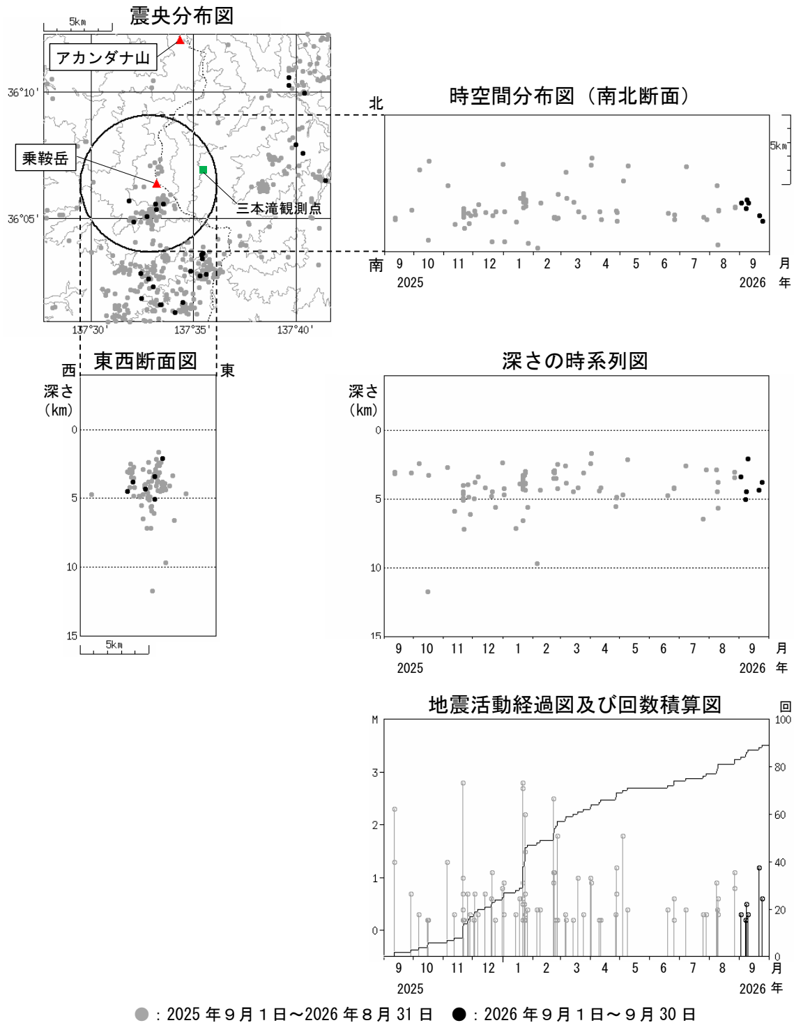
図3 乗鞍岳 広域地震観測網による山体・周辺の地震活動(2025年9月1日～2026年9月30日)
