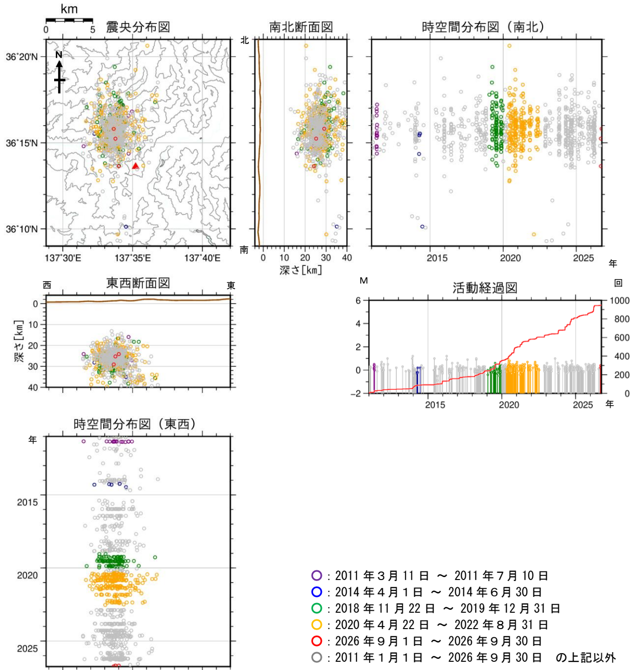
図10 焼岳 広域地震観測網による深部低周波地震の震源分布図（2011年1月1日～2026年9月30日）
