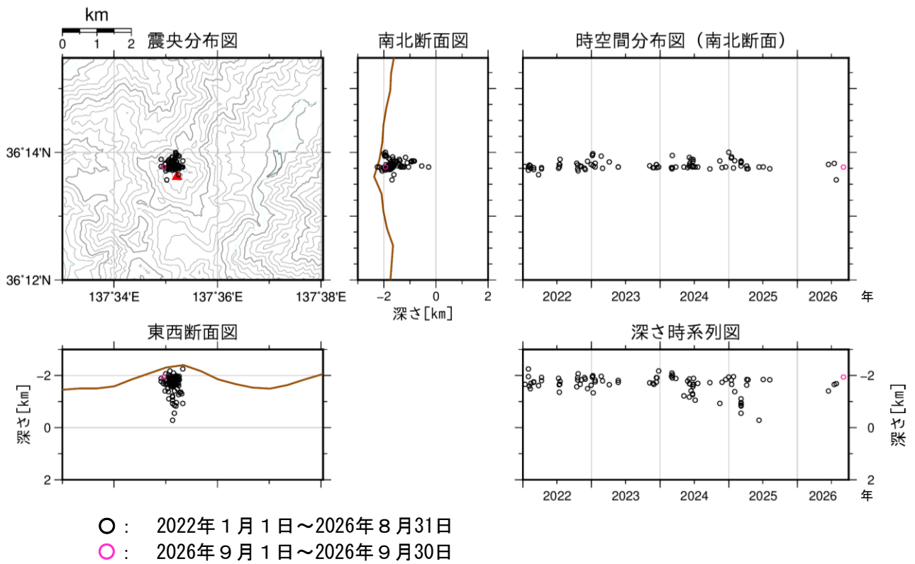
図2 焼岳 山頂付近の地震の震源分布図（2022年1月1日～2026年9月30日）
