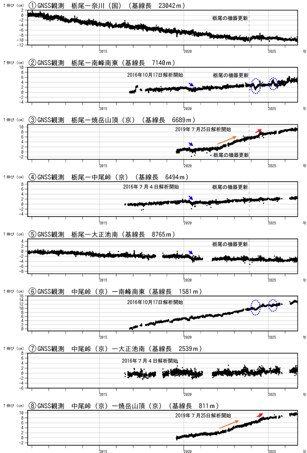
図6 焼岳 GNSS 連続観測による基線長変化（2010年10月1日～2026年9月30日）
