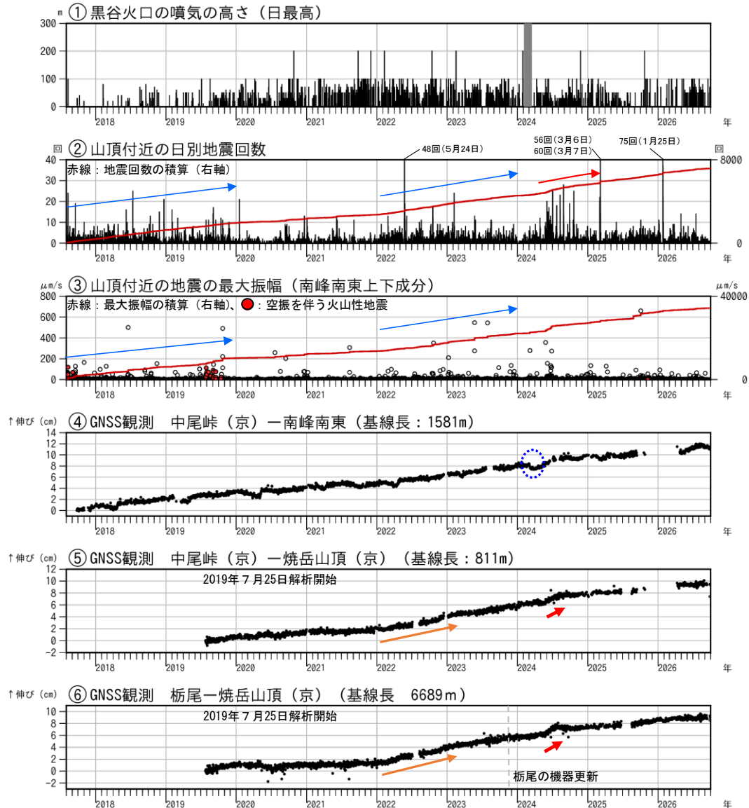
図1 焼岳 火山活動経過図（2017年8月1日～2026年9月30日）
