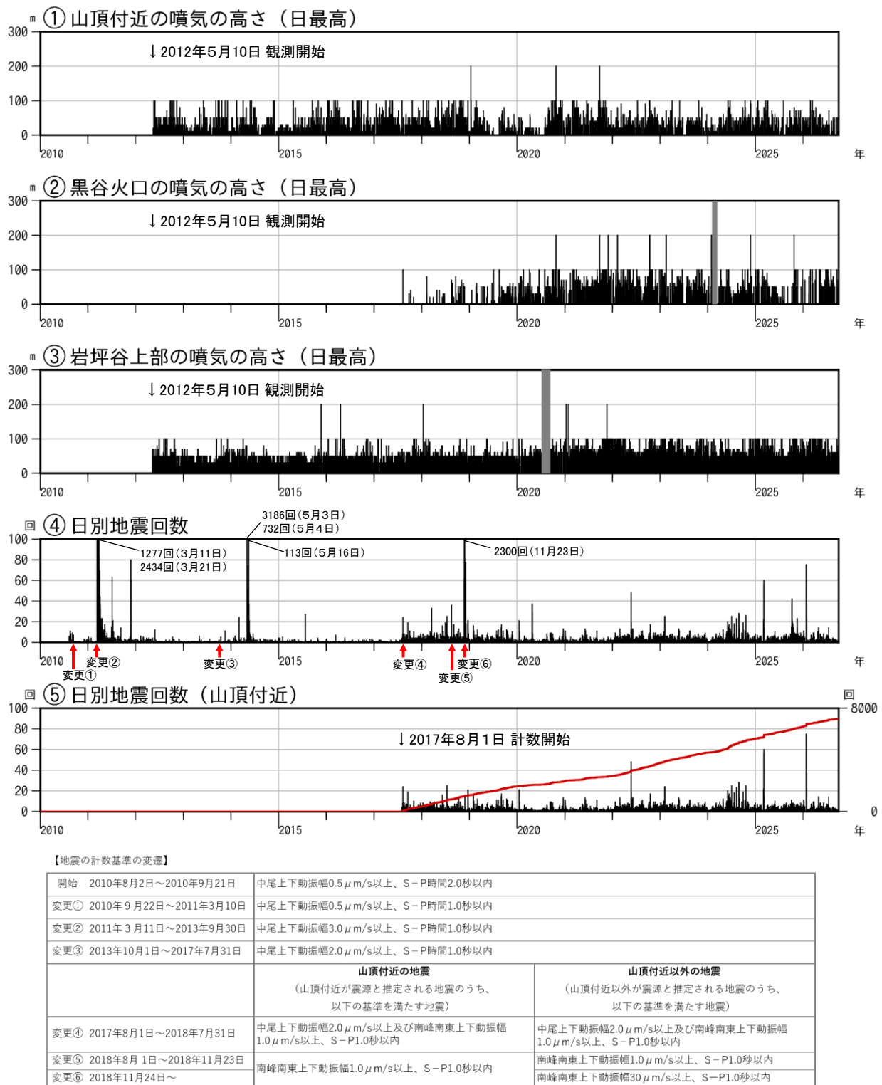
図5 焼岳 噴気の高さと地震回数の推移(2010年8月2日～2026年9月30日)
