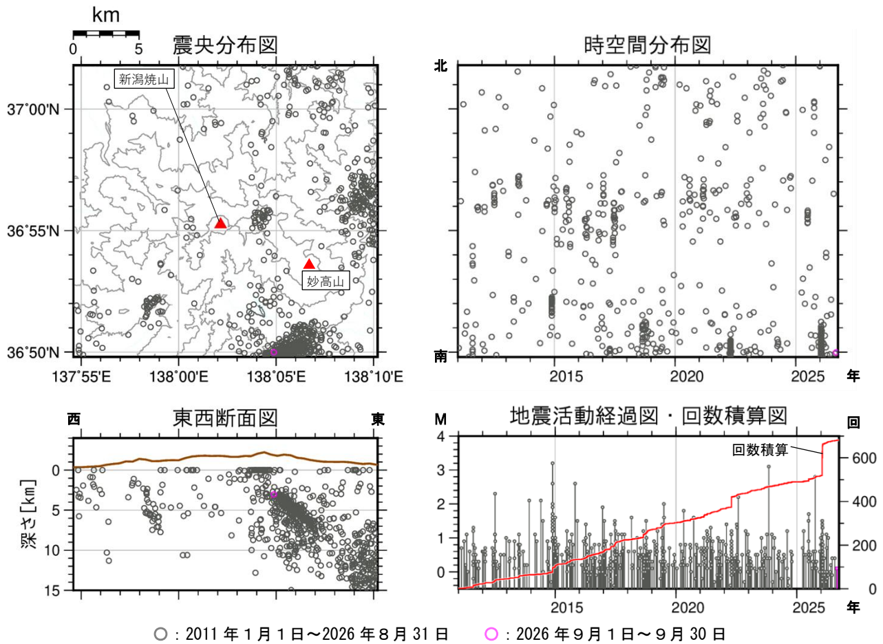
図4 新潟焼山 広域地震観測網による山体・周辺の地震活動（2011 年 1 月 1 日～2026 年 9 月 30 日） 広域地震観測網により震源決定したもので、深さは全て海面以下として決定しています。なお、2020 年 9 月以降については、地震観測点の標高を考慮する等、震源決定の手法を変更しています。 図中の震源要素は一部暫定値が含まれており、後日変更することがあります。
