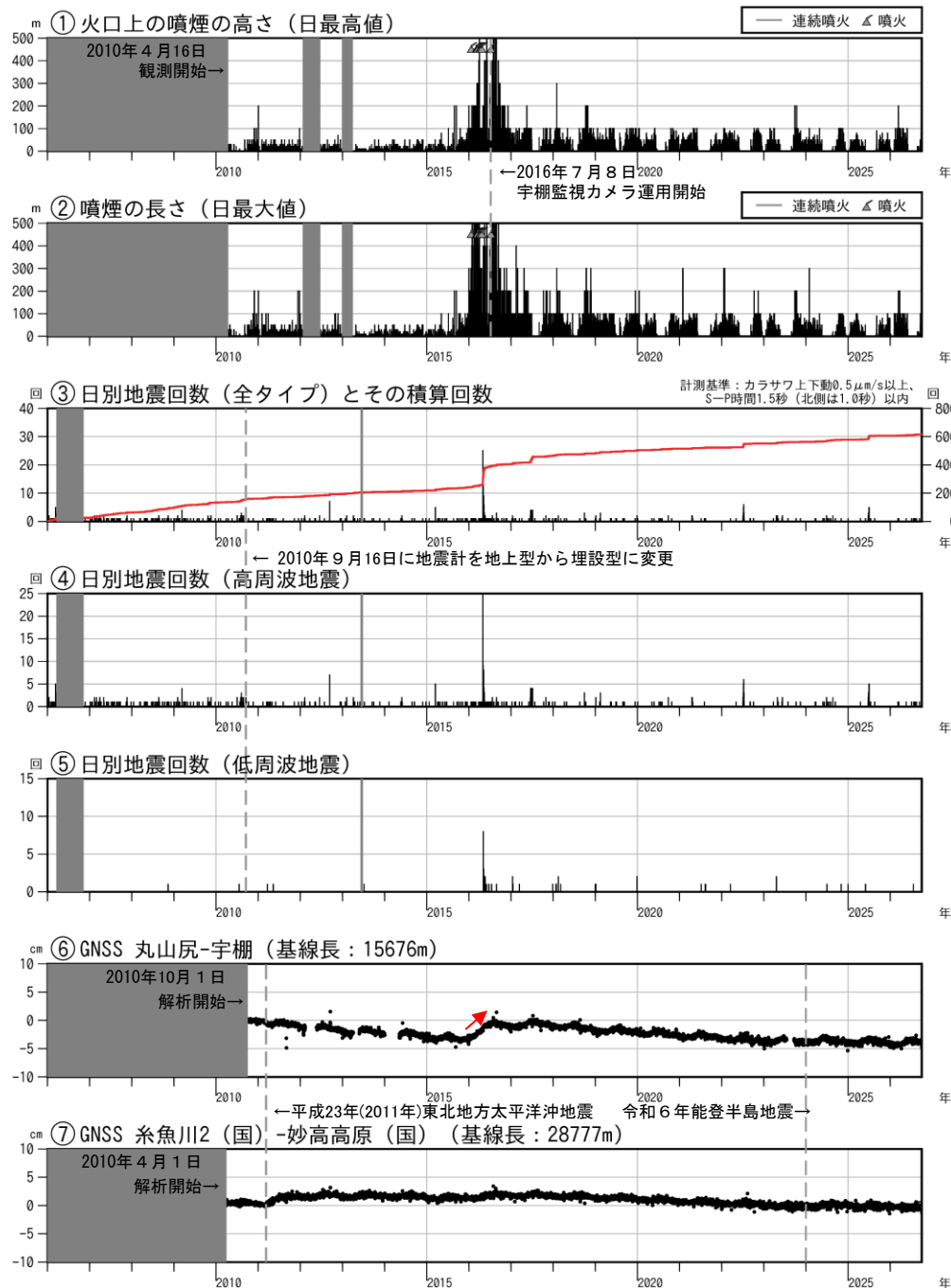
図2 新潟焼山 火山活動経過図（2006年1月1日～2026年9月30日）
