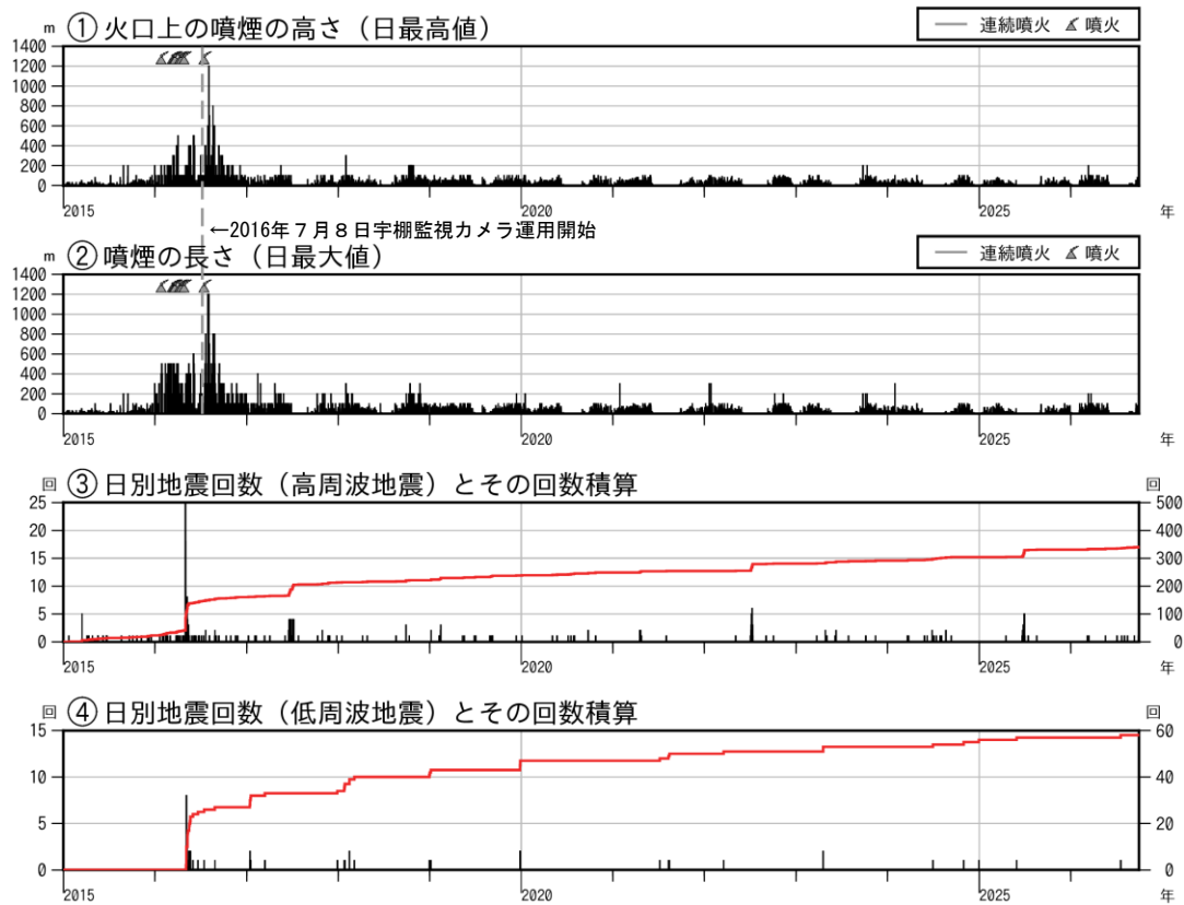
図3 新潟焼山 火山活動経過図（短期）（2015年1月1日～2026年9月30日）
