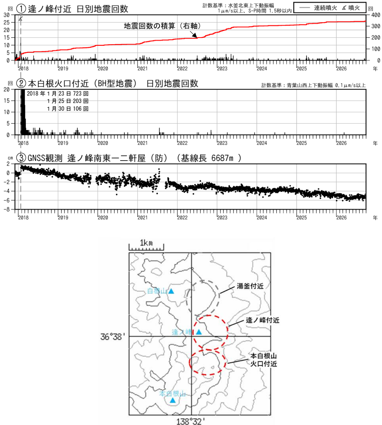
図13 草津白根山（本白根山） 火山活動経過図（2017年12月1日～2026年9月30日）
