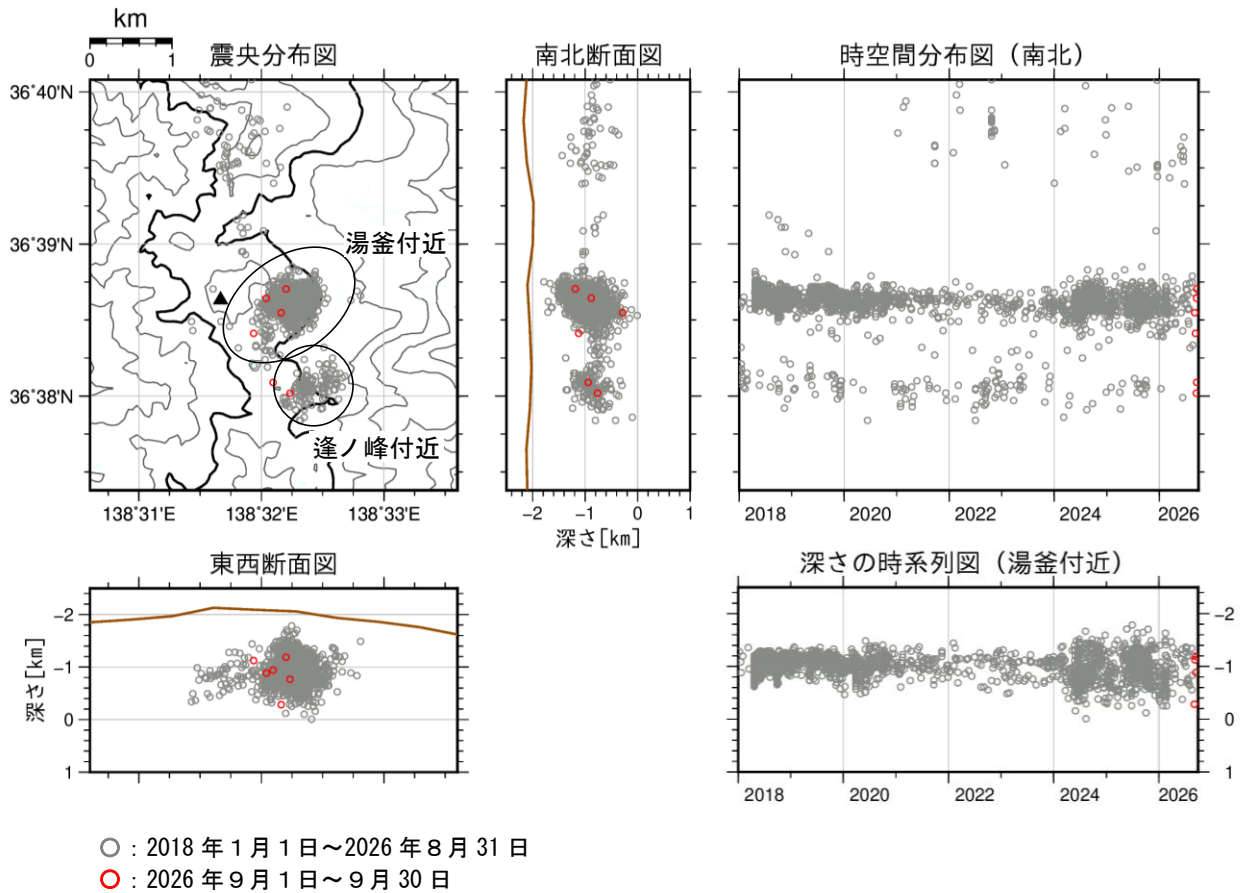
図4 草津白根山 震源分布図（2018 年 1 月 1 日～2026 年 9 月 30 日）
