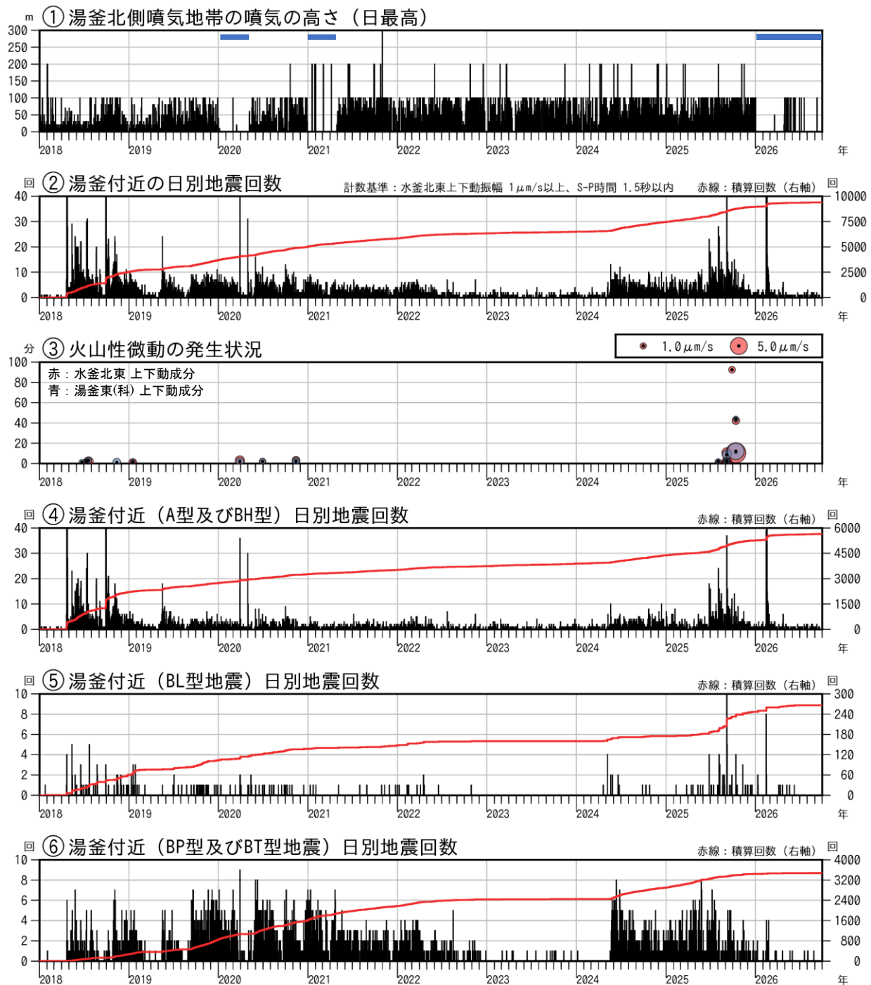
図3 草津白根山（白根山（湯釜付近）） 火山活動経過図（2018年1月1日～2026年9月30日）
