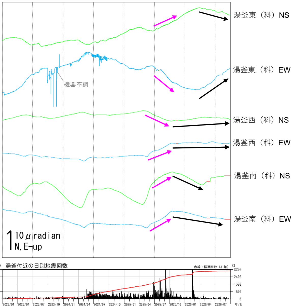
図5 草津白根山（白根山（湯釜付近）） 傾斜変動及び日別地震回数 (2023年1月1日～2026年9月30日)
