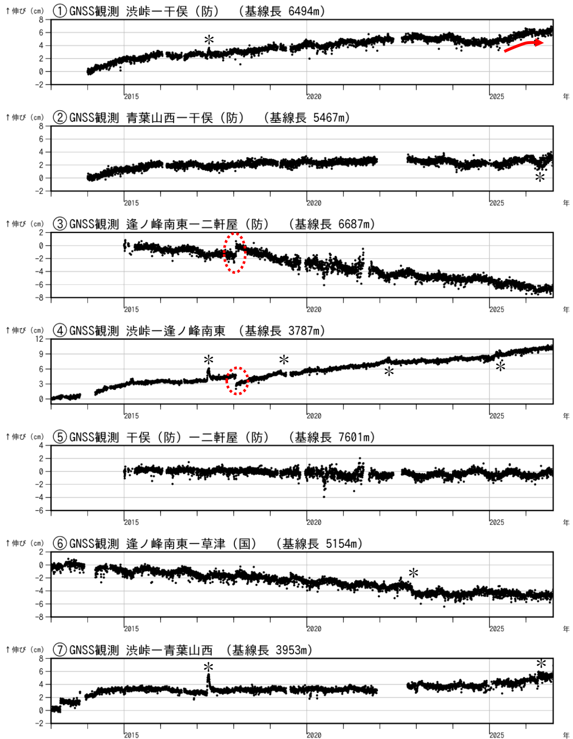
図6 草津白根山 GNSS 連続観測結果（2013年1月1日～2026年9月30日）
