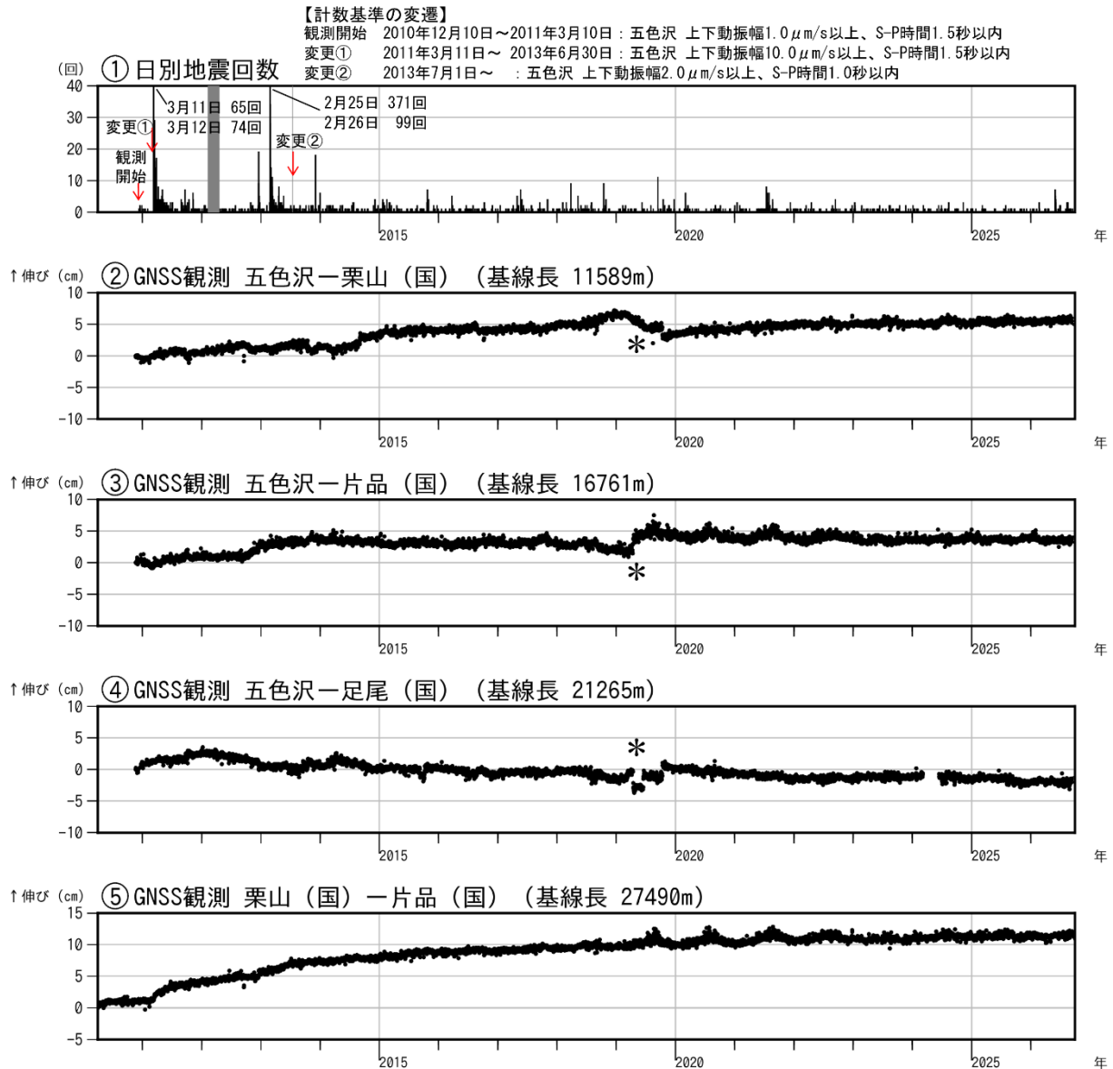
図2 日光白根山 火山活動経過図（2010年4月1日～2026年9月30日）
