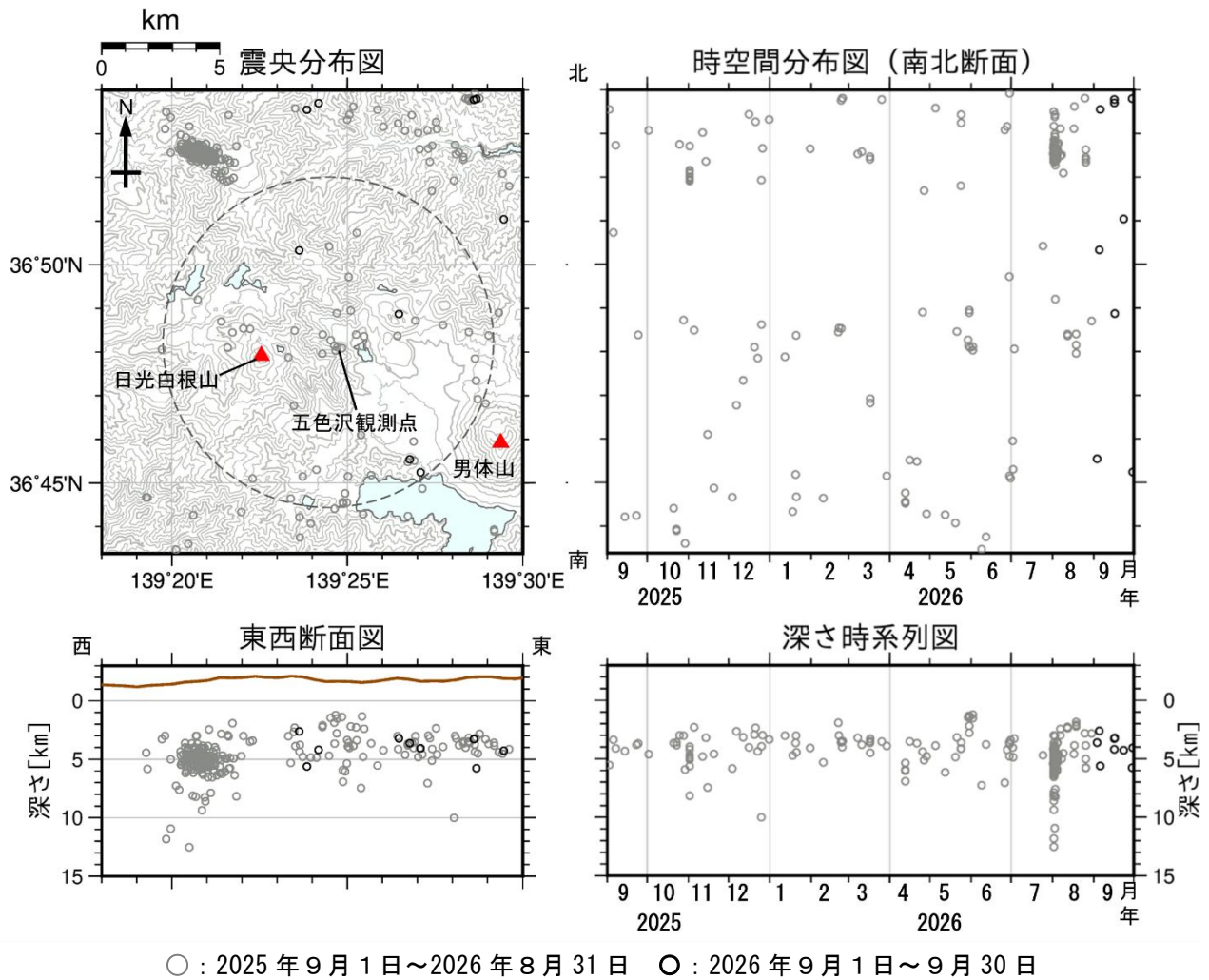
図3 日光白根山 広域地震観測網による山体周辺の地震活動 (2025 年 9 月 1 日～2026 年 9 月 30 日)
