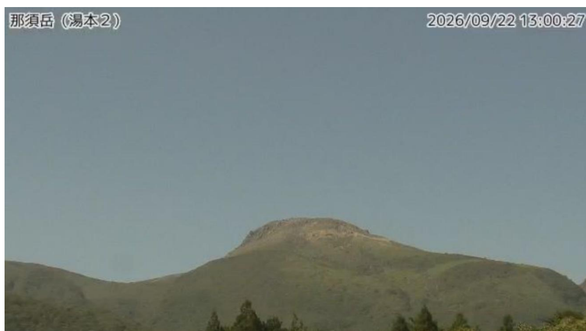
図1 那須岳 茶臼岳の状況（9月22日、湯本2監視カメラによる）
