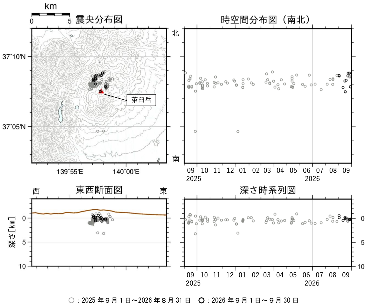
図5 那須岳 震源分布図（2025 年 9 月 1 日～2026 年 9 月 30 日）
