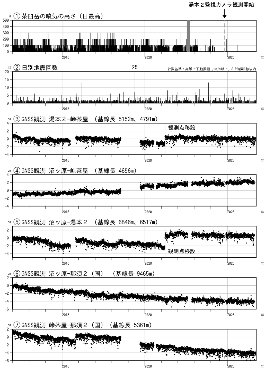
図4 那須岳 火山活動経過図（2012年1月1日～2026年9月30日）
