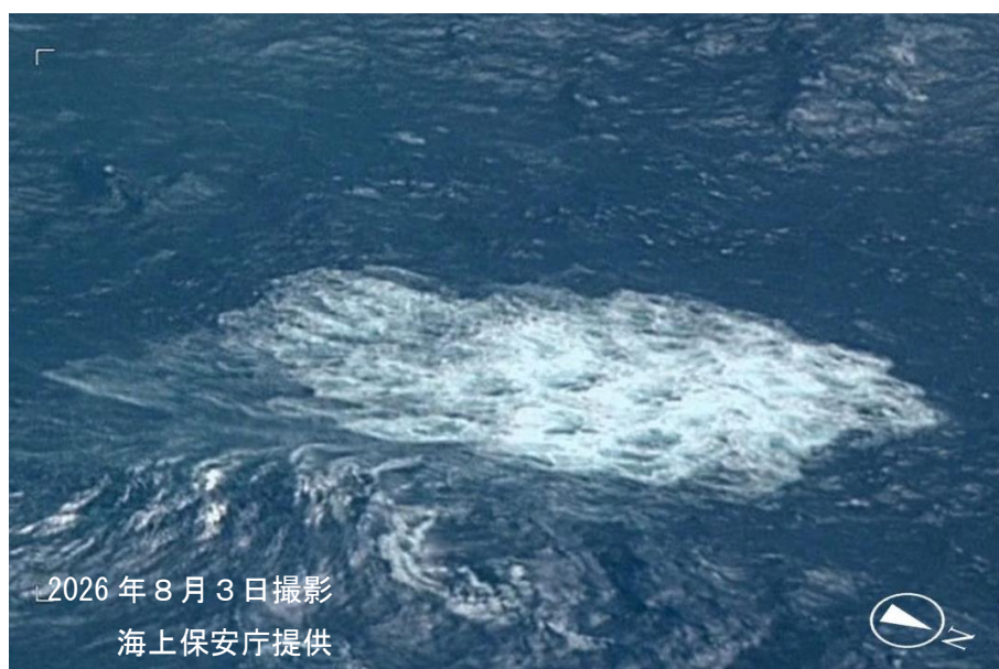
図2 福德岡ノ場全景（上）および気泡の噴出（下）
