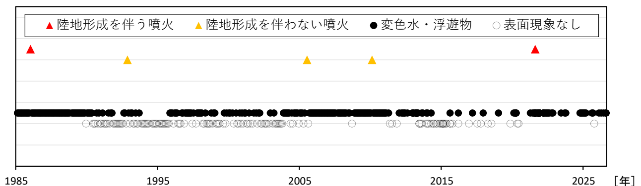
図4 福徳岡ノ場 1985年以降の活動状況
