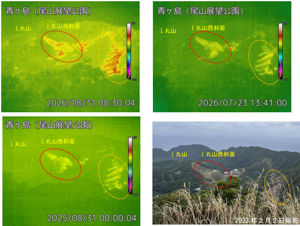
図2 青ヶ島 カルデラ内の地表面温度の状況（左上、右上、左下：尾山展望公園監視カメラによる、右下：2023年2月2日に撮影した同場所からの写真） 左上の画像は、日射の影響を強く受けています。
