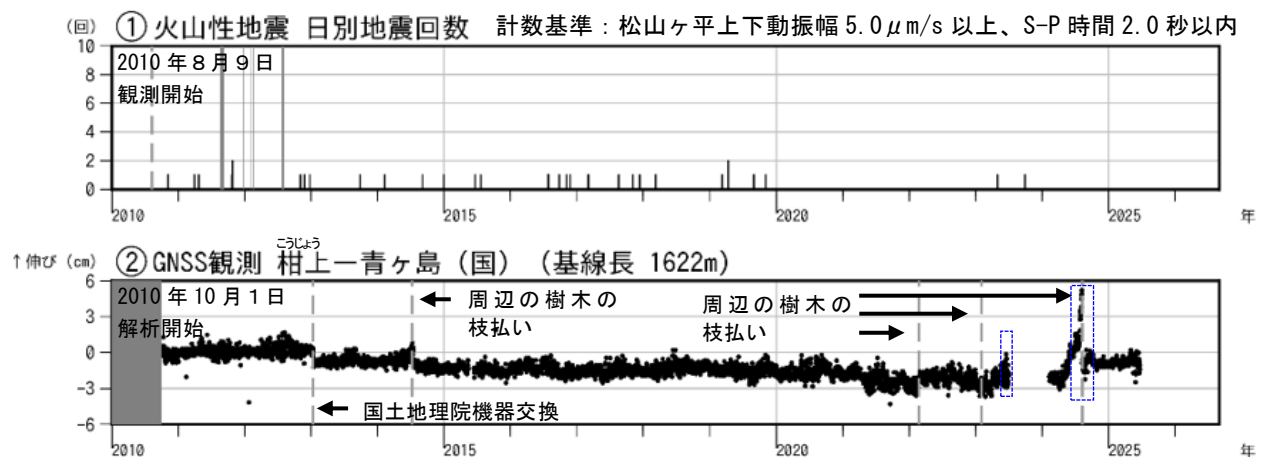
図3 青ヶ島 火山活動経過図（2010年8月9日～2026年8月31日）
