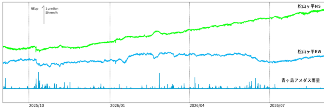
図4 青ヶ島 松山ヶ平観測点における傾斜データ（2025年8月1日～2026年8月31日） ・傾斜計による観測では、火山活動によるとみられる変動は認められません。
