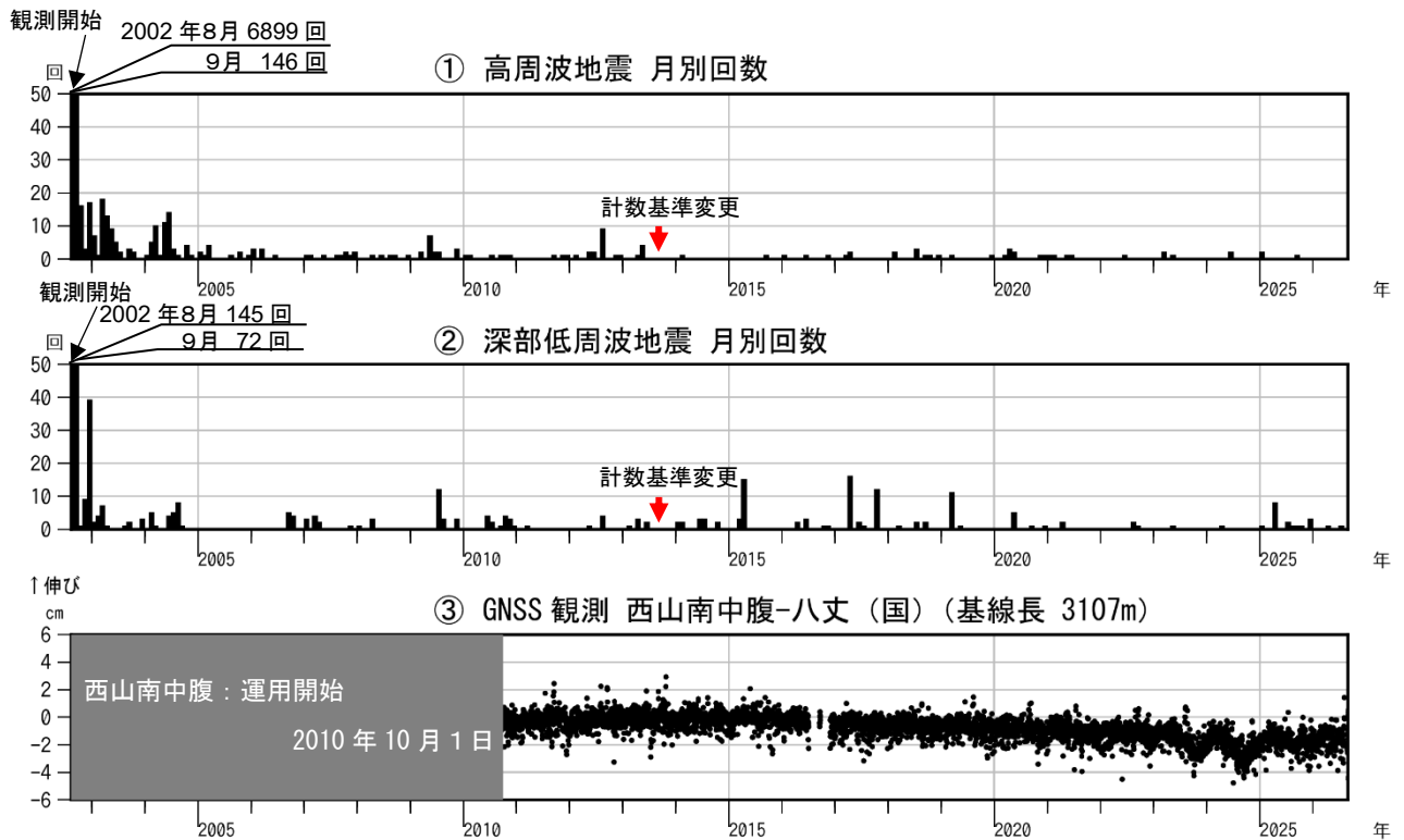
図2 八丈島 火山活動経過図（2002年8月13日～2026年8月31日）
