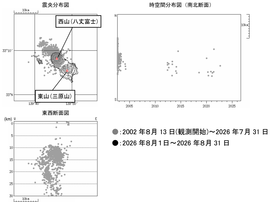
図3 八丈島 震源分布図（2002 年 8 月 13 日～2026 年 8 月 31 日）
