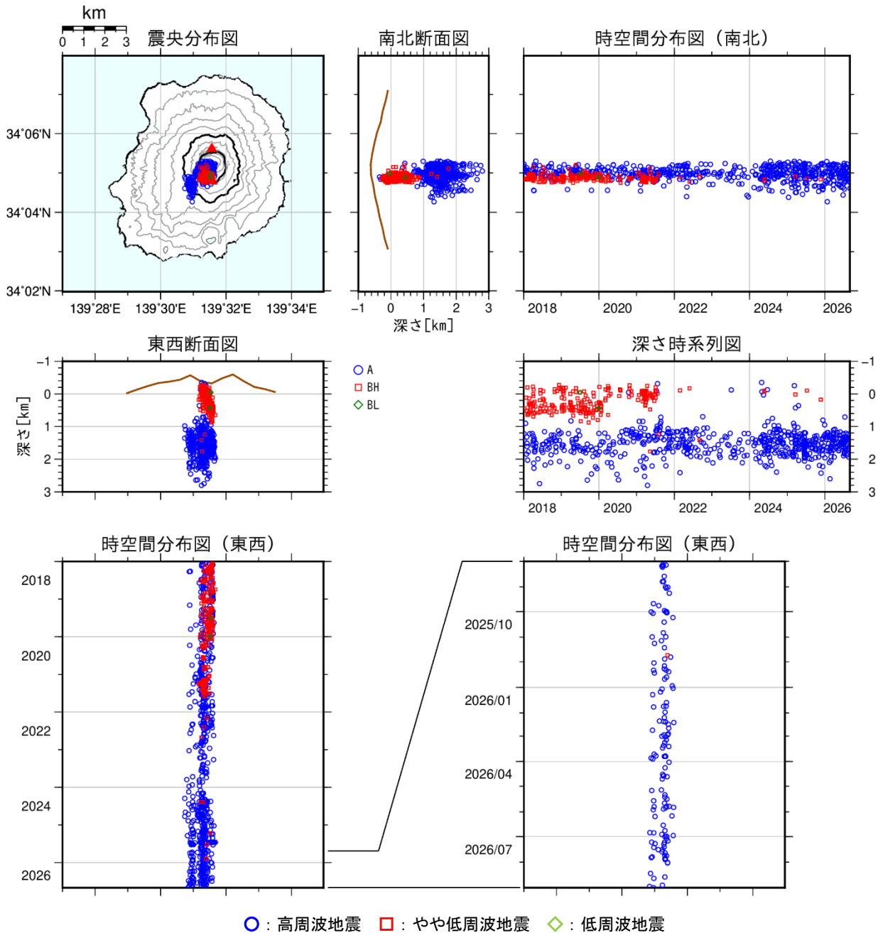
図7 三宅島 震源分布図（2018年1月1日～2026年8月31日）
