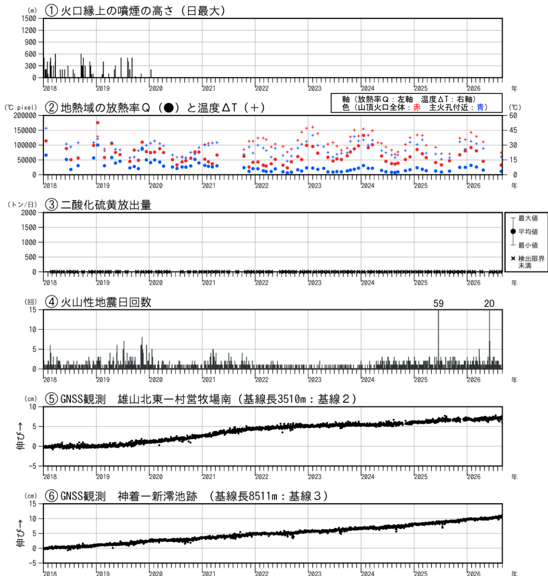
図4 三宅島 火山活動経過図（2018年1月1日～2026年8月31日）
