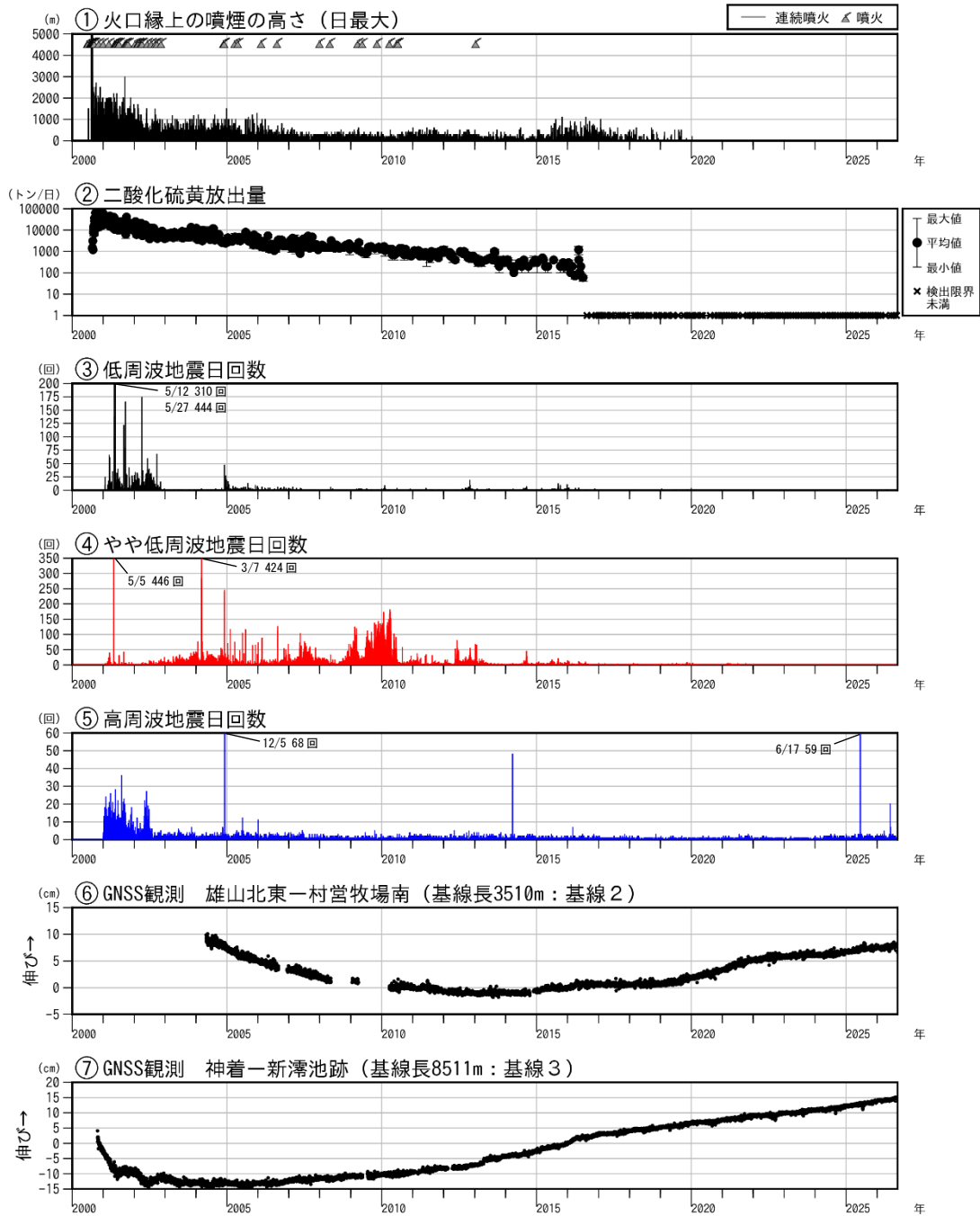
図5 三宅島 長期の火山活動経過図（2000年1月1日～2026年8月31日）
