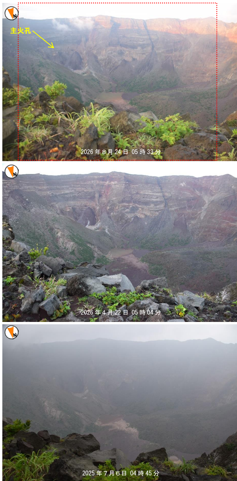
図3－① 三宅島 山頂火口内の状況（スオウ穴から撮影）
