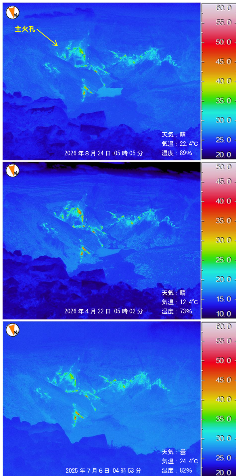
図3-② 三宅島 山頂火口内の地熱域の状況（スオウ穴から撮影）
