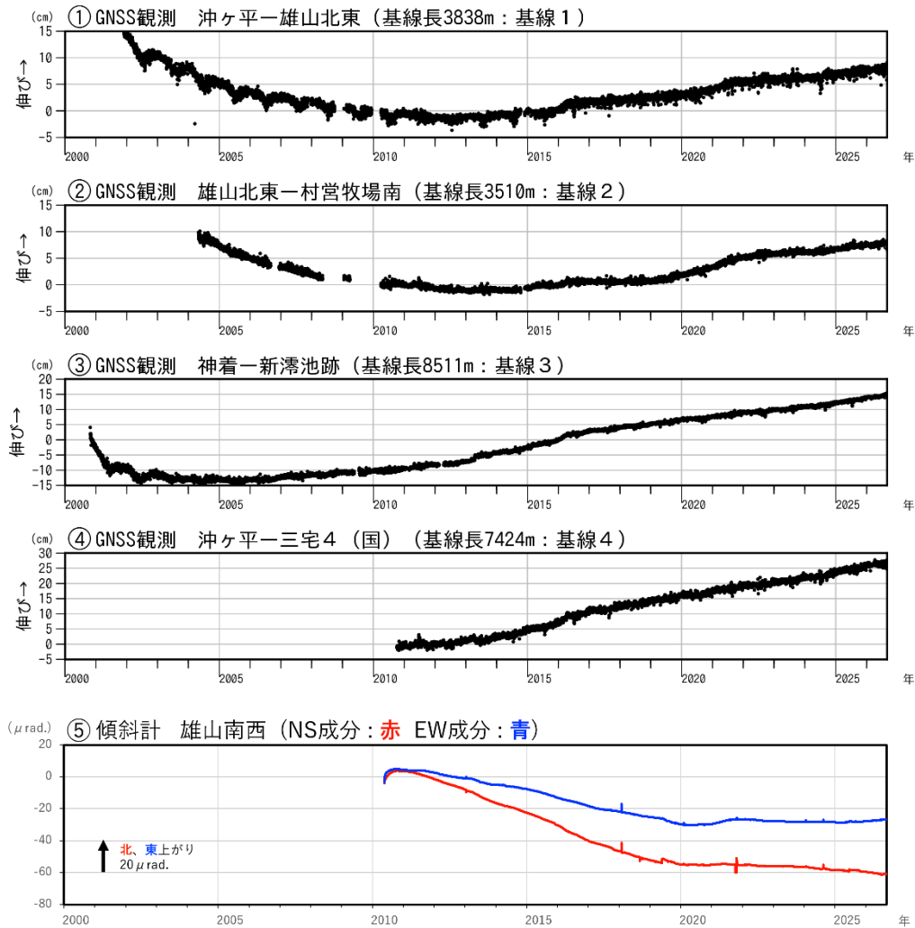
図6 三宅島 GNSS 連続観測及び傾斜計観測結果（2000年1月1日～2026年8月31日）
