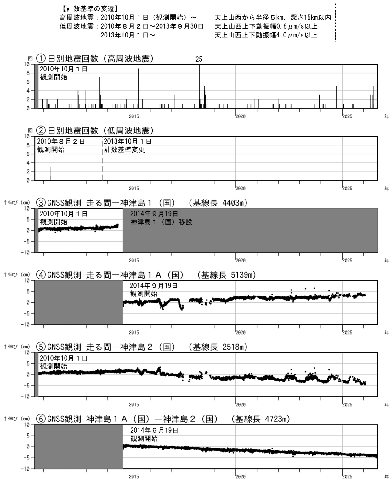
図2 神津島 火山活動経過図(2010年8月2日～2026年8月31日)
