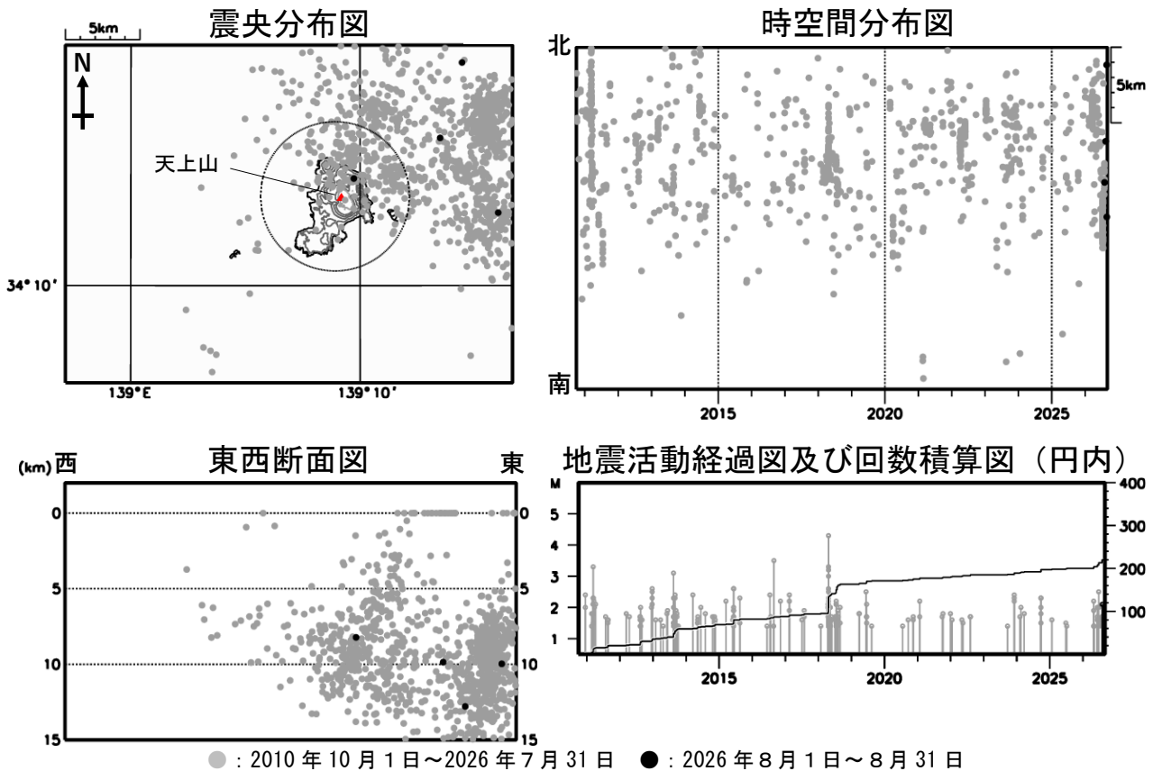
図3 神津島 広域地震観測網による山体・周辺の地震活動（2010年10月1日～2026年8月31日） 広域地震観測網により震源決定したもので、深さは全て海面以下として決定しています。なお、2020年9月以降については、地震観測点の標高を考慮する等、震源決定の手法を変更しています。 M（マグニチュード）は地震の規模を表し、M1.4以上の地震を示しています。 図中の震源要素は一部暫定値が含まれており、後日変更することがあります。 計数対象（天上山西から半径約5km、深さ約15km以内）以外の地震が含まれるため、図2-①の日別地震回数（高周波地震）とは異なります。 震央分布図中の円は火山性地震の回数の計数対象（天上山西から半径5km、深さ15km以内）の範囲を示しています。 ・地震活動は低調に経過しました。 ・1日21時36分に新島・神津島近海で発生した地震（マグニチュード2.1）により、神津島村で震度1を観測しました。
