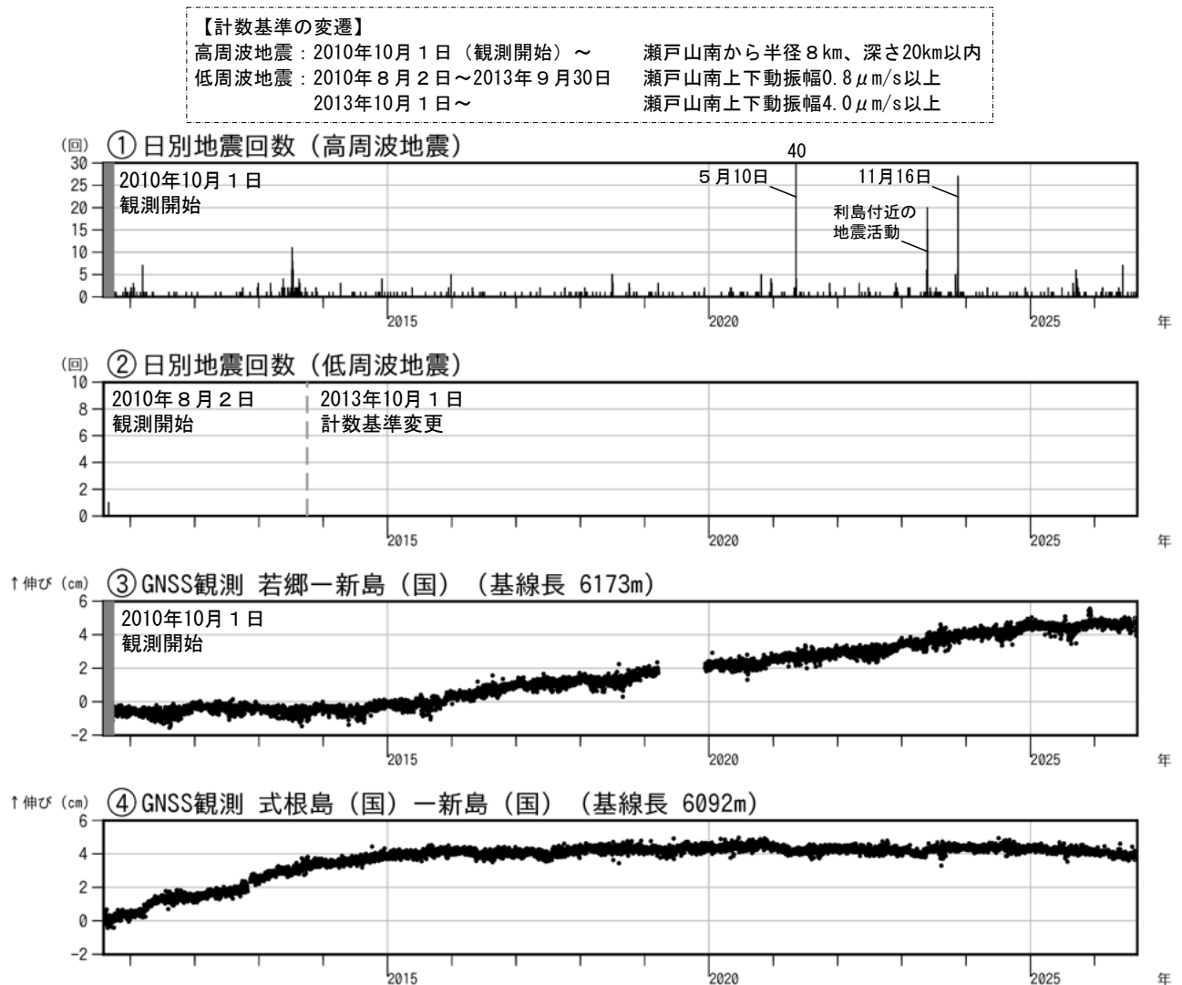
図2 新島 火山活動経過図(2010年8月2日～2026年8月31日)
