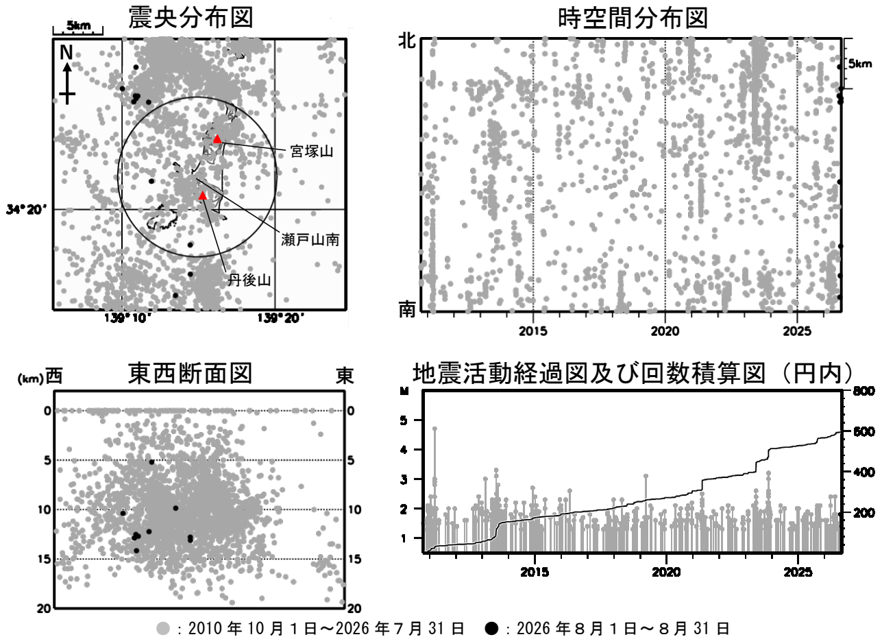
図3 新島 広域地震観測網による山体・周辺の地震活動（2010年10月1日～2026年8月31日） 広域地震観測網により震源決定したもので、深さは全て海面以下として決定しています。なお、2020年9月以降については、地震観測点の標高を考慮する等、震源決定の手法を変更しています。 M（マグニチュード）は地震の規模を表し、M1.3以上の地震を示しています。 図中の震源要素は一部暫定値が含まれており、後日変更することがあります。 計数対象（瀬戸山南から半径約8km、深さ約20km以内）以外の地震が含まれるため、図2-①の日別地震回数（高周波地震）とは異なります。 震央分布図中の円は火山性地震の回数の計数対象（瀬戸山南から半径8km、深さ20km以内）の範囲を示しています。 ・地震活動は低調に経過しました。
