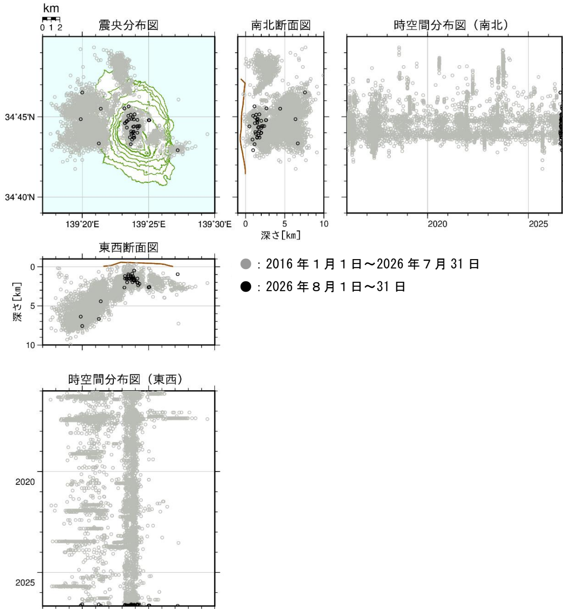
図4 伊豆大島 震源分布図（2016 年 1 月 1 日～2026 年 8 月 31 日）
