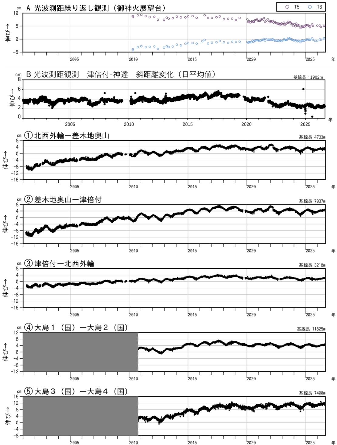
図3-1 伊豆大島 GNSS 連続観測及び光波測距観測による基線長変化(2001 年 1 月～2026 年 8 月)
