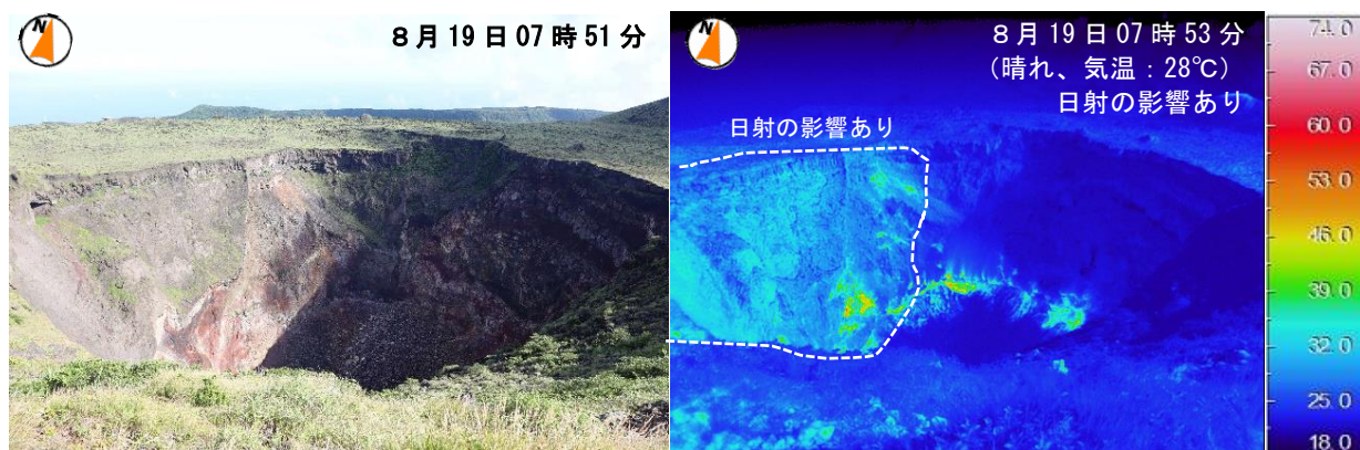
図6-1 伊豆大島 中央火孔内の状況（撮影方向は図6-3参照）
