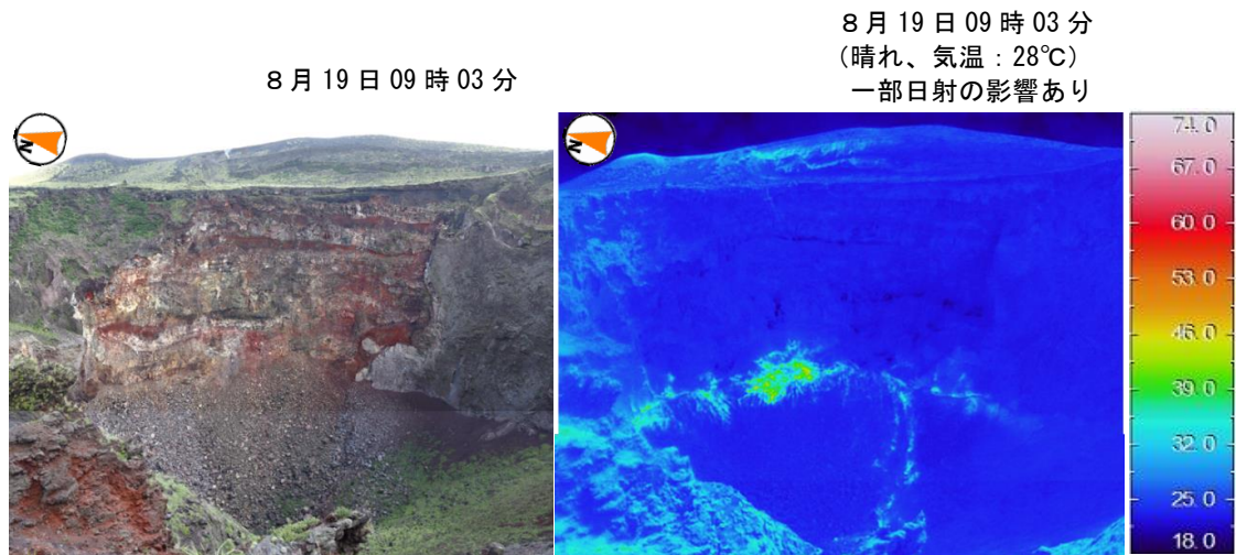
図6-2 伊豆大島 中央火孔内の状況（撮影方向は図6-3参照）
