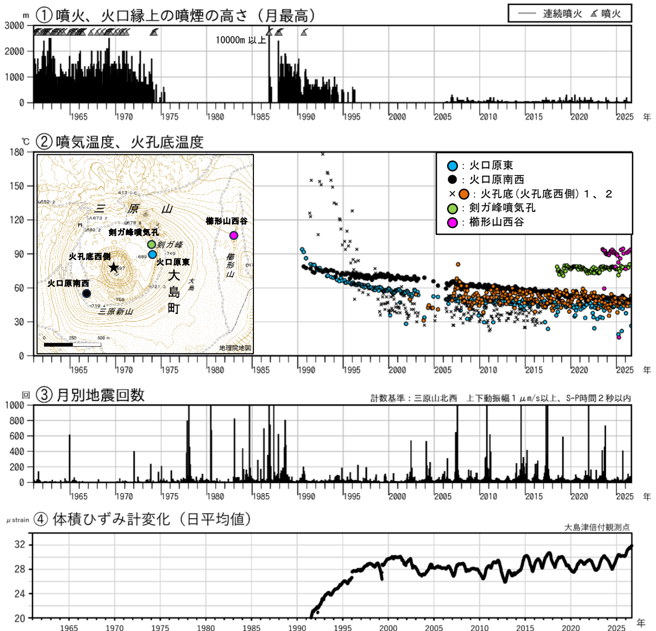
図1 伊豆大島 長期間の火山活動経過図（1961年1月～2026年8月）
