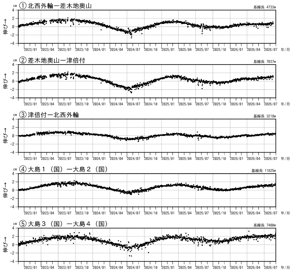
図3-2 伊豆大島 GNSS 連続観測による基線長変化(2022年12月～2026年8月)
