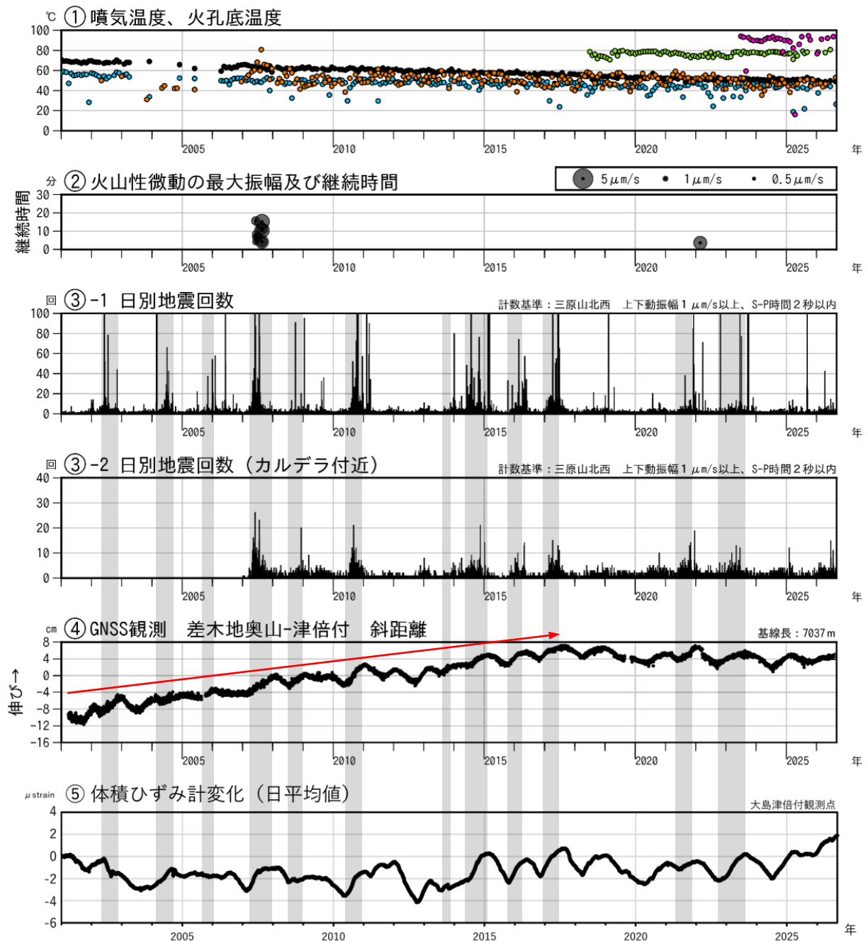
図2 伊豆大島 最近の火山活動経過図（2001年1月～2026年8月）
