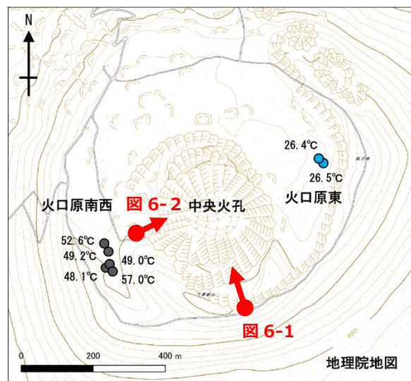
図6-3 伊豆大島 噴気温度の分布及び現地調査での撮影位置・撮影方向
