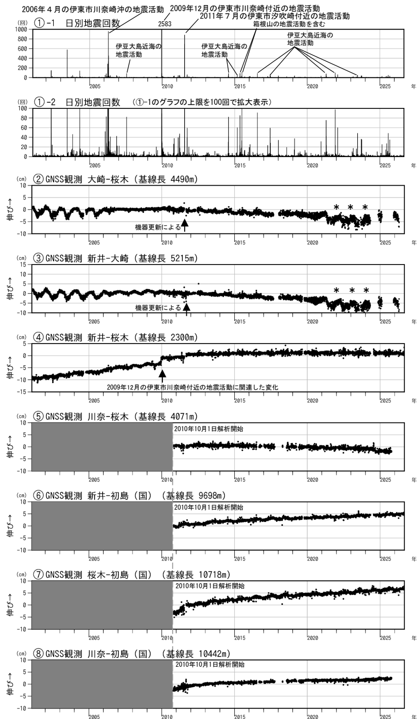
図3 伊豆東部火山群 火山活動経過図（2001年2月1日～2026年8月31日）
