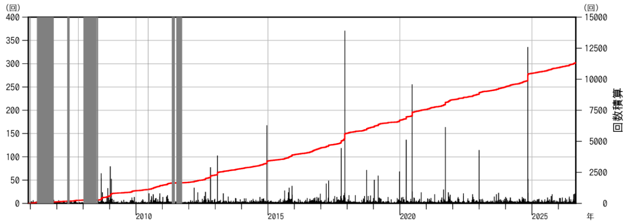
図3 白山 日別地震回数と積算回数（2005年12月1日～2026年8月31日） 図の灰色部分は機器障害による欠測期間。赤線は積算回数を示します。
