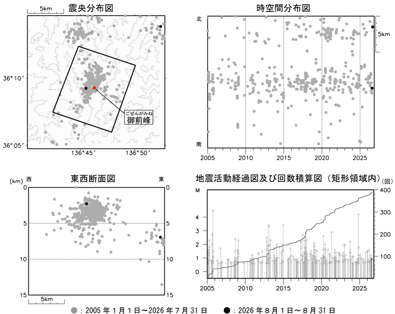
図4 白山 広域地震観測網による山体・周辺の地震活動（2005年1月1日～2026年8月31日） 広域地震観測網により震源決定したもので、深さは全て海面以下として決定しています。なお、2020年9月以降については、地震観測点の標高を考慮する等、震源決定の手法を変更しています。 M（マグニチュード）は地震の規模を表します。M0.6以上の地震を表示しています。 図中の震源要素は一部暫定値を含んでおり、後日変更することがあります。 ・今期間、白山付近の地震活動は低調に経過しました。
