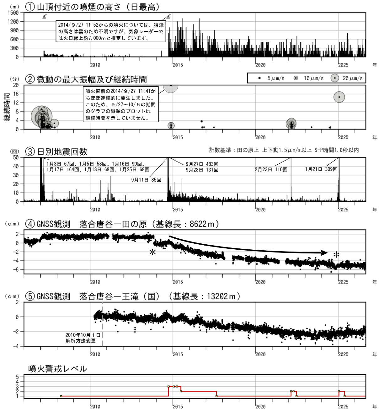
図1 御嶽山 長期間の火山活動経過図（2006年1月1日～2026年8月31日）
