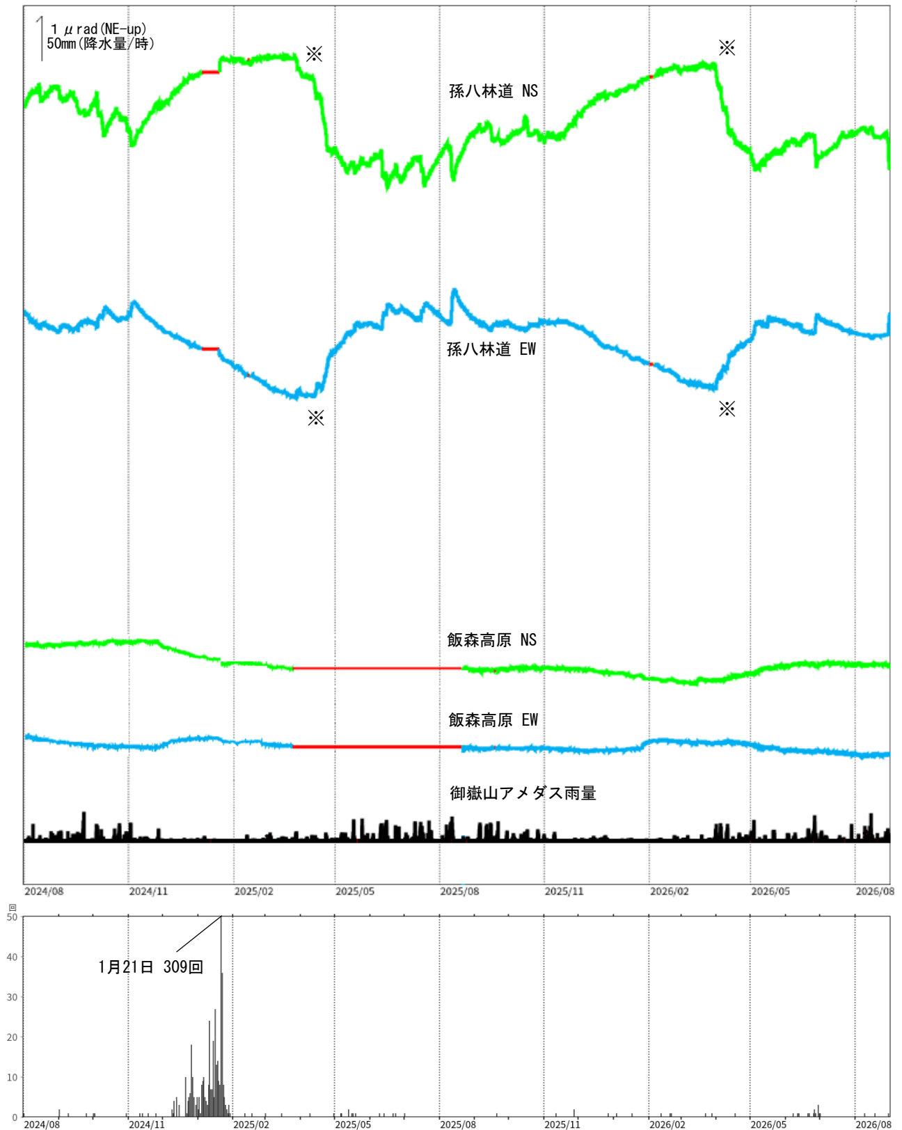
図7 御嶽山 傾斜変動と日別地震回数の推移（2024年8月1日～2026年8月31日）
