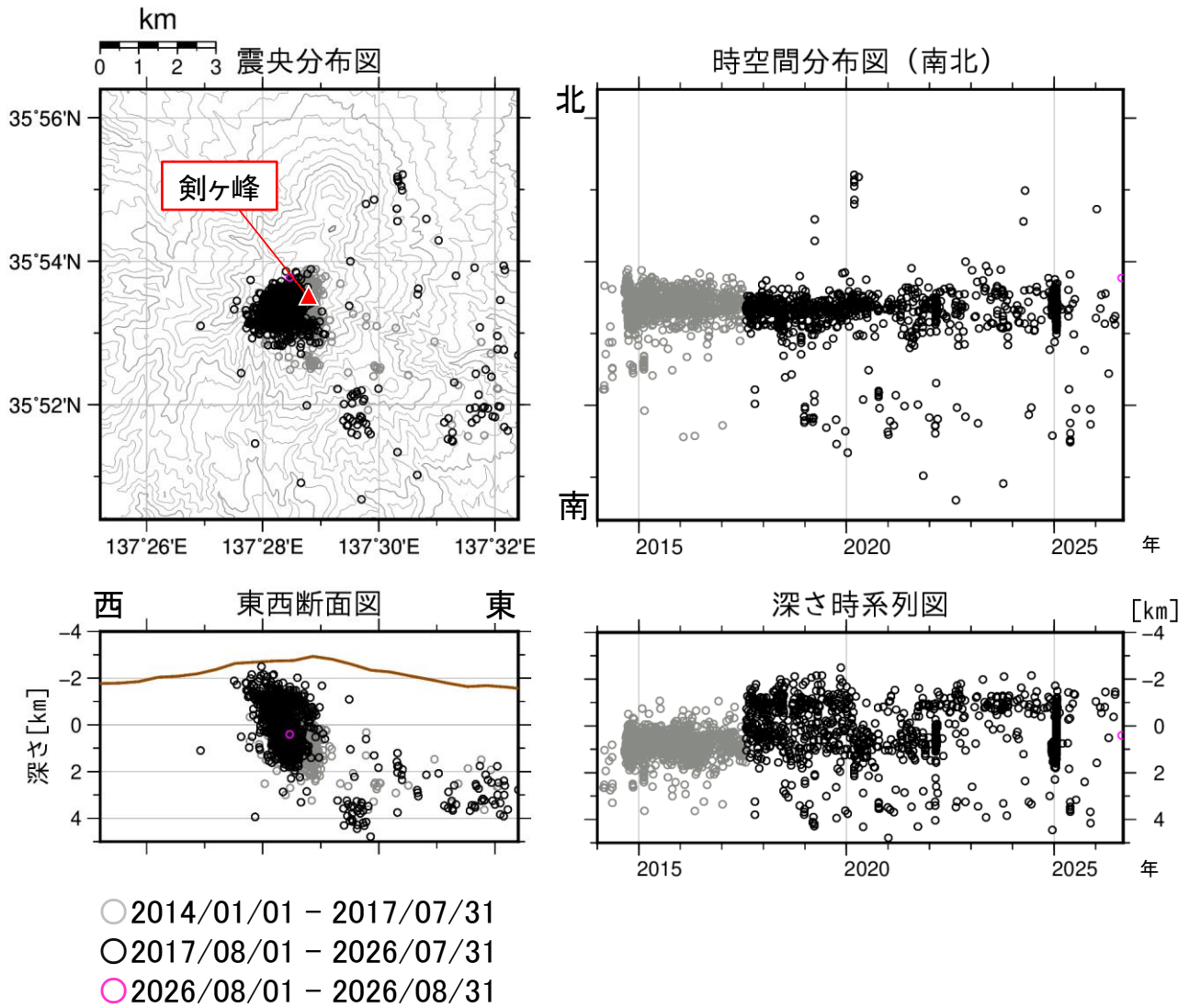
図4 御嶽山 震源分布図（2014年1月1日～2026年8月31日） 2017年8月1日以降の震源分布は、震源計算に使用する観測点を新たに追加して再計算したものを示しています。 観測点の移動状況により、求まる震源の数の減少や位置の精度低下が生じる場合があります。
