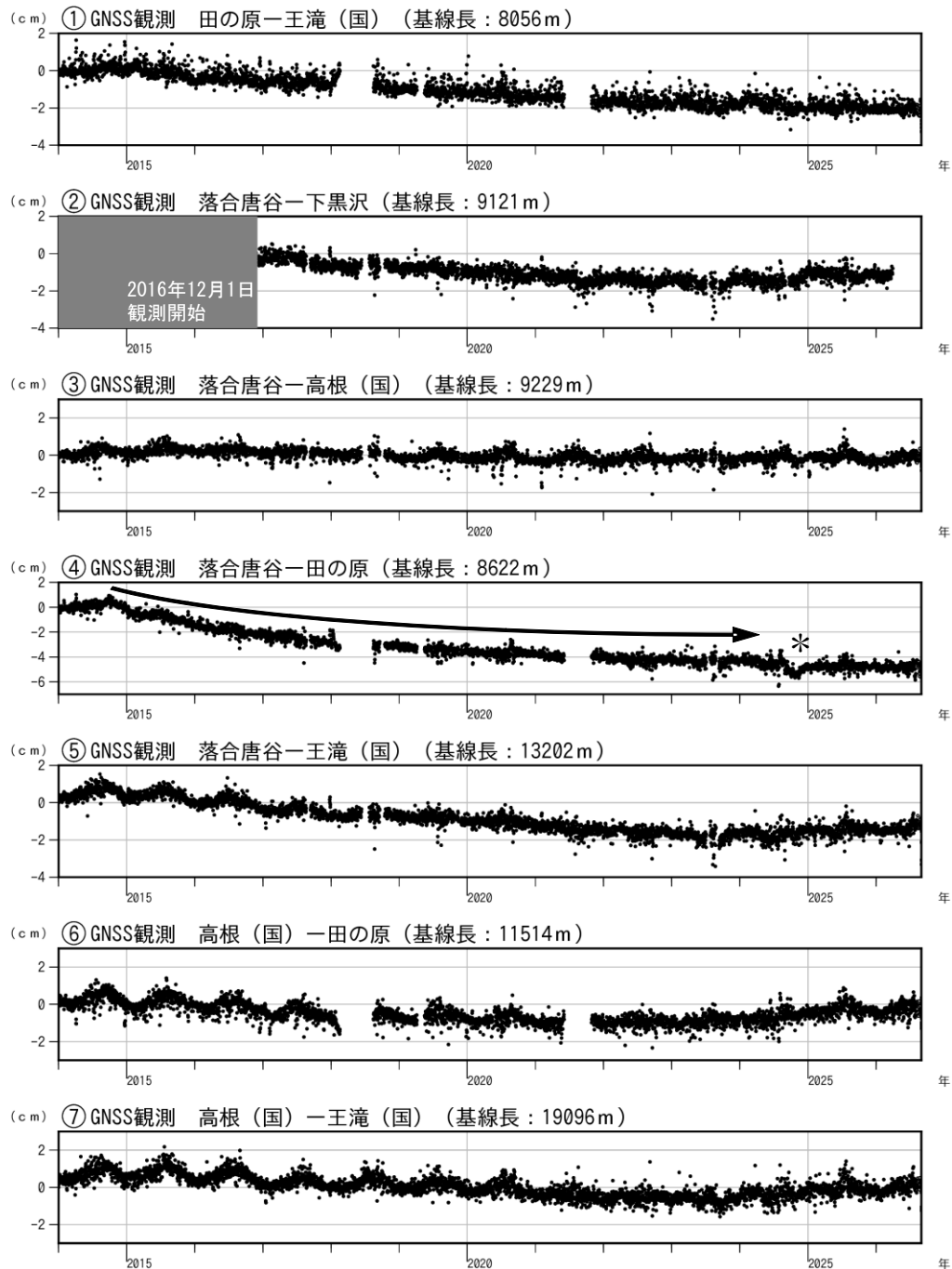
図5 御嶽山 GNSS 連続観測結果（2014年1月1日～2026年8月31日）
