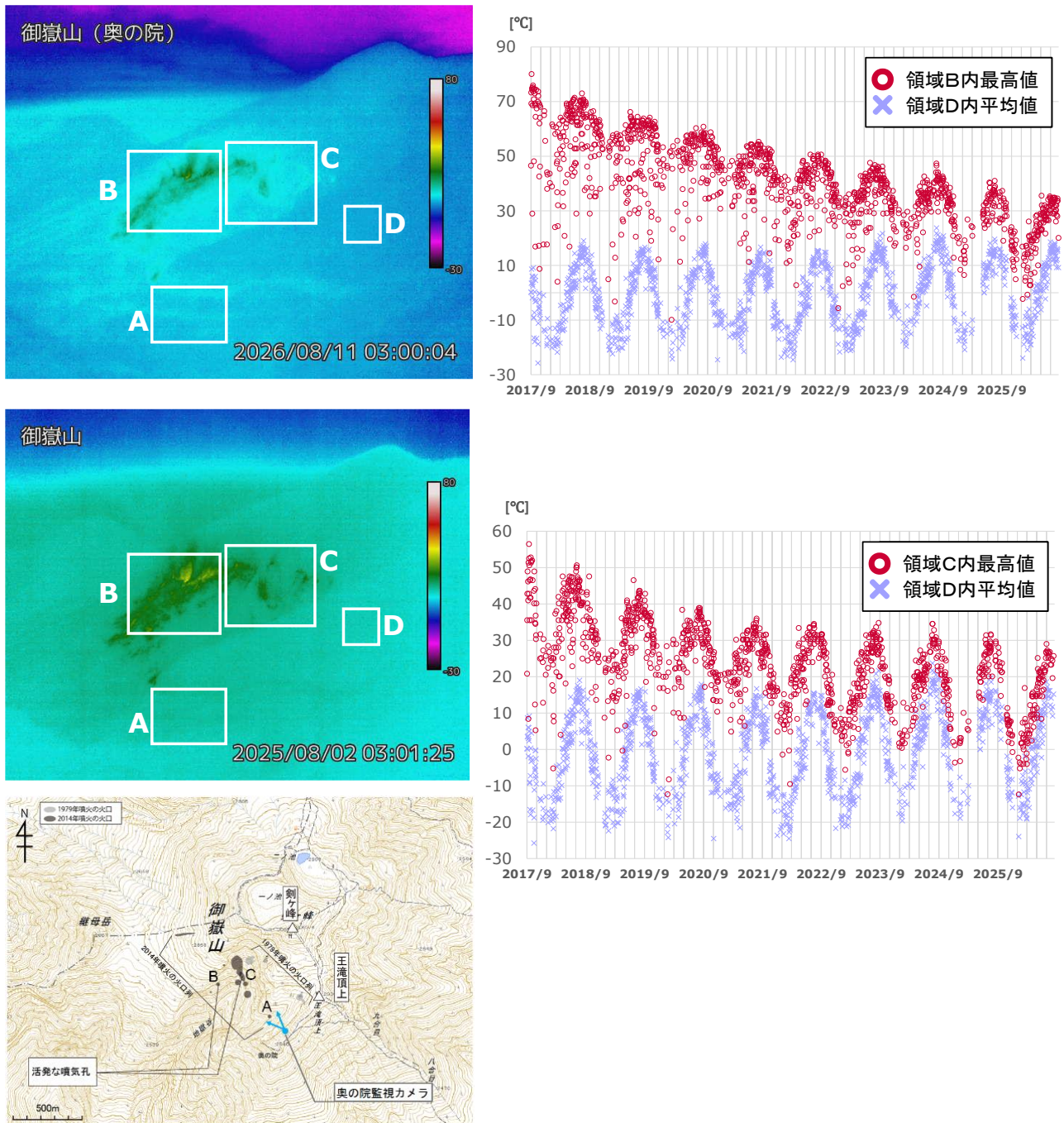
図3 御嶽山 奥の院赤外熱映像カメラによる地獄谷火口における最高温度の推移 (2017年9月13日～2026年8月31日)
