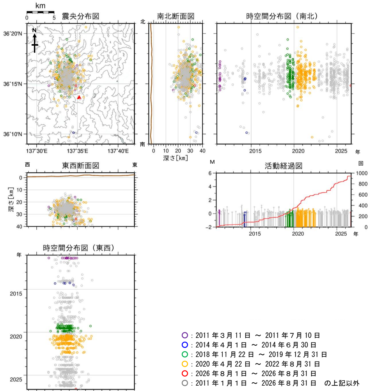
図10 焼岳 広域地震観測網による深部低周波地震の震源分布図（2011年1月1日～2026年8月31日）
