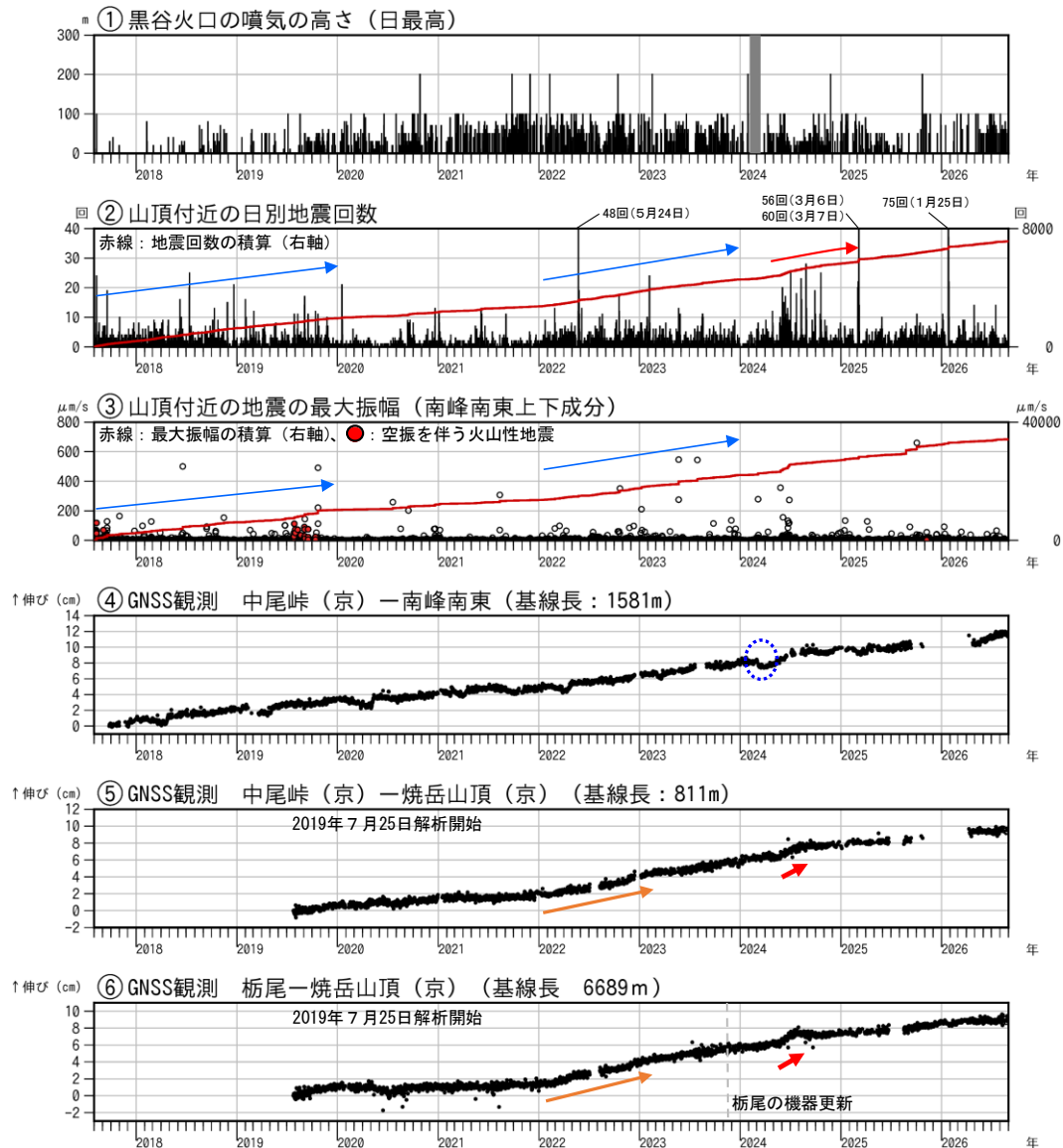
図1 焼岳 火山活動経過図（2017年8月1日～2026年8月31日）
