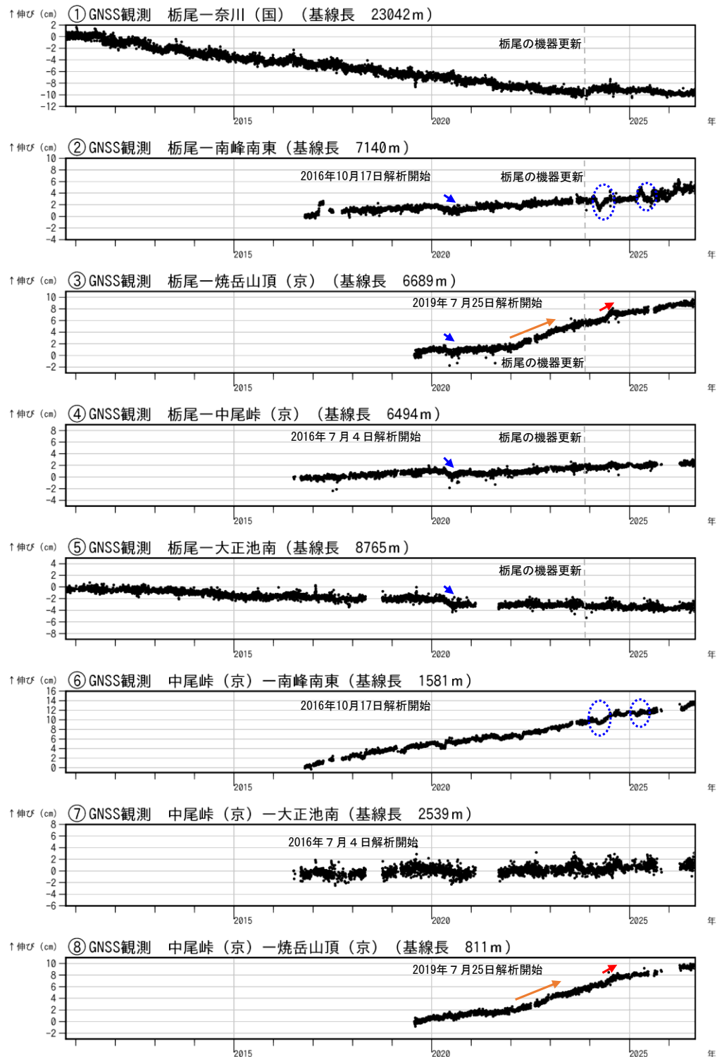
図6 焼岳 GNSS 連続観測による基線長変化（2010年10月1日～2026年8月31日）
