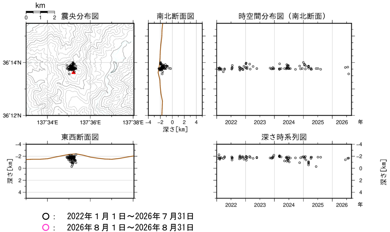
図2 焼岳 山頂付近の地震の震源分布図（2022年1月1日～2026年8月31日）
