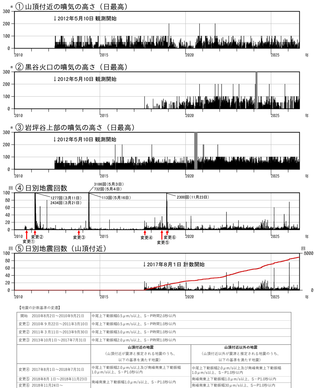
図5 焼岳 噴気の高さと地震回数の推移(2010年8月2日～2026年8月31日)
