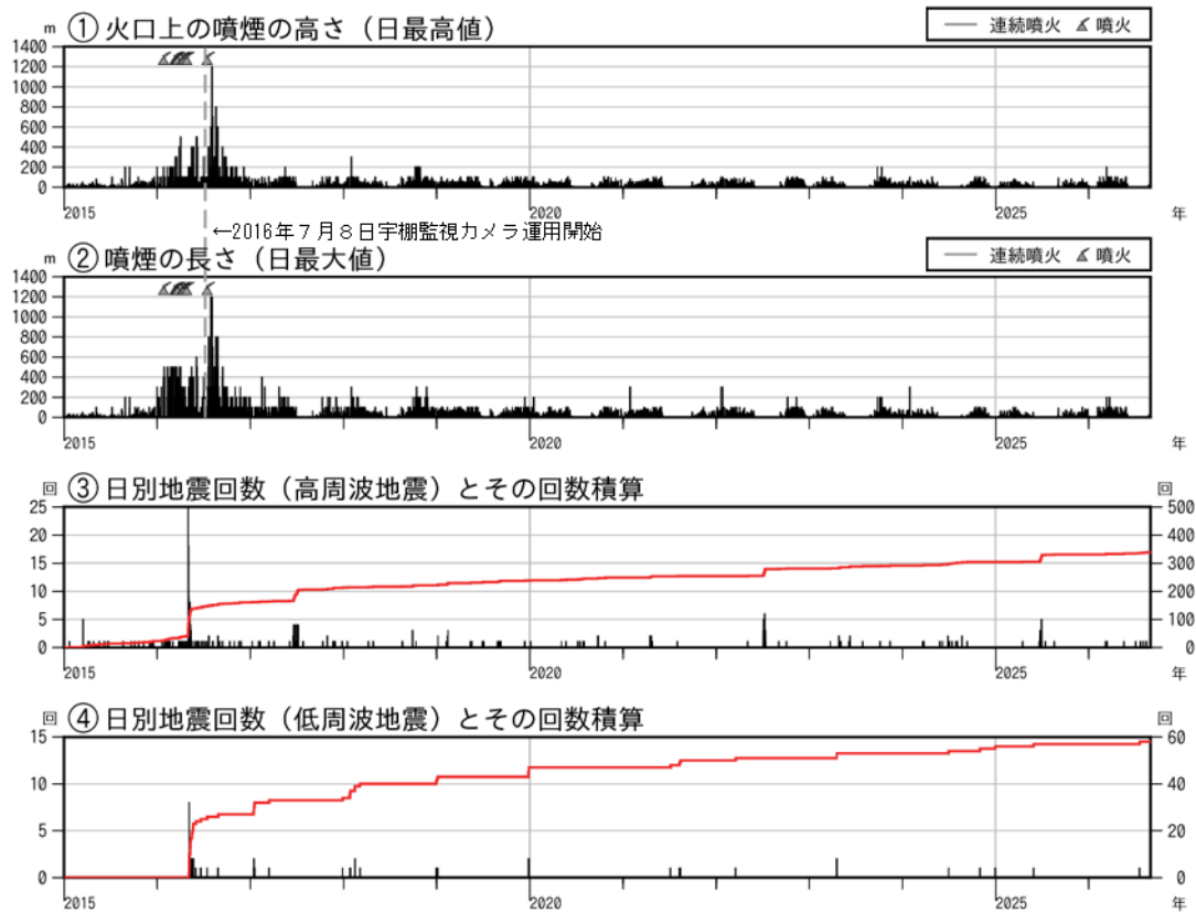
図3 新潟焼山 火山活動経過図（短期）（2015年1月1日～2026年8月31日）
