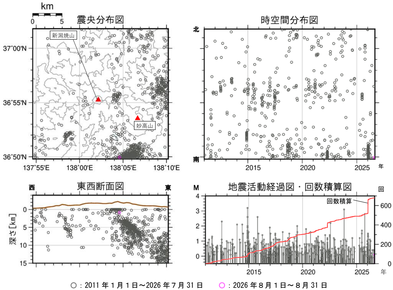
図4 新潟焼山 広域地震観測網による山体・周辺の地震活動（2011 年 1 月 1 日～2026 年 8 月 31 日） 広域地震観測網により震源決定したもので、深さは全て海面以下として決定しています。なお、2020 年 9 月以降については、地震観測点の標高を考慮する等、震源決定の手法を変更しています。 図中の震源要素は一部暫定値が含まれており、後日変更することがあります。
