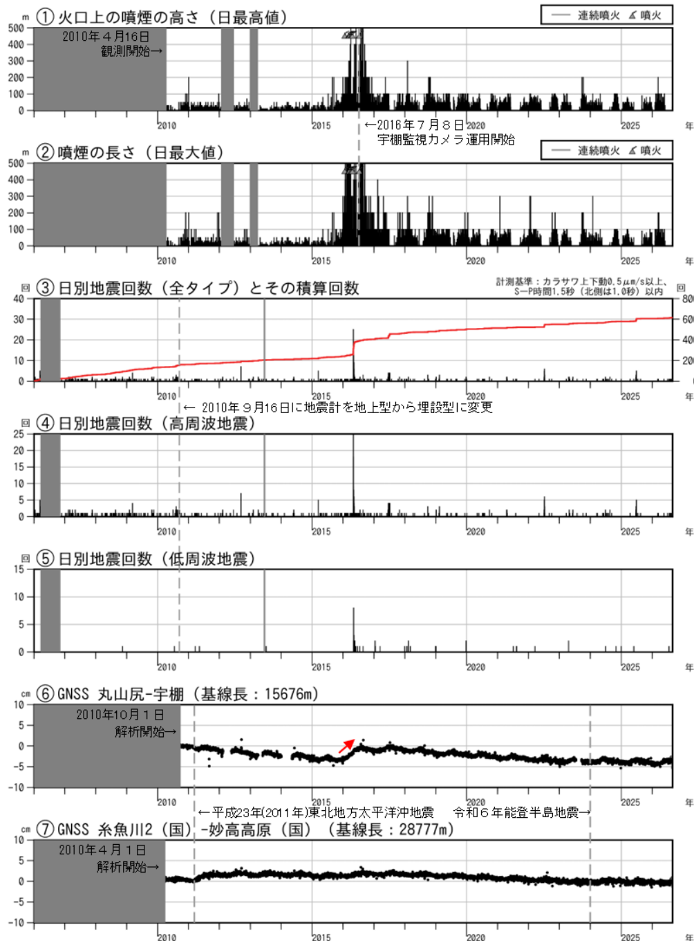
図2 新潟焼山 火山活動経過図（2006年1月1日～2026年8月31日）
