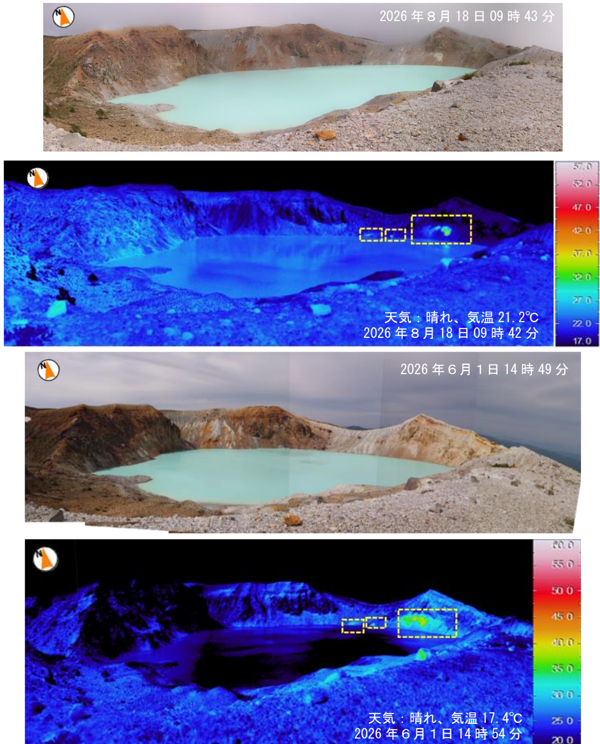
図1－3 草津白根山（白根山（湯釜付近））湯釜火口内の状況
