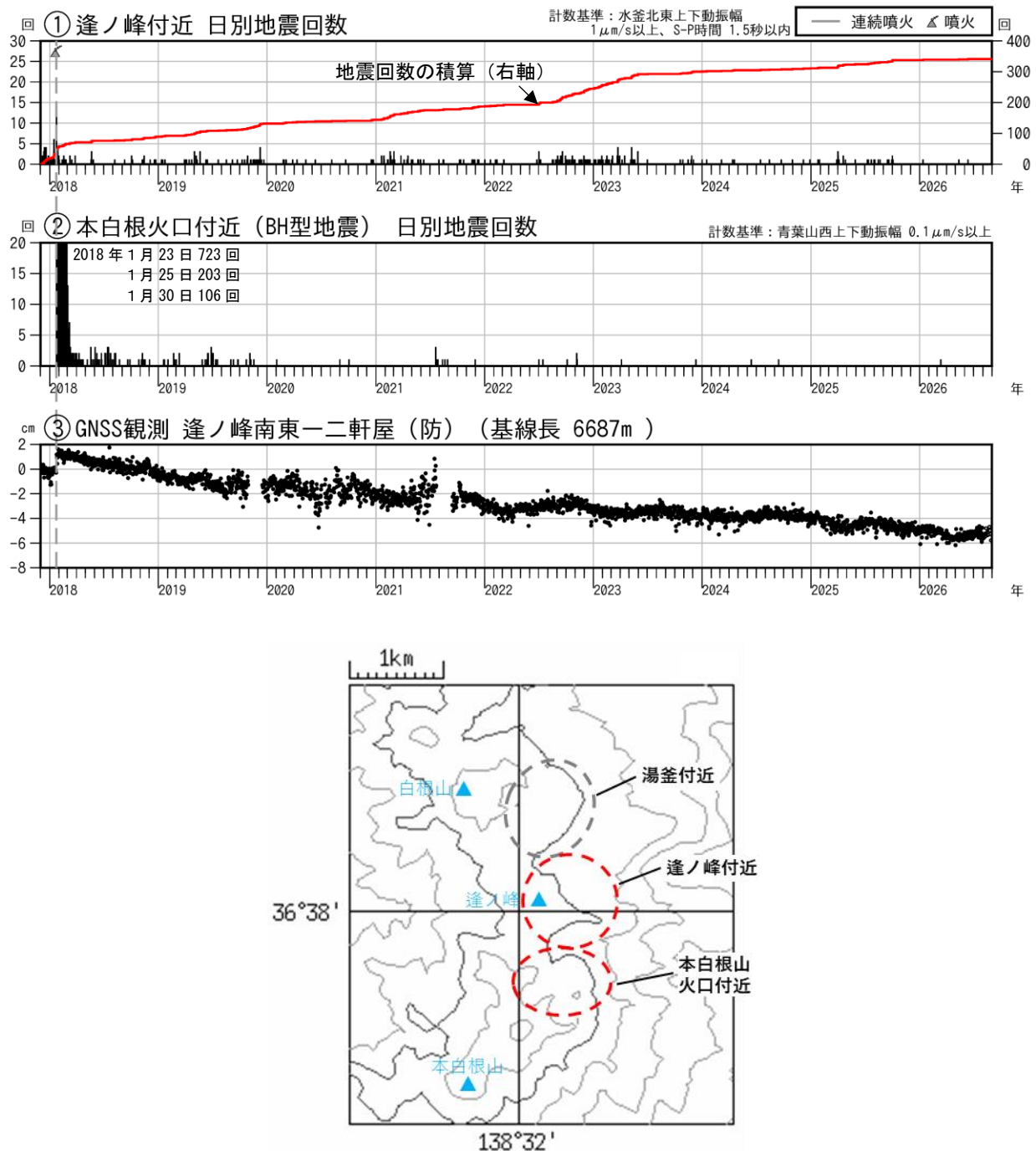
図 13 草津白根山（本白根山） 火山活動経過図（2017 年 12 月 1 日～2026 年 8 月 31 日）
