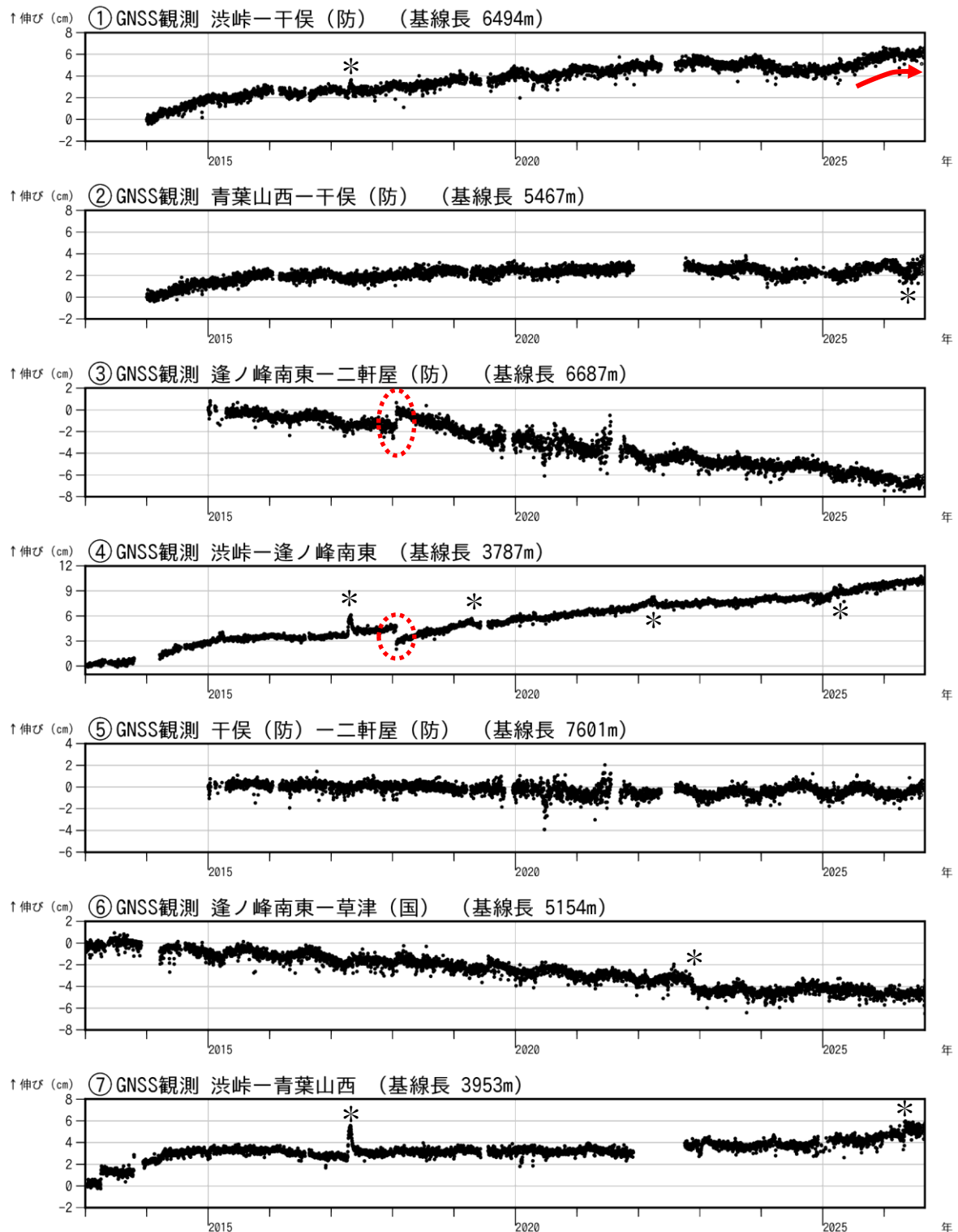
図6 草津白根山 GNSS 連続観測結果（2013年1月1日～2026年8月31日）
