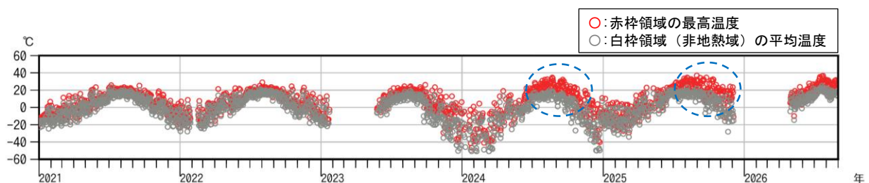
図1-4 草津白根山（白根山（湯釜付近）） 水釜北東の地熱域の状況
