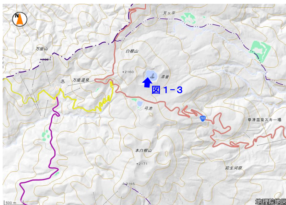
図1-2 草津白根山（白根山（湯釜付近） 観測位置及び撮影方向
