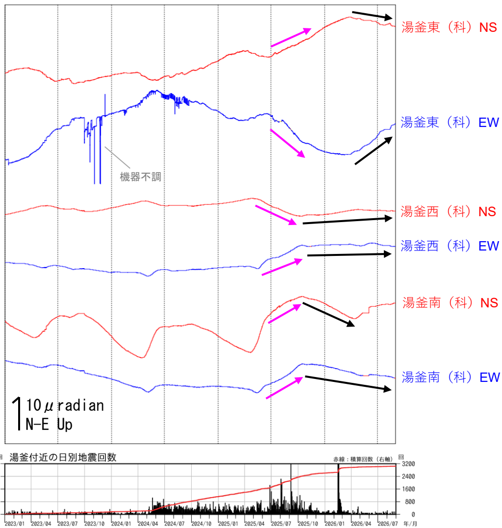
図5 草津白根山（白根山（湯釜付近）） 傾斜変動及び日別地震回数 (2023年1月1日～2026年8月31日)
