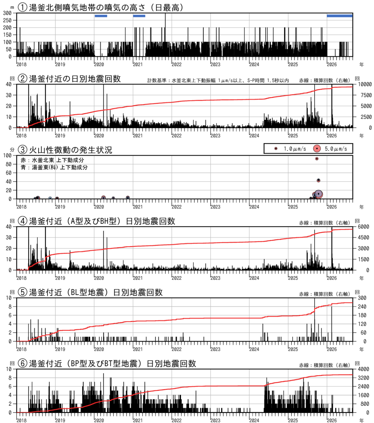
図3 草津白根山（白根山（湯釜付近）） 火山活動経過図（2018年1月1日～2026年8月31日）
