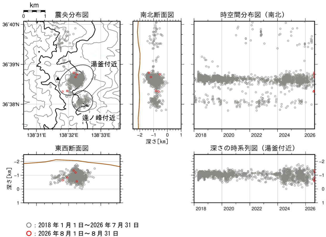
図4 草津白根山 震源分布図（2018年1月1日～2026年8月31日）
