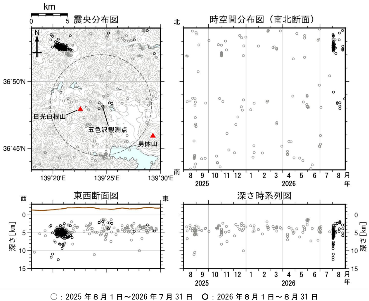
図3 日光白根山 広域地震観測網による山体周辺の地震活動 (2025 年 8 月 1 日～2026 年 8 月 31 日)
