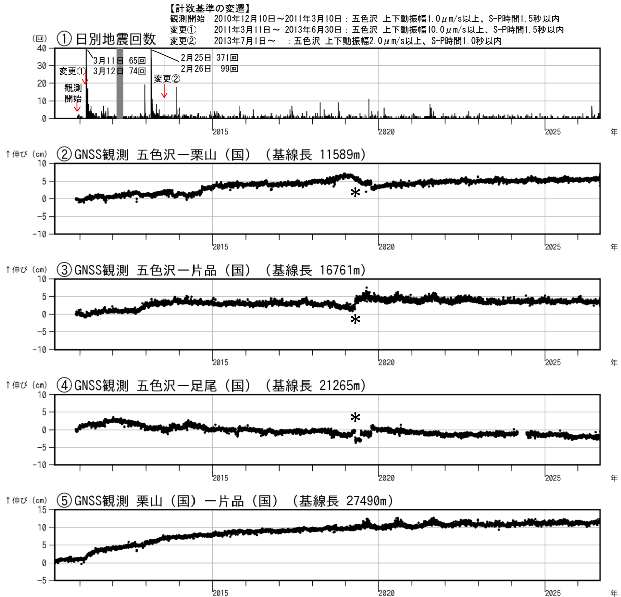
図2 日光白根山 火山活動経過図（2010年4月1日～2026年8月31日）
