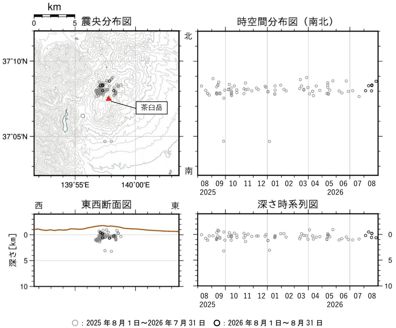
図5 那須岳 震源分布図（2025年8月1日～2026年8月31日）
