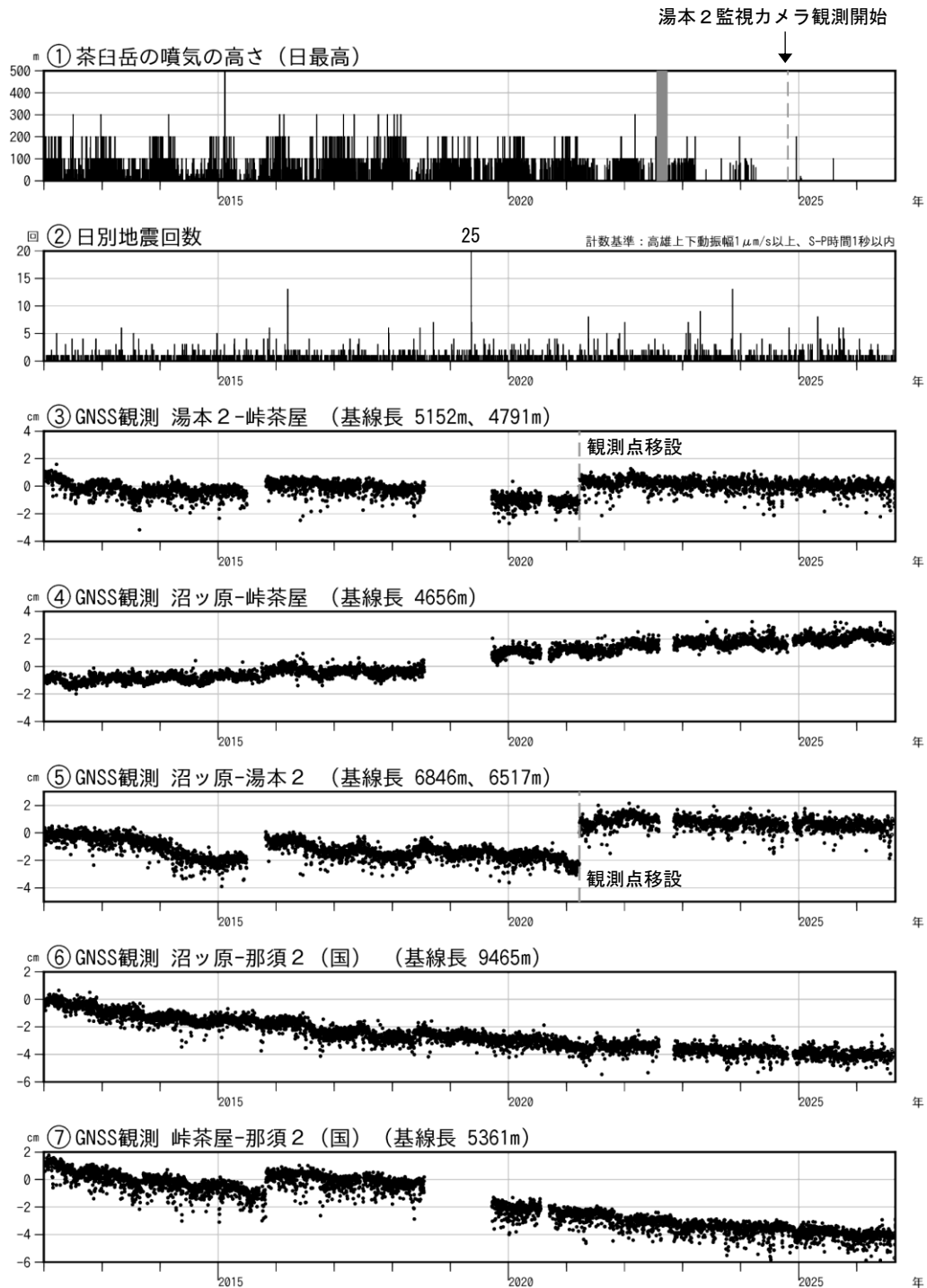
図4 那須岳 火山活動経過図（2012年1月1日～2026年8月31日）
