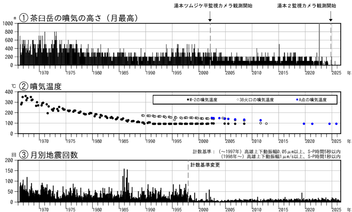
図3-1 那須岳 火山活動経過図 (1966年6月～2026年8月)
