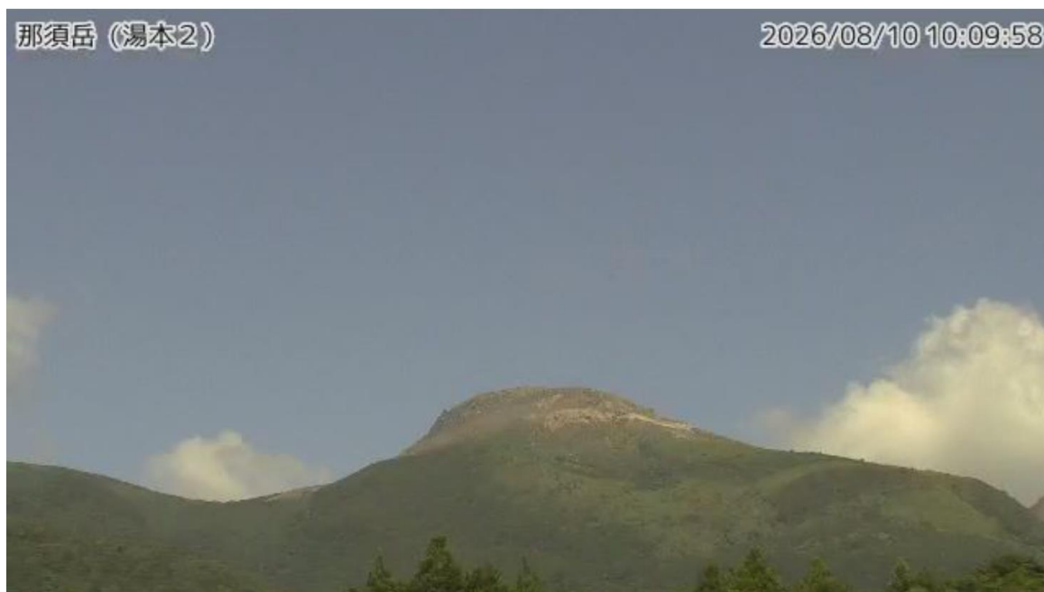
図1 那須岳 茶臼岳の状況（8月10日、湯本2監視カメラによる）
